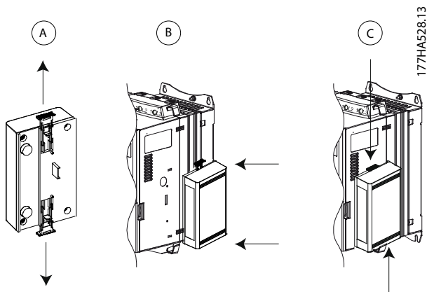
Abbildung 3.1 Installieren der EtherNet/IP-Option
