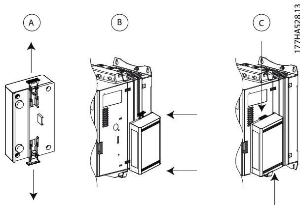
Disegno 3.1 Installazione dell'opzione EtherNet/IP
