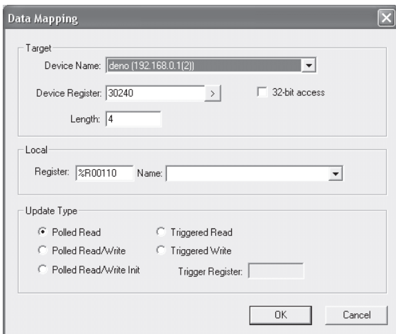
Illustration 7.3 Obtenir état (démarrage à l'adresse 30240)
