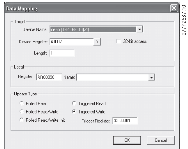
Illustration 7.6 Envoyer ordre de démarrage (registre 40002)
