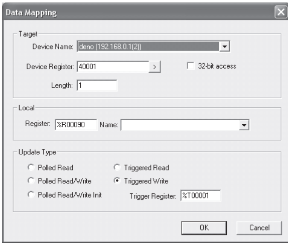
Illustration 7.2 Envoyer ordre de démarrage (registre 40001)
