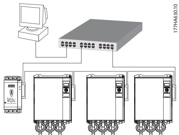
Abbildung 8.3 Ring-Netzwerktopologie
