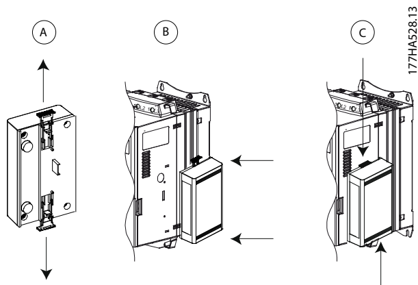
Disegno 3.1 Installazione dell'opzione EtherNet/IP
