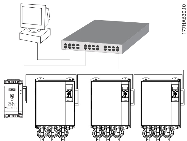
Disegno 8.3 Topologia di rete ad anello
