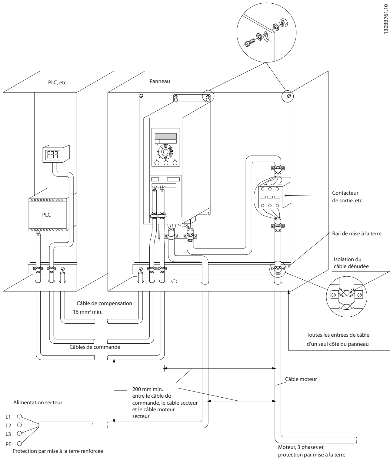
Illustration 1.20 Installation électrique conforme CEM
