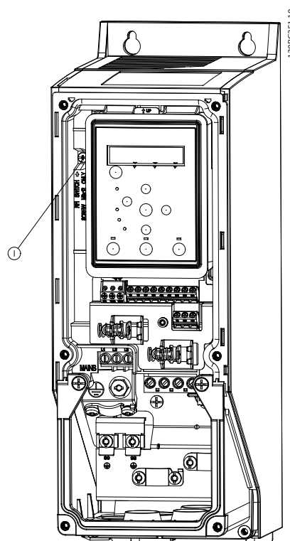
Illustration 1.2 IP54 400 V 0,75-18,5 kW 1: vis CEM
