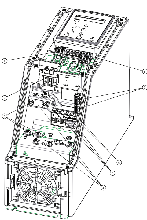
图 1.13 I2 机架 IP54 380-480 V 0.75-4.0 kW
