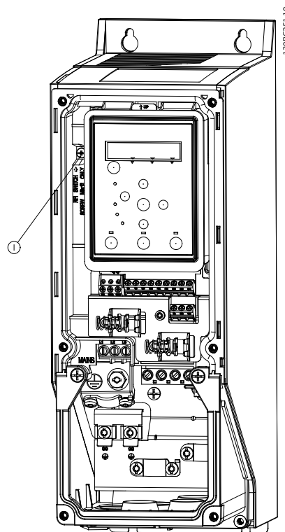
图 1.2 IP54 400 V 0.75-18.5 kW
