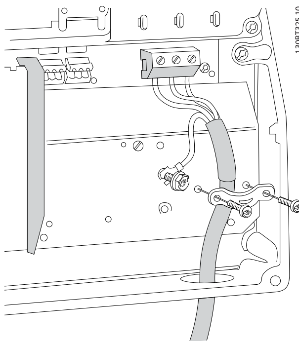
图 1.18 I6 机架 IP54 380-480 V 22-37 kW
