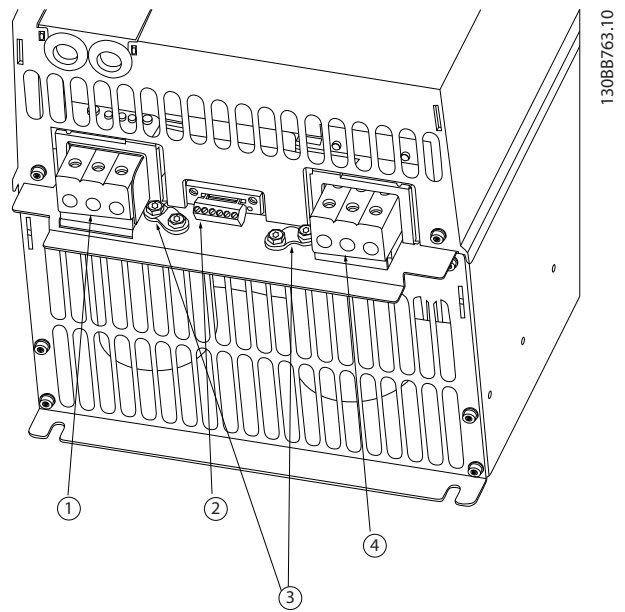
图 1.5 H7 机架
