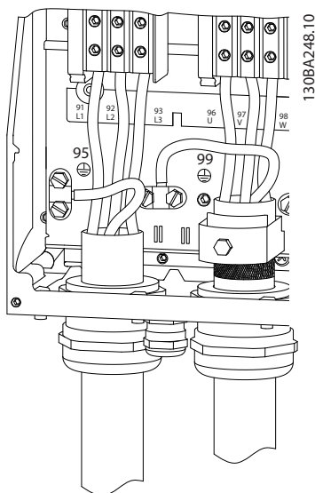
图 1.20 17、18 机架 IP54 380-480 V 45-55 kW IP54 380-480 V 75-90 kW
