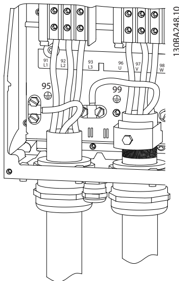
Illustration 3.20 I7- og I8-kapslinger IP54, 380-480 V, 45-55 kW (60-70 hk) IP54, 380-480 V, 75-90 kW (100-125 hk)
