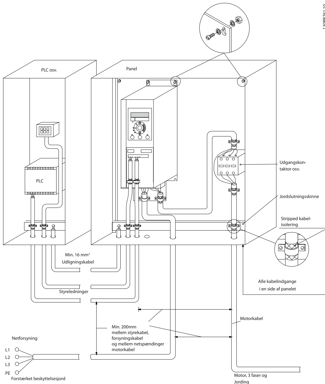
Illustration 3.21 EMC-korrekt elektrisk installation
