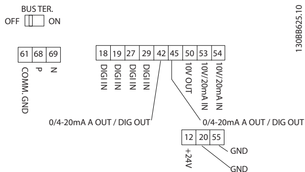
Illustration 3.23 Styreklemmer
