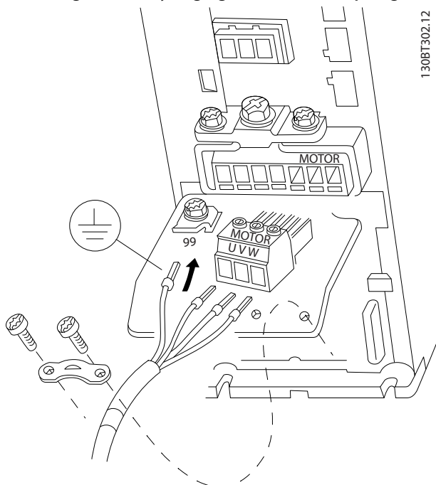
Illustration 3.7 Tilslutning af frekvensomformereren til motor, H9-kapsling
