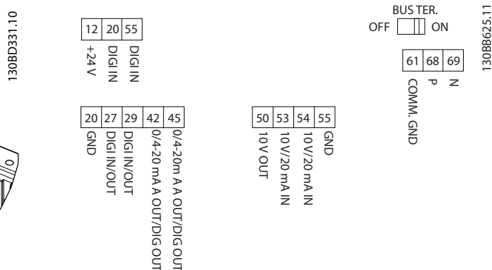
图 3.23 控制端子
