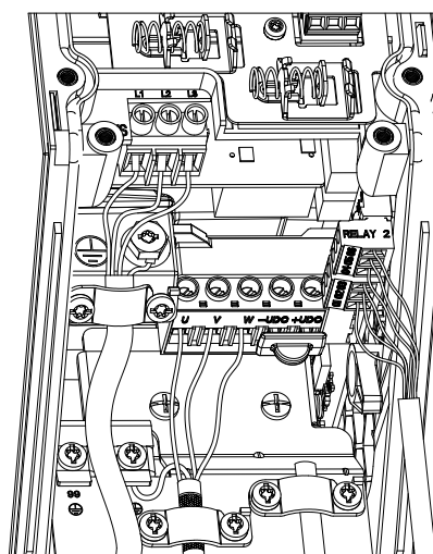
图 3.16 IP54 机箱规格 I2、I3、I4
