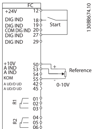
Illustration 4.2 Frekvensomformerens ledningsføring
