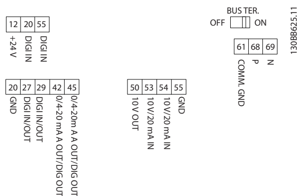
Ilustración 3.23 Terminales de control
