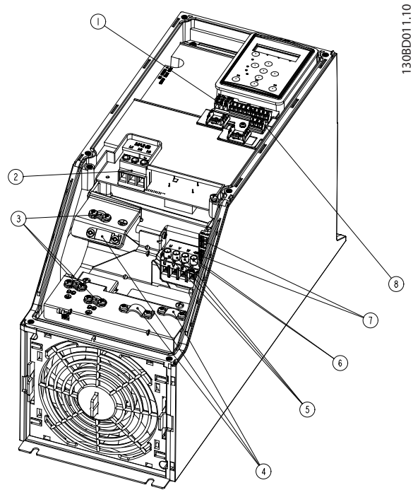
외함 용량 I4
