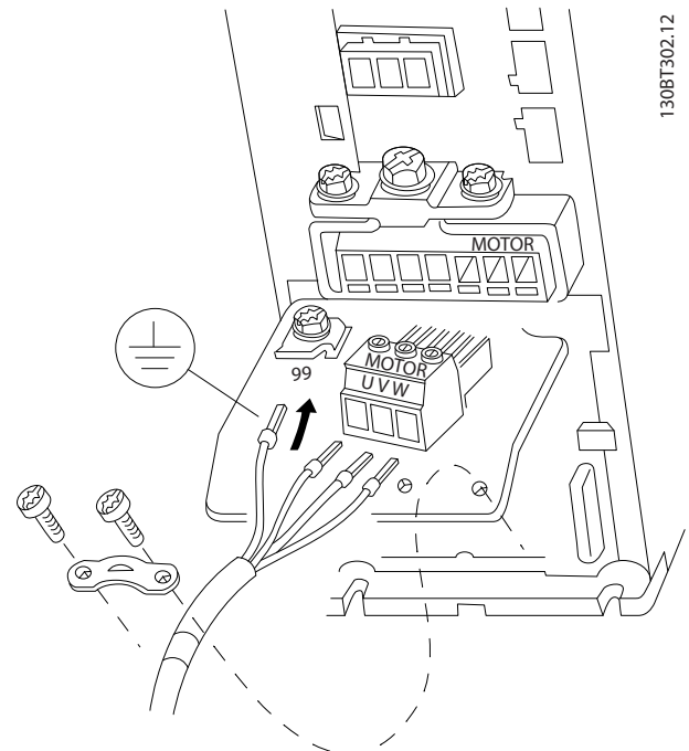
그림 3.7 모터에 주파수 변환기 연결, 외함 용량 H9 IP20, 600 V, 2.2-7.5 kW (3-10 hp)
