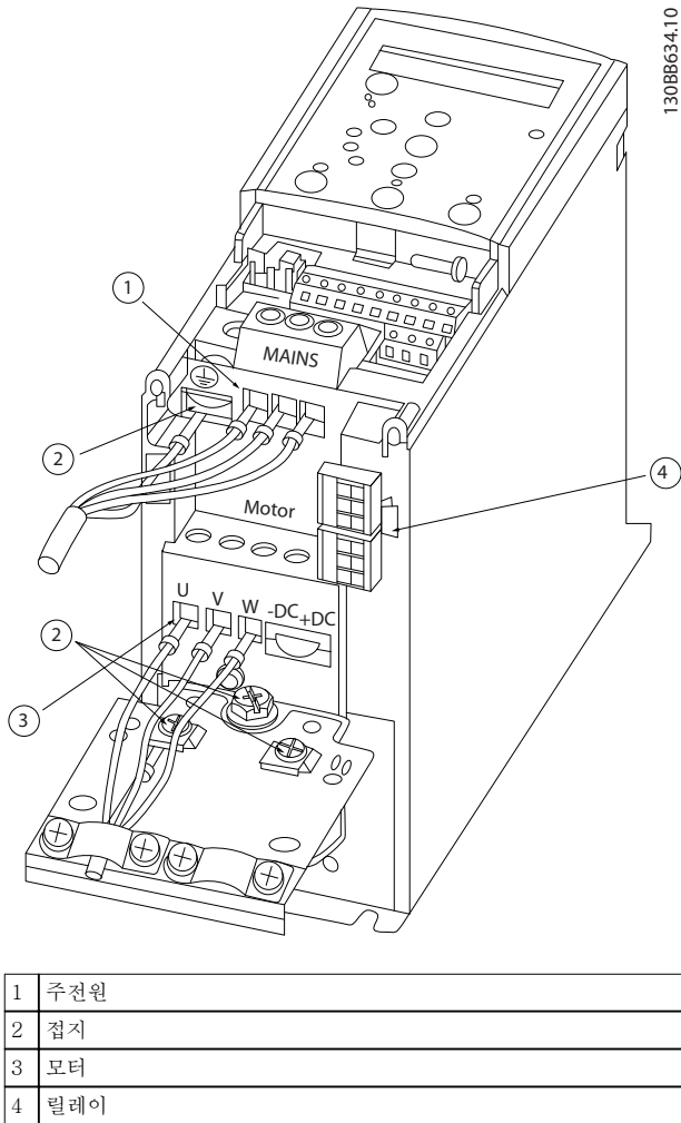
그림 3.3 외함 용량 H1-H5
