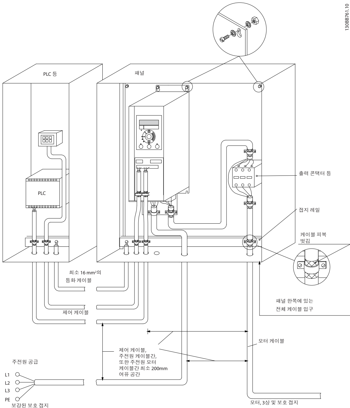
그림 3.21 EMC 규정에 따른 전기적인 설치
