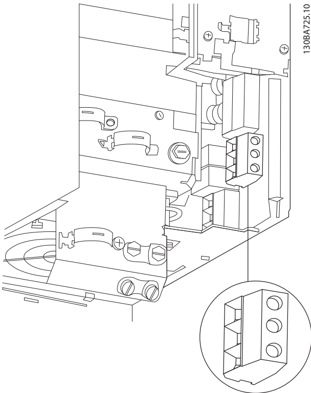
그림 3.12 외함 용량 H10 IP20, 600 V, 11-15 kW (15-20 hp)
