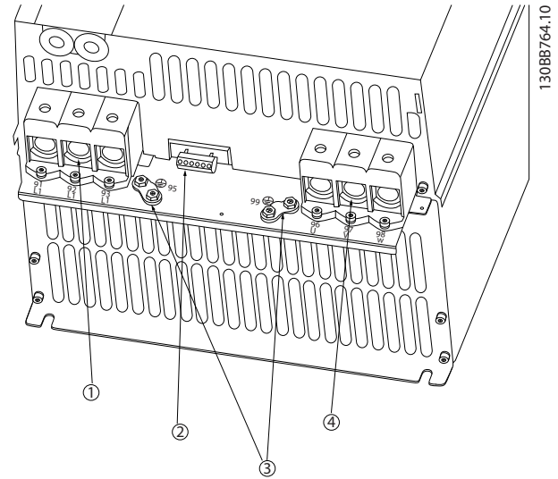
외함 용량 H8의 릴레이 및 단자
