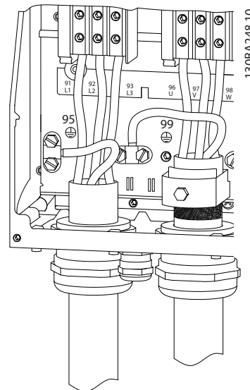
그림 3.20 외함 용량 I7, I8 IP54, 380-480 V, 45-55 kW (60-70 hp) IP54, 380-480 V, 75-90 kW (100-125 hp)
