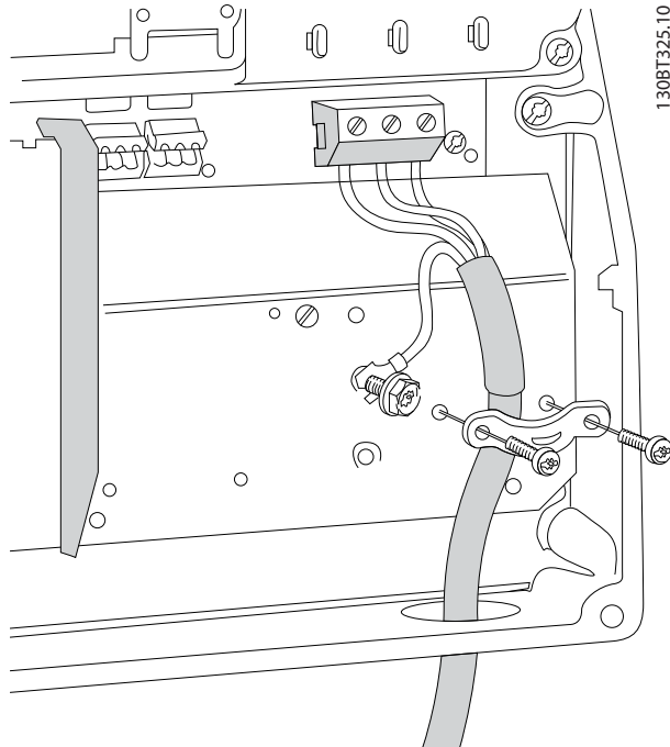
그림 3.18 모터에 연결(외함 용량 I6) IP54, 380-480 V, 22-37 kW (30-50 hp)
