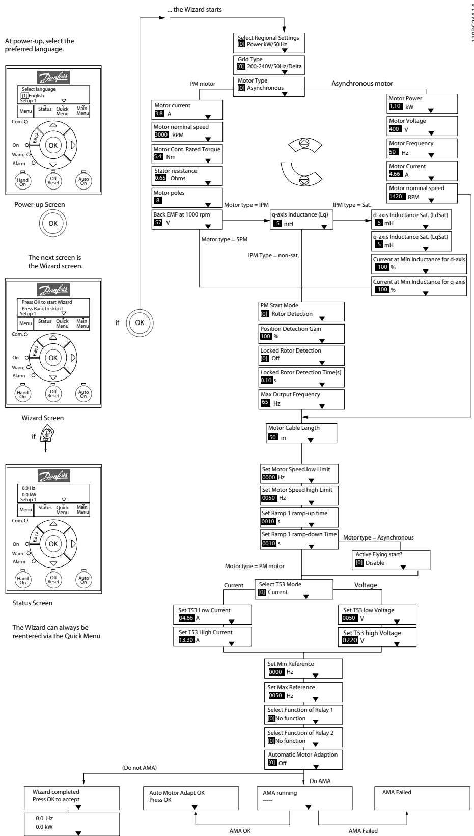
그림 4.4 개회로 어플리케이션용 셋업 마법사
