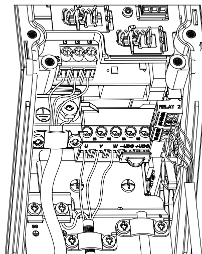
그림 3.16 IP54 외함 용량 I2, I3, I4
