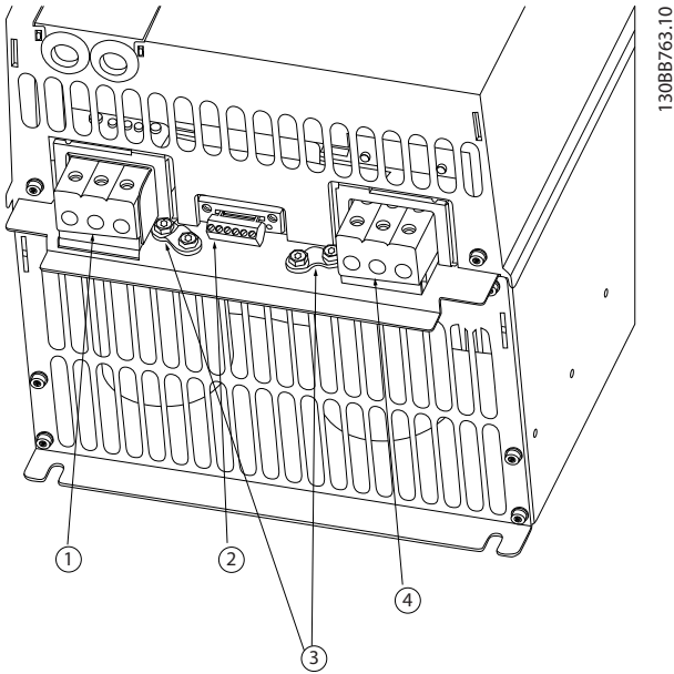
외함 용량 H7의 릴레이 및 단자
