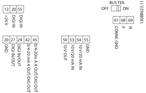
그림 3.23 제어 단자
