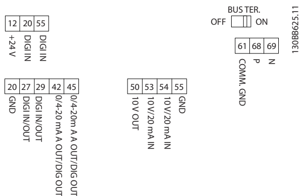
Ilustrasi 3.23 Terminal Kontrol
