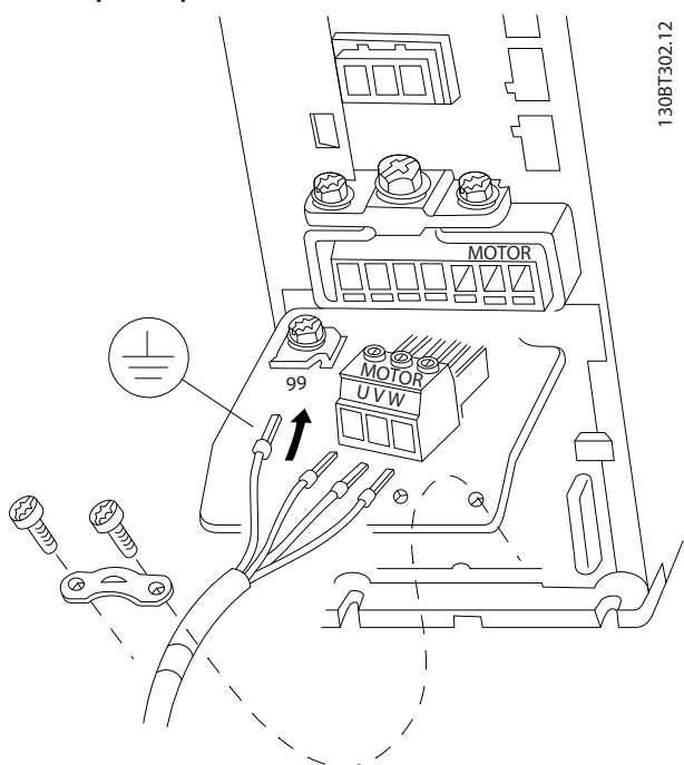
Ilustrasi 3.8 Pemasangan Pelat Dudukan
