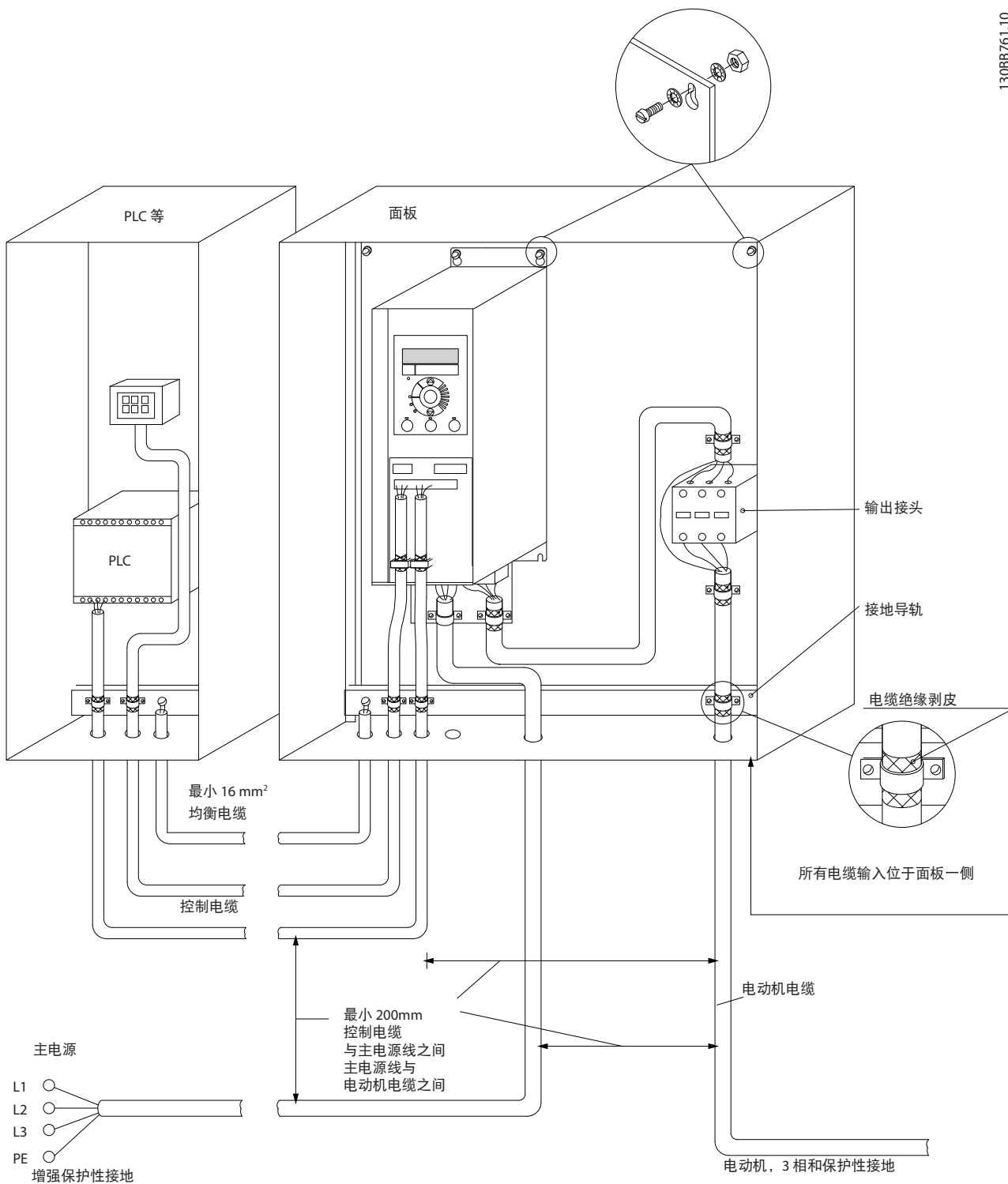
图 3.21 符合 EMC 规范的电气安装
