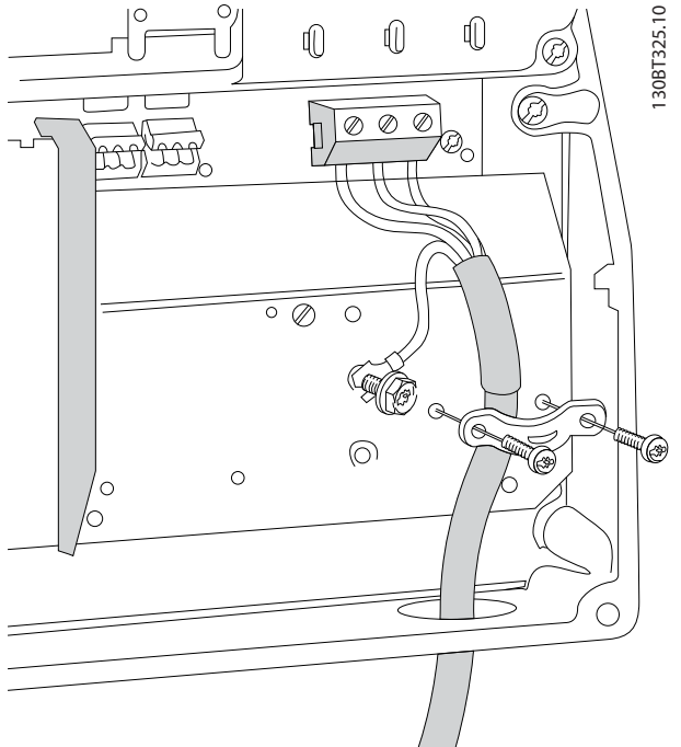
图 3.18 连接电机 — 16 机箱
