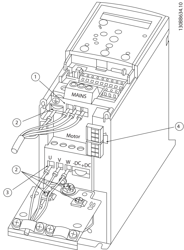
外殼規格 H1-H5 上的繼電器與端子
