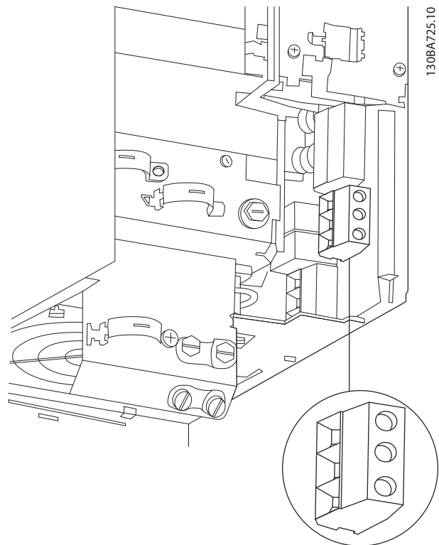
圖 3.12 外殼規格 H10 IP20, 600 V, 11 - 15 kW (15 - 20 hp)
