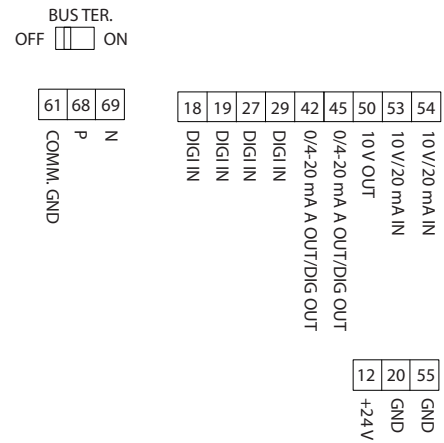
圖 3.23 控制端子
