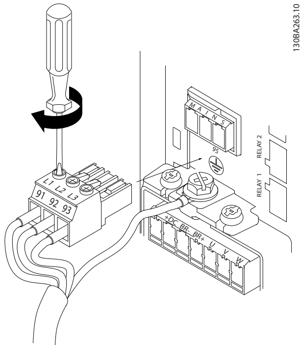
圖 3.10 安裝主電源插頭
