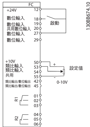
圖 4.2 變頻器接線
