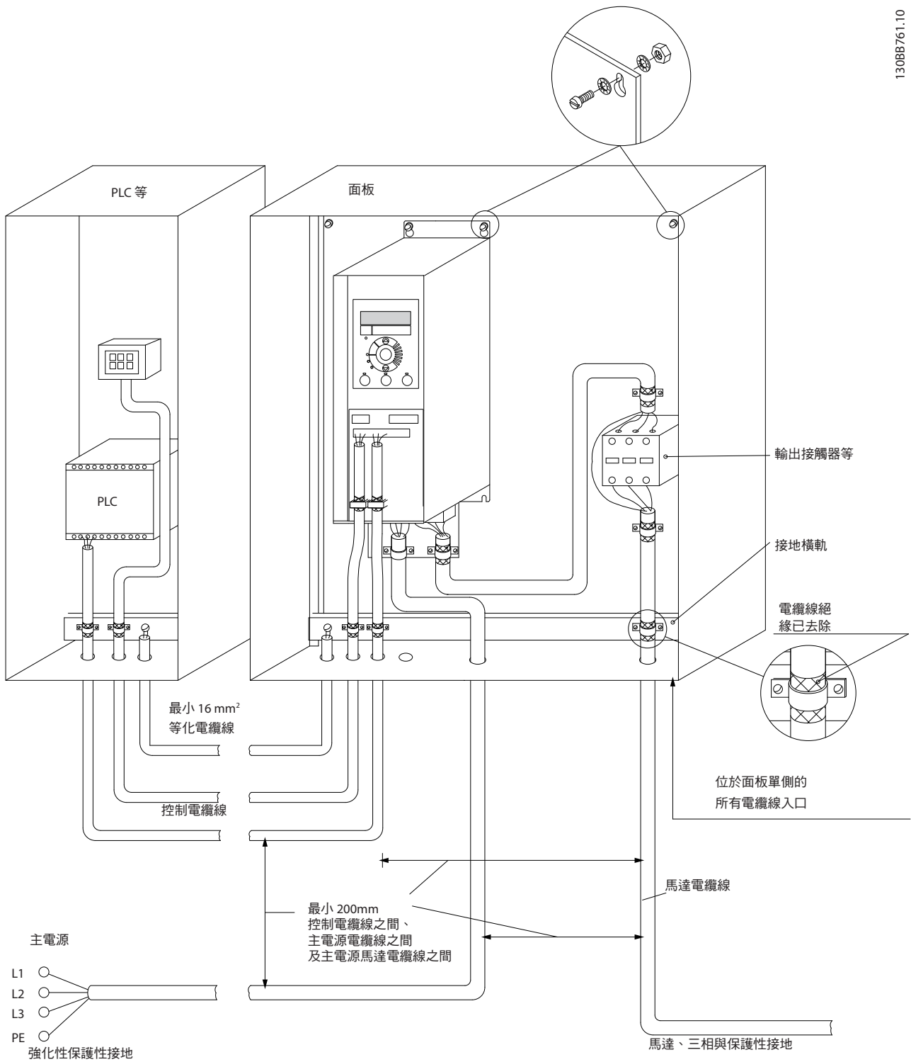
圖 3.21 符合 EMC 規範的電氣安裝
