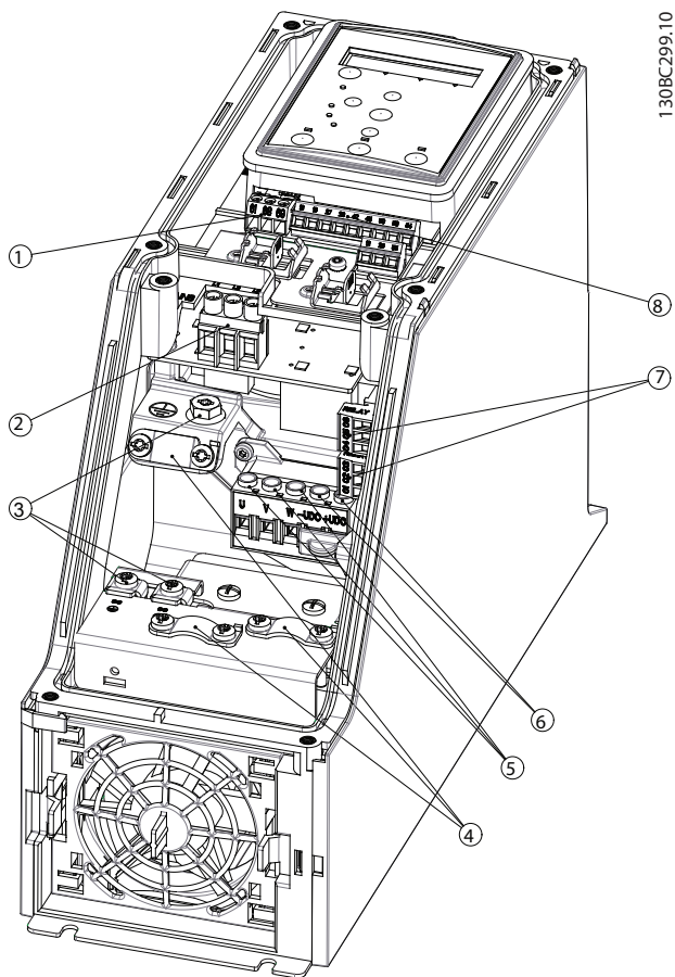
外殼規格 12
