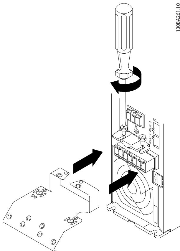
圖 3.8 裝上安裝板
