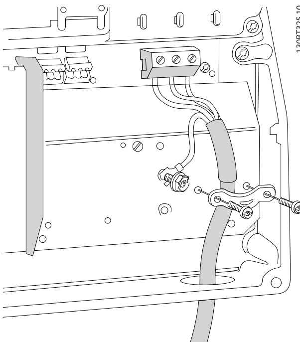
圖 3.18 連接至外殼規格 16 的馬達
