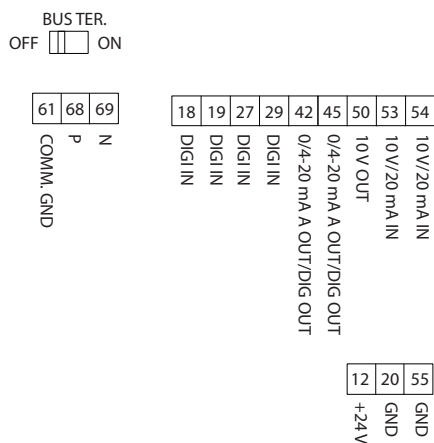
Disegno 3.23 Morsetti di controllo
