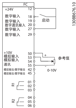
图 4.2 变频器接线
