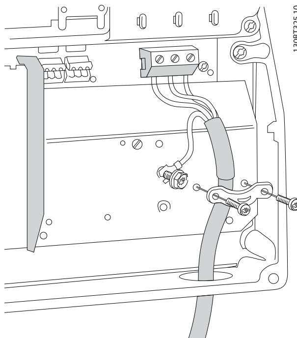
图 3.18 连接电机 — 16 机箱
