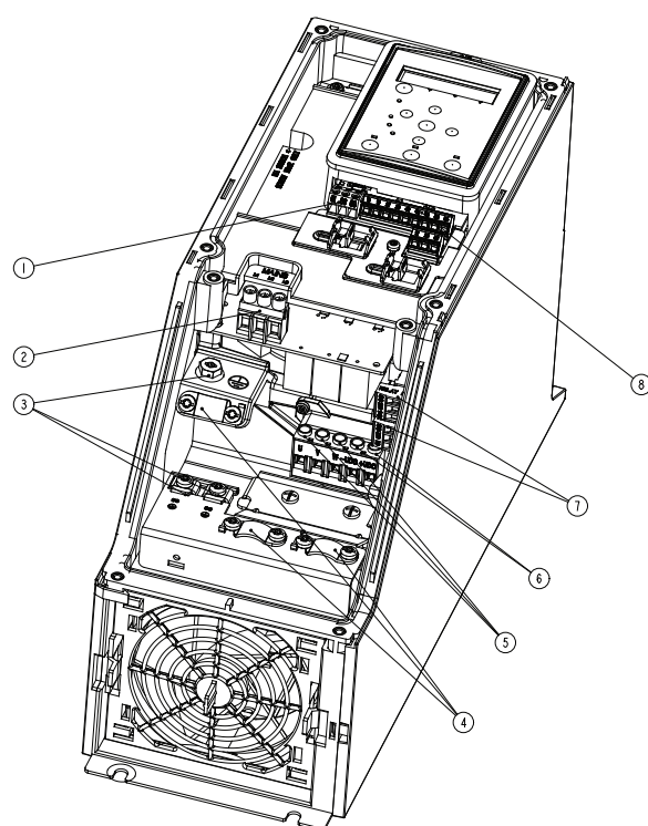
机箱规格 13
