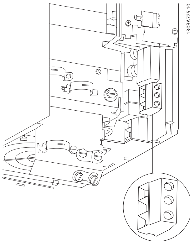
图 3.12 机箱规格 H10 IP20, 600 V, 11 - 15 kW (15 - 20 hp)
