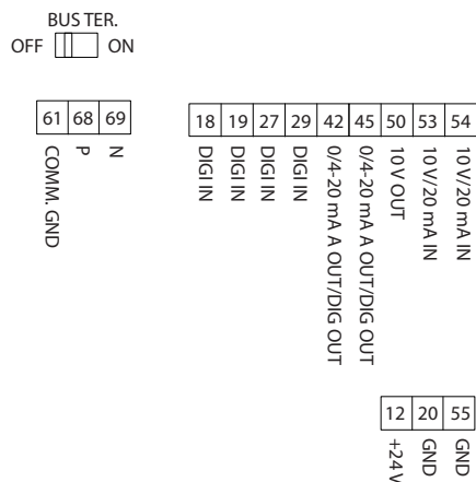
图 3.23 控制端子
