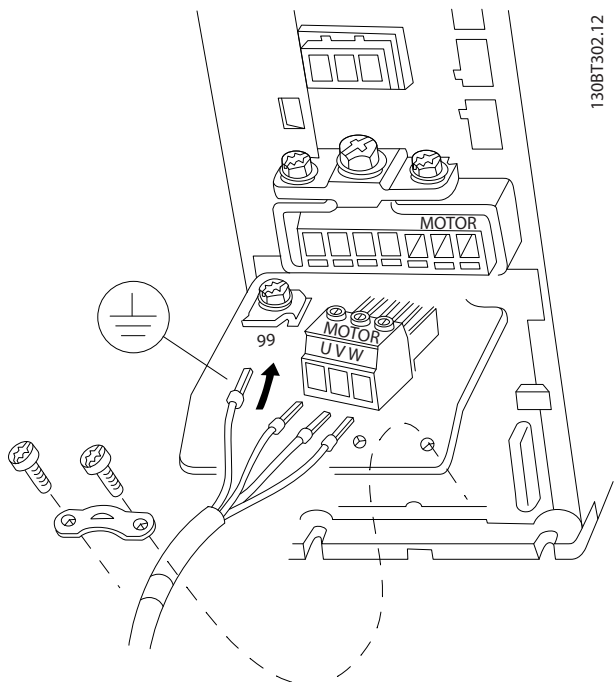
图 3.7 将变频器连接到电机, H9 机箱 IP20, 600 V, 2.2 - 7.5 kW (3.0 - 10 hp)
