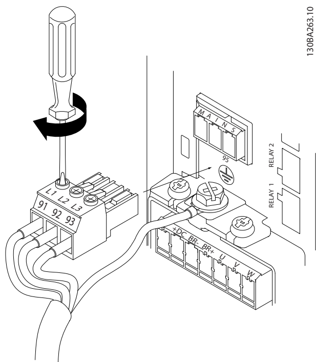
图 3.10 安装主电源插头
