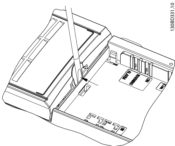
图 3.22 拆下端子盖
