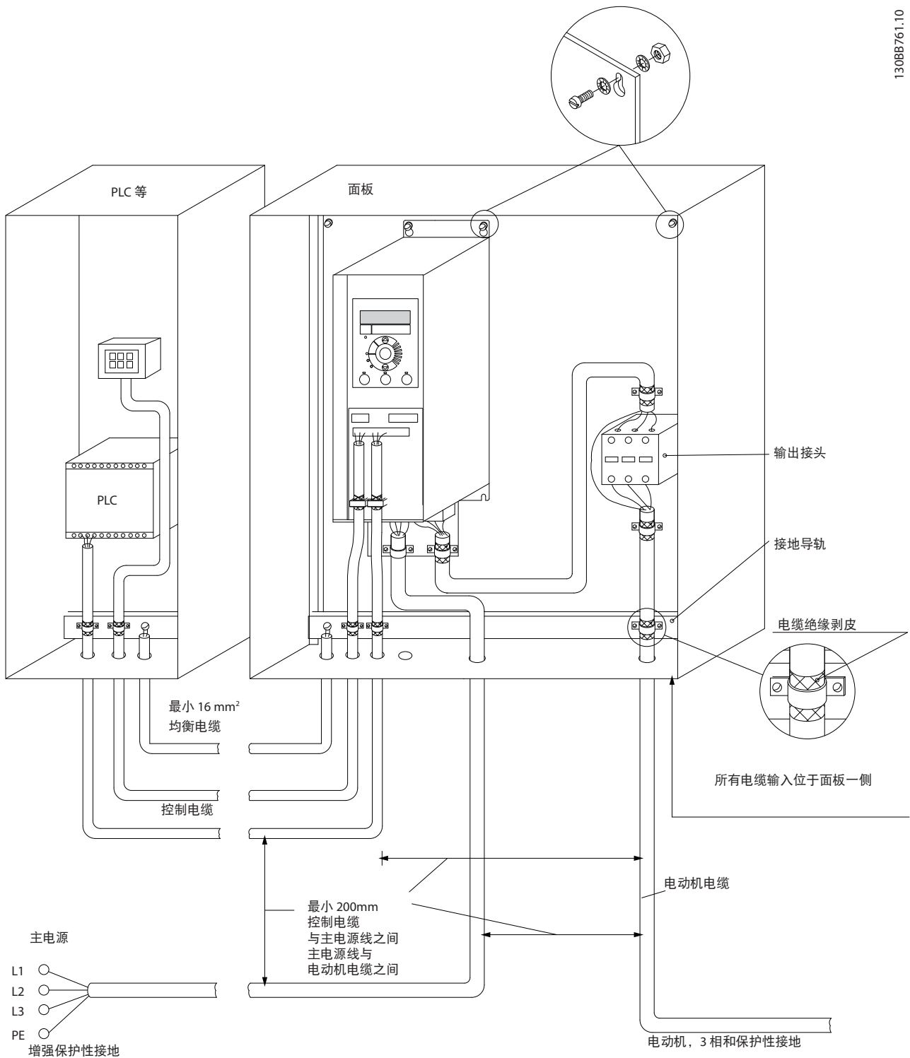
图 3.21 符合 EMC 规范的电气安装
