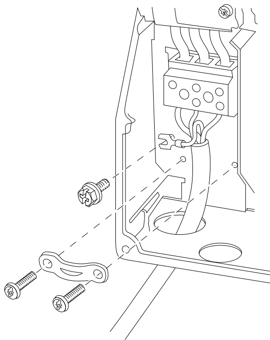
图 3.17 连接主电源 — 16 机箱
