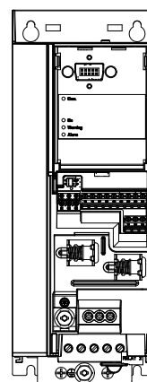
图 7.2 端接器开关的出厂设置
