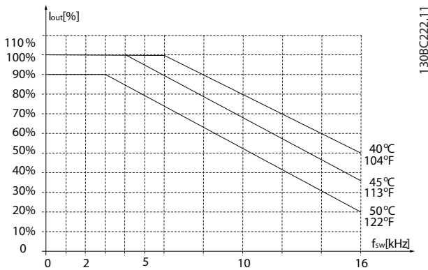
图 3.27 5.5 - 7.5 kW (7.4 - 10 hp), 400 V, 机箱规格 H3, IP20
