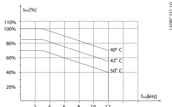
图 3.36 22 - 30 kW (30 - 40 hp), 200 V, 机箱规格 H7, IP20
