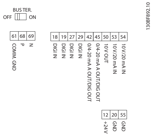
图 5.17 控制端子
