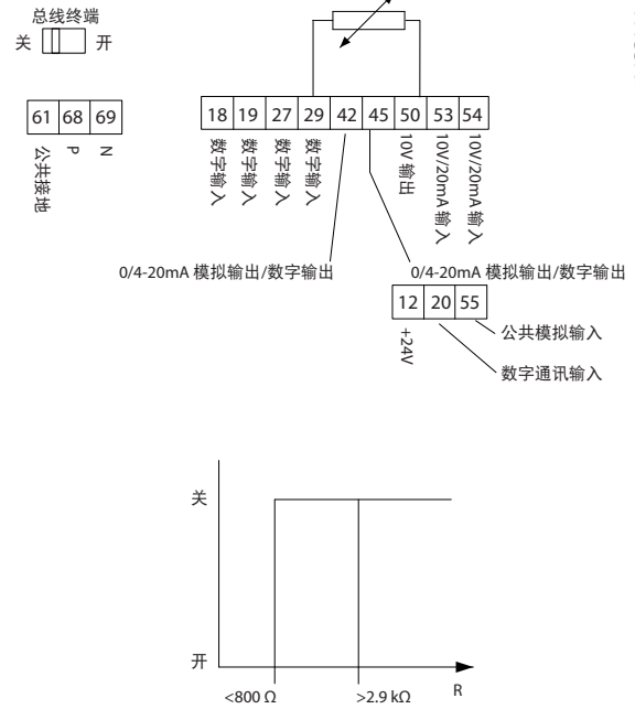
图 3.58 数字输入/10 V 电源
