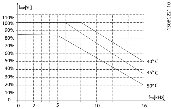
图 3.26 3.7 kW (5.0 hp), 200 V, 机箱规格 H3, IP20
