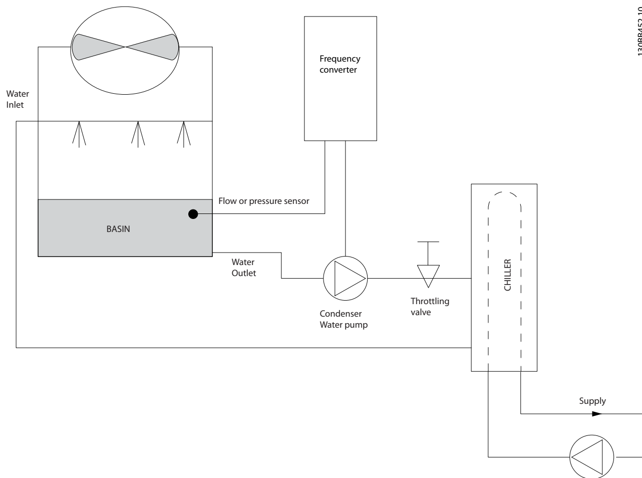
图 3.14 冷凝器泵
