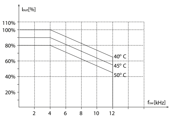
图 3.33 30 - 37 kW (40 - 50 hp), 400 V, 机箱规格 H6, IP20
