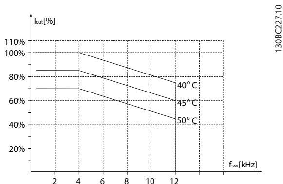
图 3.32 15 - 18.5 kW (20 - 25 hp), 200 V, 机箱规格 H6, IP20
