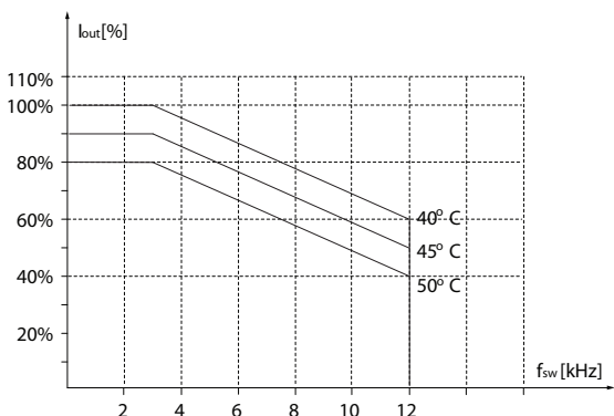
图 3.34 45 kW (60 hp), 400 V, 机箱规格 H6, IP20
