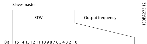
图 7.16 状态字
