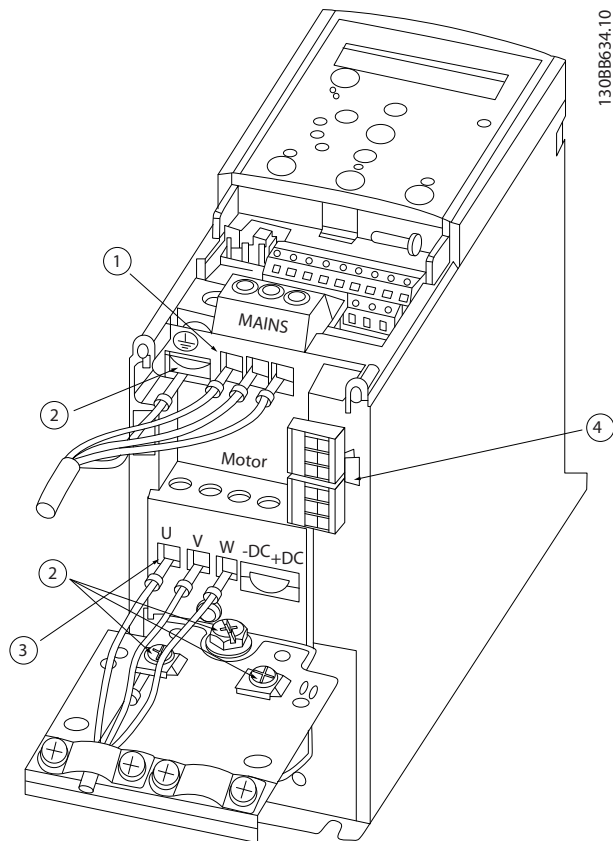
图 5.3 机箱规格 H6
