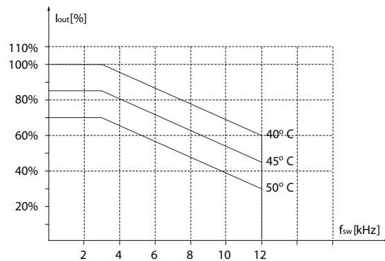
图 3.37 55 - 75 kW (74 - 100 hp), 400 V, 机箱规格 H7, IP20
