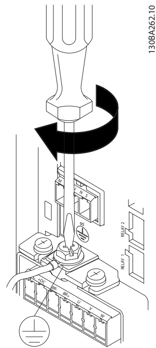
图 1.5 安装电缆时，首先安装并拧紧接地电缆。
