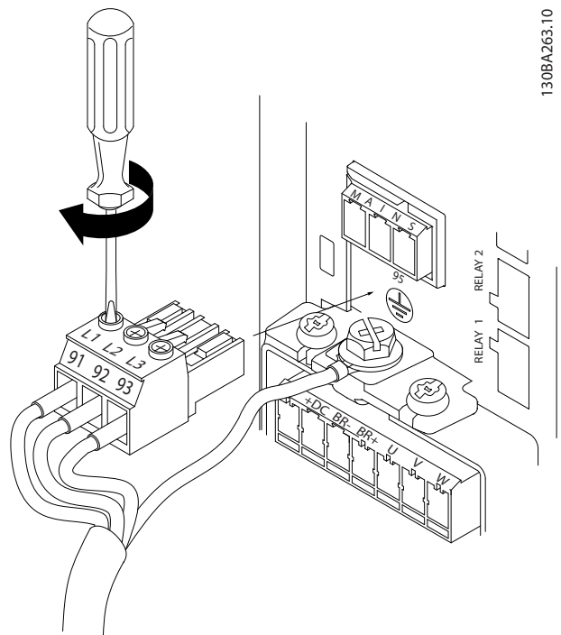
图 1.6 安装主电源插头并拧紧电缆。
