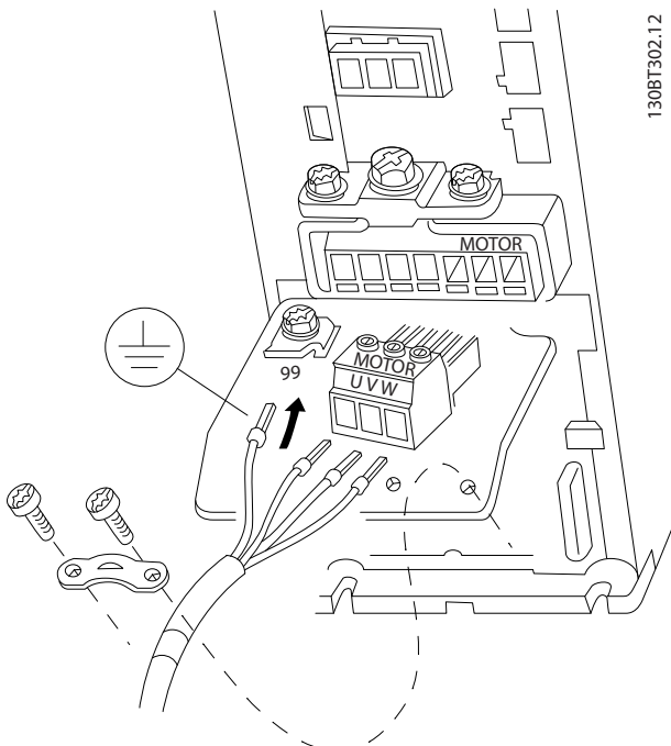
图 1.4 机箱 H3 - H5
