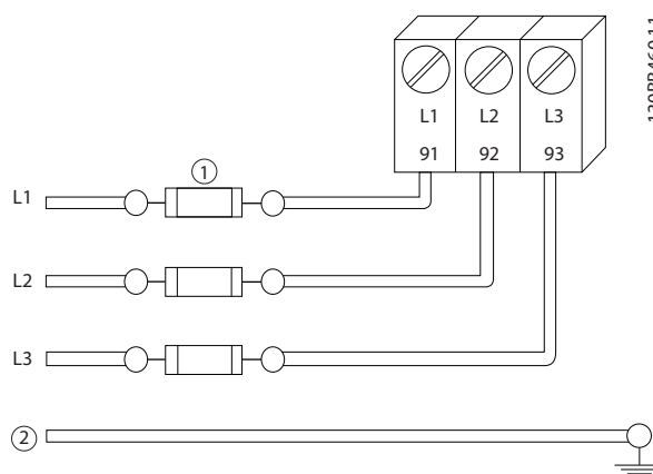
Ábra 2.6 Biztosítékok
