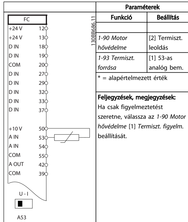
Táblázat 6.12 Motortermisztor
