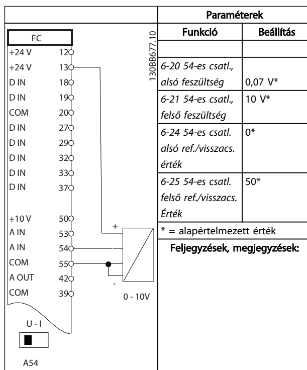
Táblázat 6.3 Analóg feszültségvisszacsatolójel-távadó (4 vezetékes)
