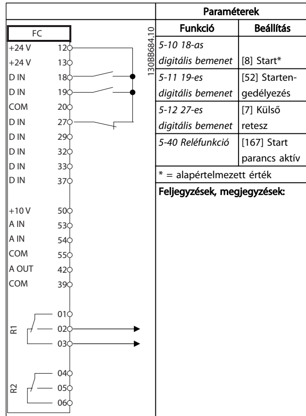
Táblázat 6.10 Startengedélyezés
