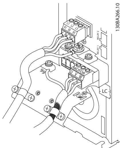
Ábra 2.8 Motor-, hálózati és földelővezetékek A házméret esetén
