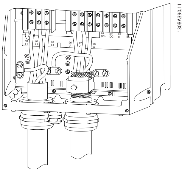
Ábra 2.9 Motor-, hálózati és földelővezetékek B és nagyobb házméretnél, árnyékolt kábelek használata esetén
