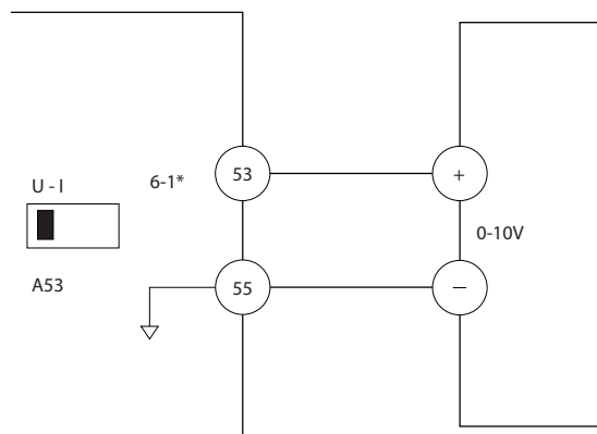
Ábra 5.8 0–10 V-os vezérlőjelet szolgáltató külső készülék bekötési példája (frekvenciaváltó baloldalt, külső készülék jobboldalt)
