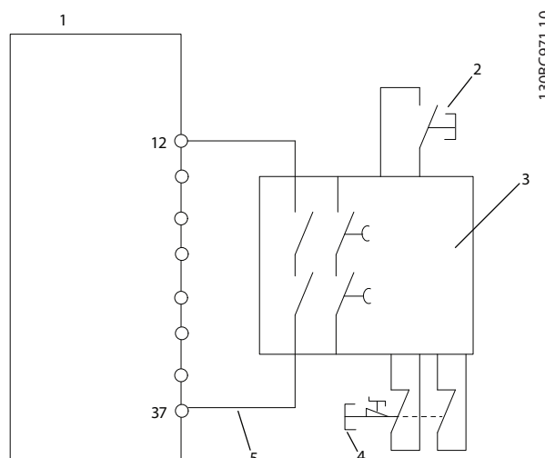
Ilustrasi 1.5 Instalasi untuk Mencapai Kategori Penghentian 0 (EN 60204-1) dengan Cat. /#3 PL "d" (ISO 13849-1 SIL 2) atau (EN 62061).
