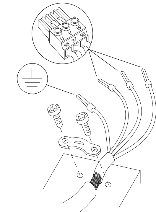
圖 4.5 馬達連接
