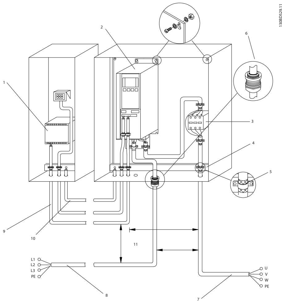
圖 4.2 符合 -EMC 電氣 連接
