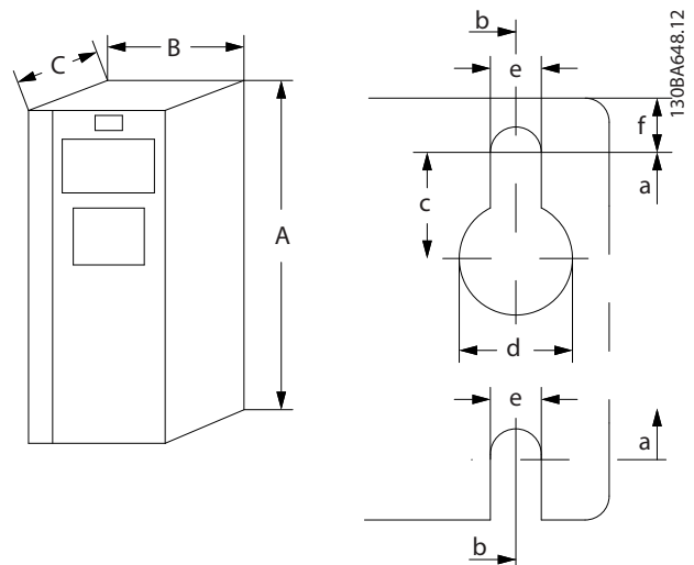
圖 3.4 頂部與底部安裝孔（參閱 章 8.9 額定功率、重量與尺寸）
