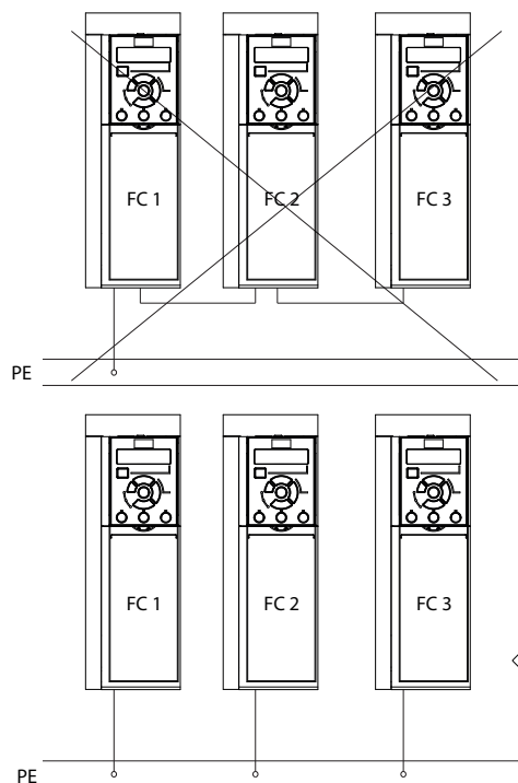
Bild 4.1 Jordningsprincip
