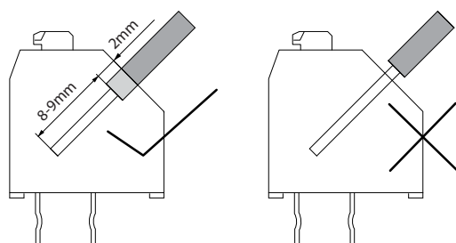
图 7.7 正确的线路插接方式
