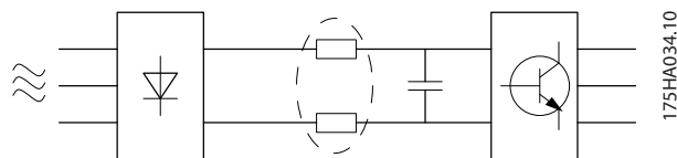
图 3.3 中间电路线圈
