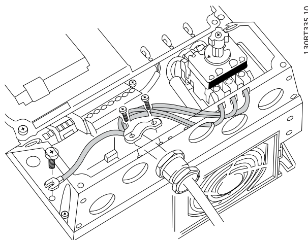
图 8.3 用断路器连接主电源和接地（例如机箱规格 B2 的 S2 型号，其他端子块必须用于主电源连接。
