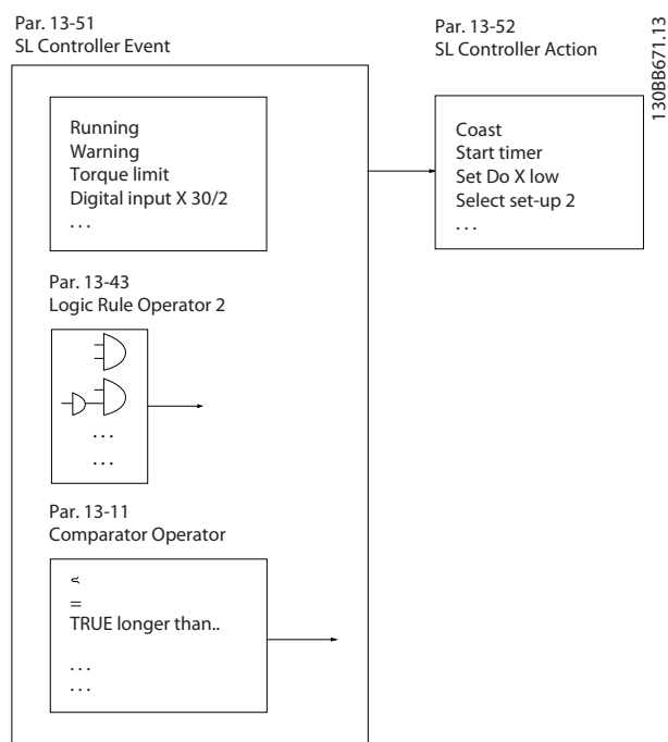
图 2.19 SLC 事件和操作
