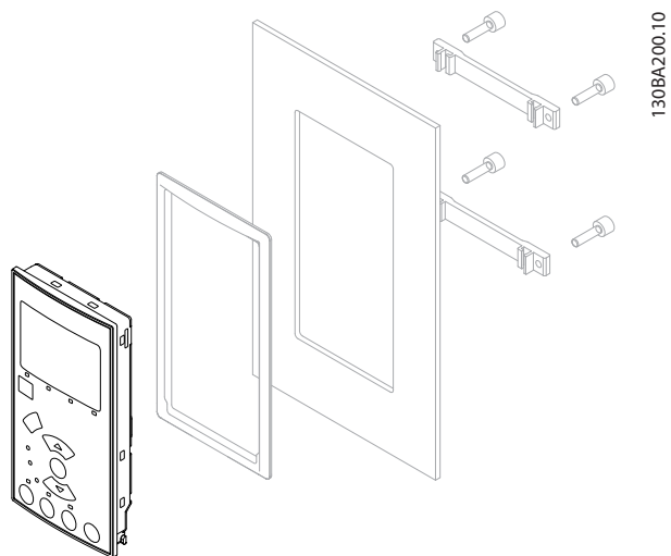
图 3.36 LCP 套件, 包括数字式 LCP、固定件和衬垫。
