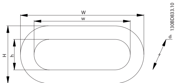
图 6.4 HF-CM 磁芯
