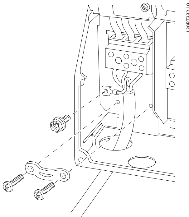
图 8.4 机箱 B1 和 B2 的主电源连接
