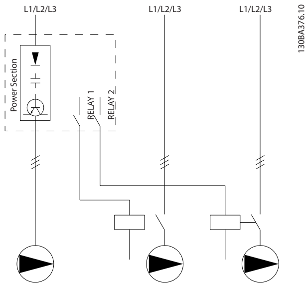
图 4.12 恒速泵/变速泵接线图
