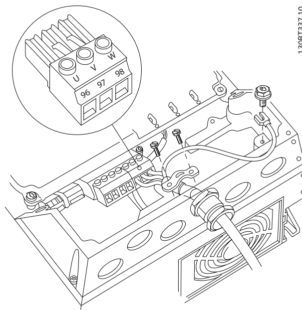
图 8.12 机箱 A4/A5 的电动机连接
