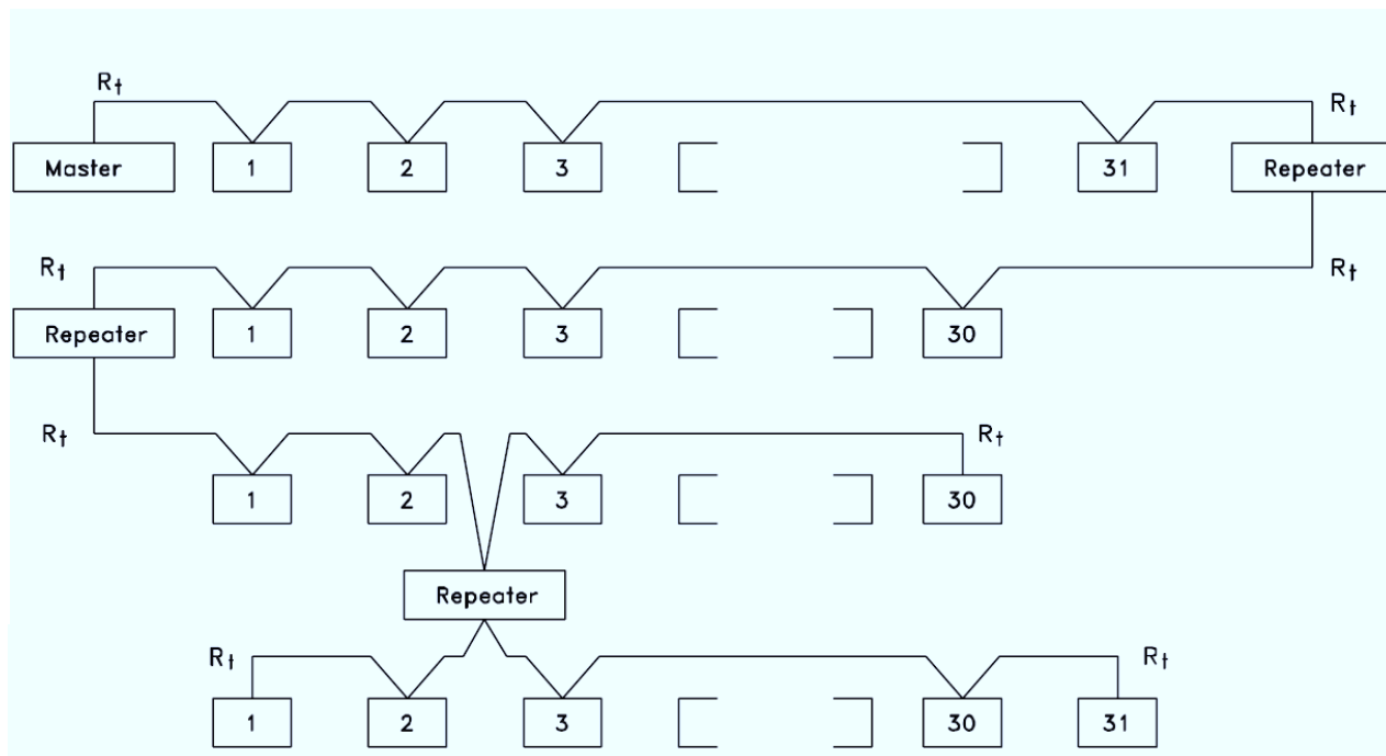
图 3.40 RS 485 总线接口
