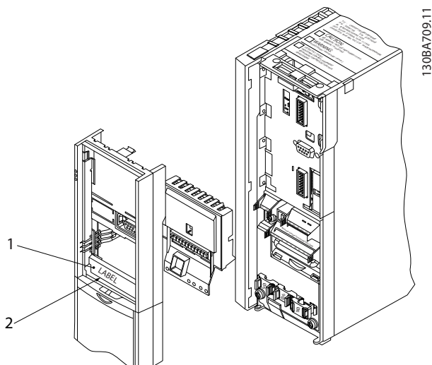
图 7.4 机箱规格 A5-B1-B2-B4-C1-C2-C3-C4
