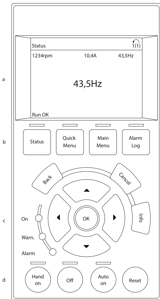
图 2.24 本地控制面板
