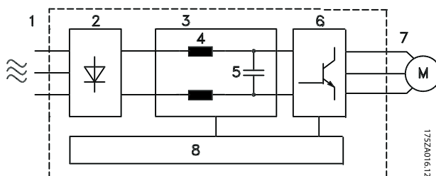
图 2.9 变频器框图
