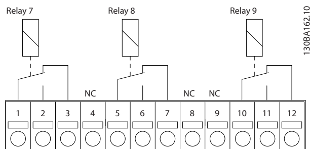
图 7.6 继电器
