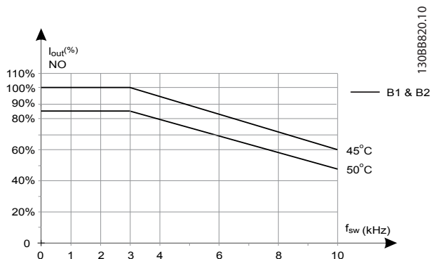
图 5.11 输出电流在不同开关频率和环境温度下的降容 - 600 V 变频器, 机箱类型 B, 60 AVM, 常开
