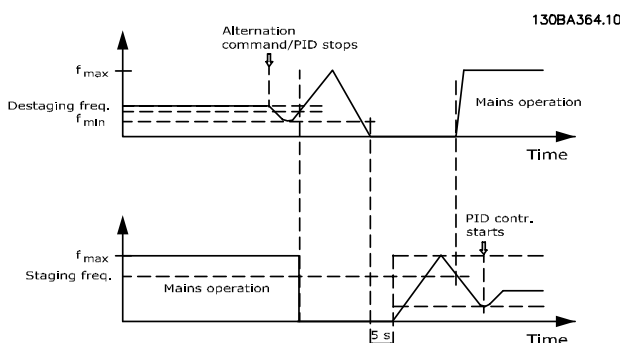
图 4.10 变频泵轮换
