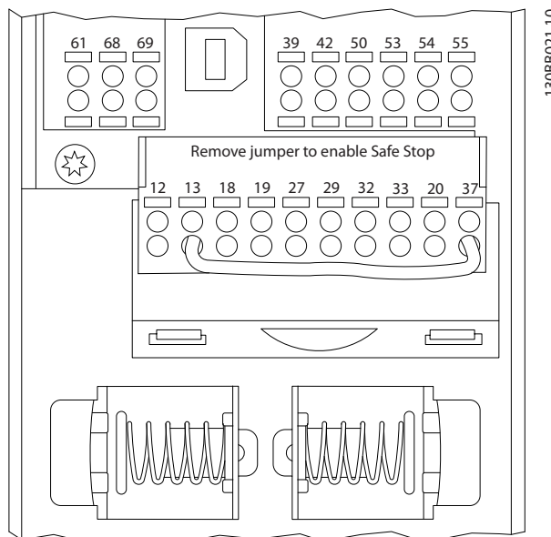
图 3.42 控制卡端子
