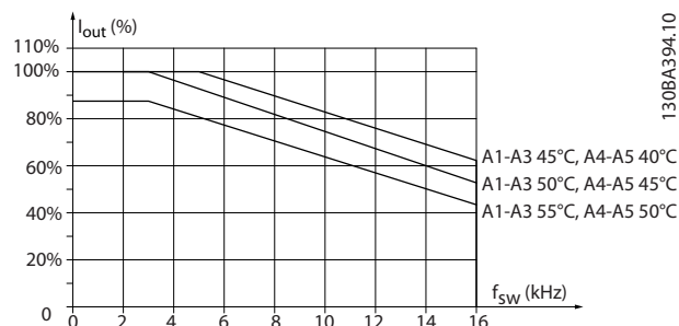
图 5.5 I_{out} 在不同 T_{AMB, MAX} 下的降容 - A 型机箱, 开关模式为 60^{\circ}AVM , 电动机电缆的最大长度不超过 10 m
