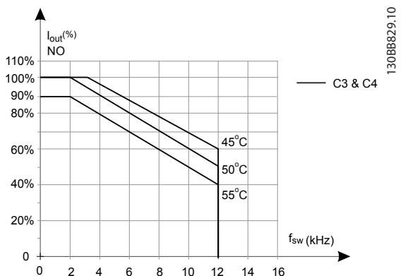
图 5.16 Iout 在不同 TAMB, MAX 下的降容, 机箱规格 C3 和 C4, 在正常过载模式 (110% 过转矩) 下使用 60° AVM
