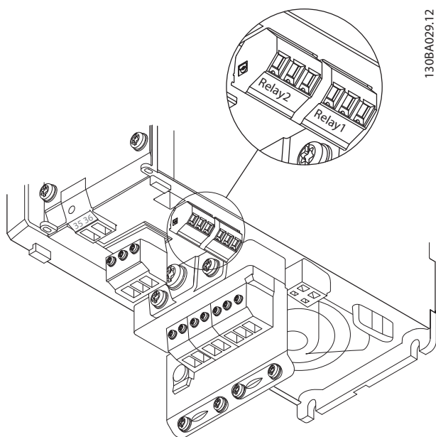
图 8.18 继电器连接端子 (机箱规格 A1、A2 和 A3)。
