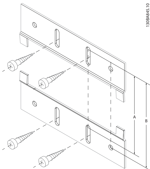
图 3.39 上托架
