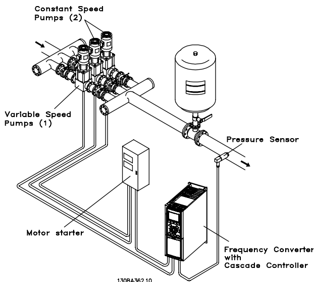
图 4.9 BASIC 多泵控制器
