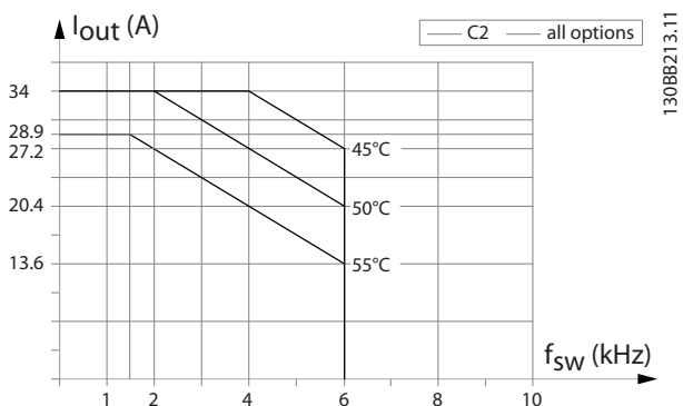
图 5.21 输出电流在不同开关频率和环境温度下的降容 - 机箱类型 C2, 60° AVM。
