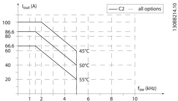
图 5.22 输出电流在不同开关频率和环境温度下的降容 - 机箱类型 C2, SFAVM。
