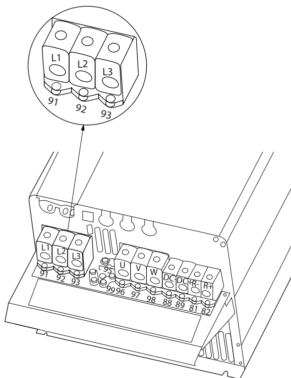
图 8.9 机箱 C4 (IP20) 的主电源连接。
