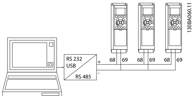
图 3.41 并行连接
