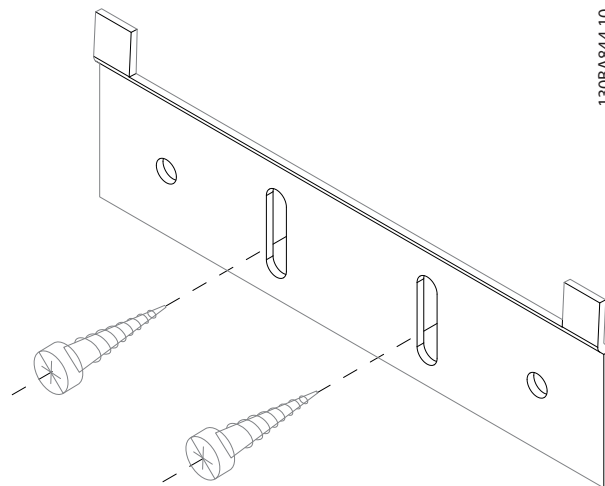
图 3.38 下托架
