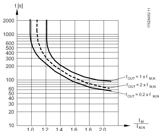
图 2.18 ETR 特性
