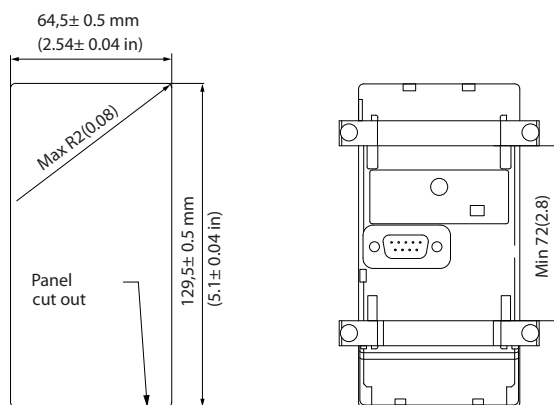
图 3.37 LCP 套件的尺寸
