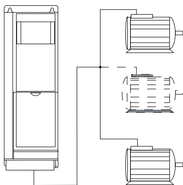
图 3.11 短电缆的共用节点连接
