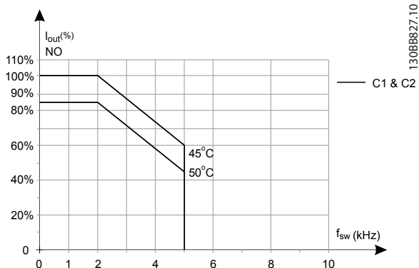
图 5.20 输出电流在不同开关频率和环境温度下的降容 - 600 V 变频器, 机箱类型 C; SFAVM, NO
