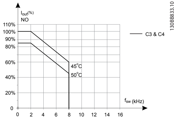
图 5.18 Iout 在不同 TAMB, MAX 下的降容 - 设备规格 C3 和 C4, 在正常过载模式 (110% 过转矩) 下使用 SFAVM
