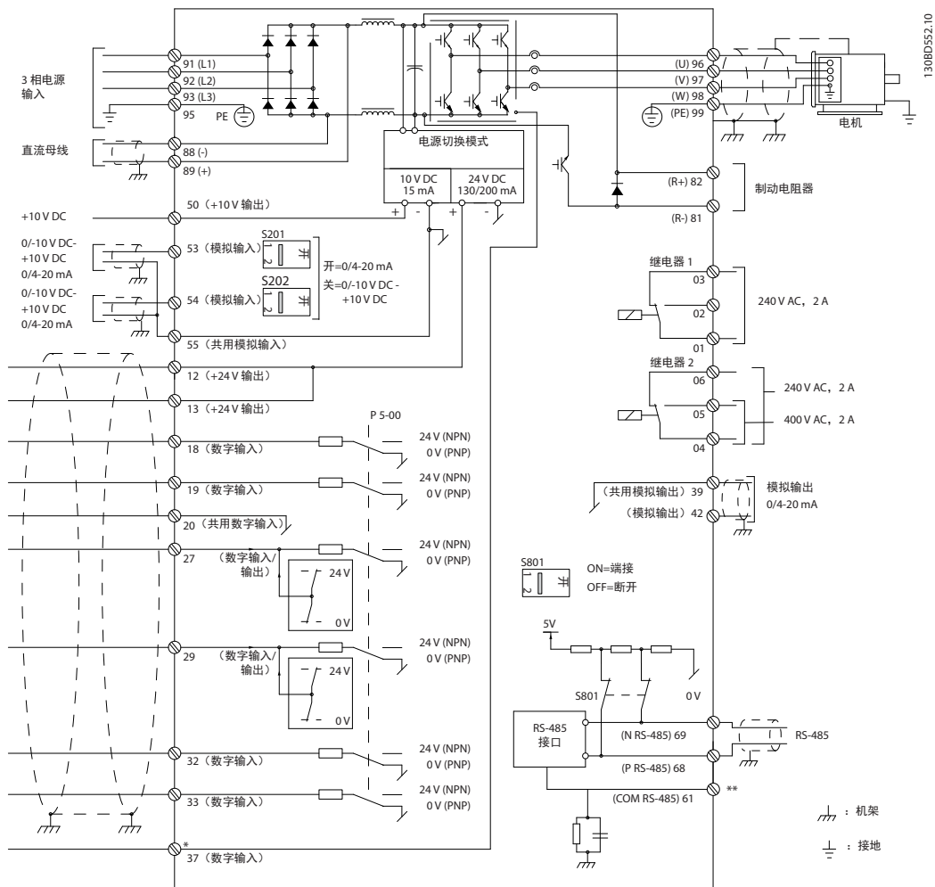
图 3.20 基本接线示意图
