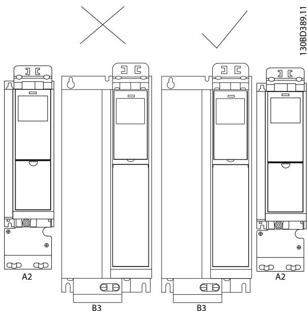
图 3.23 正确的无间隙并排安装
