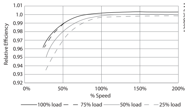
图 3.19 典型效率曲线
