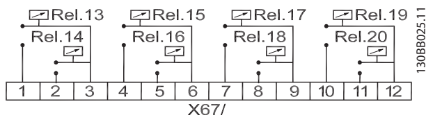
图 7.19 高级多泵控制器 MCO 102 的端子连接, 8 个继电器
