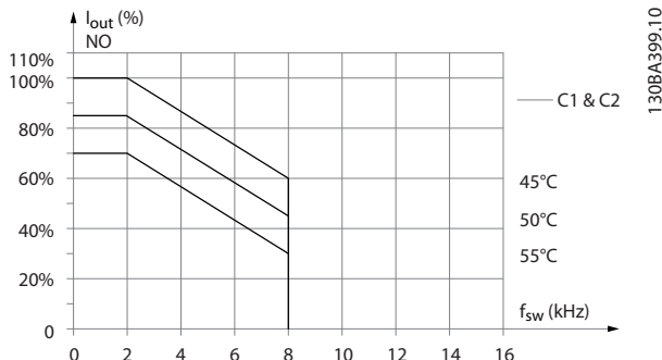
图 5.17 Iout 在不同 TAMB, MAX 下的降容, 机箱规格 C1 和 C2, 在正常过载模式 (110% 过转矩) 下使用 SFAVM
