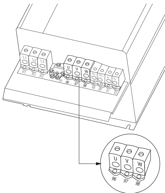
图 8.17 C3 和 C4 机箱的电动机连接
