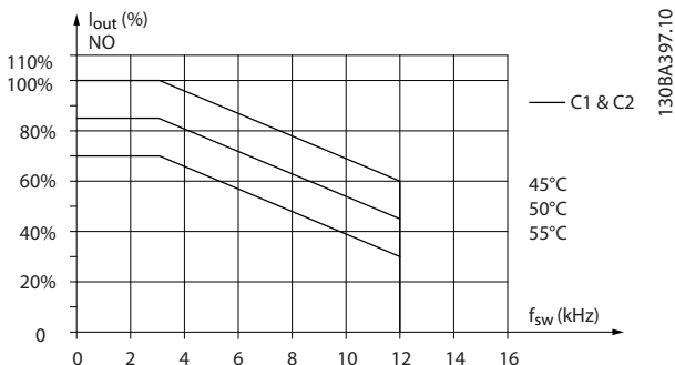
图 5.15 Iout 在不同 TAMB, MAX 下的降容, 机箱规格 C1 和 C2., 正常过载模式下使用 60° AVM (110% 过转矩)
