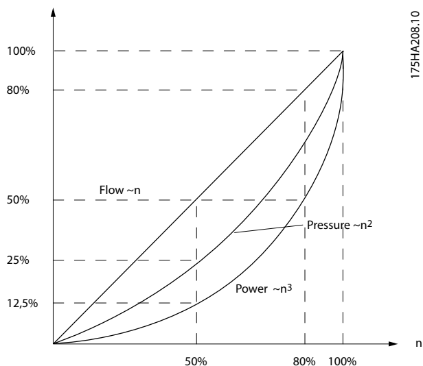
图 2.2 离心泵相似定律
