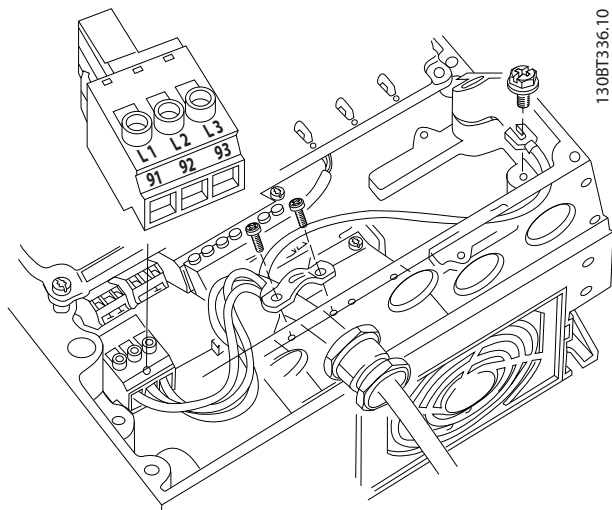
图 8.2 不用断路器连接主电源和接地
