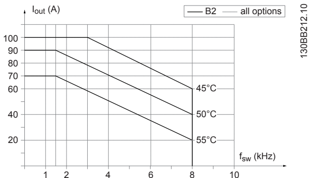
图 5.14 输出电流在不同开关频率和环境温度下的降容 - 机箱类型 B2 和 B4, SFAVM。
