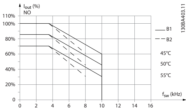
图 5.9 I_{out} 在不同 T_{AMB, MAX} 下的降容 - 机箱类型 B1 和 B2, 在正常过载模式 (110% 过转矩) 下使用 SFAVM
