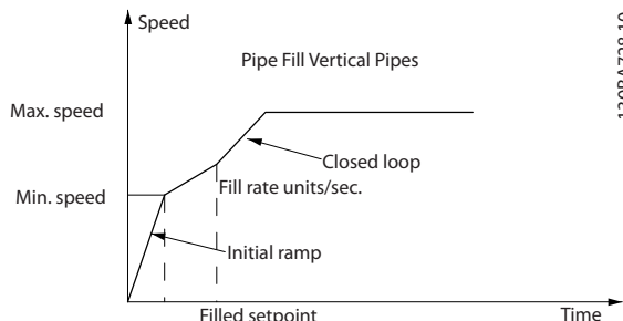
图 4.8 管道填充模式，性能曲线
