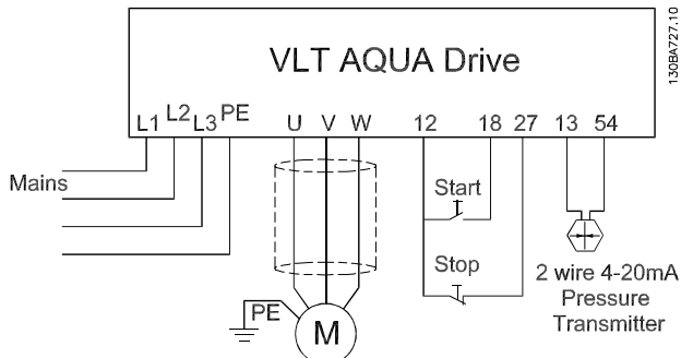
图 4.7 潜水泵应用接线
