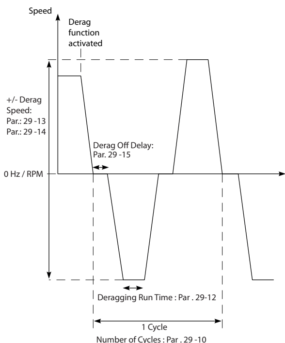
图 4.1 除屑功能
