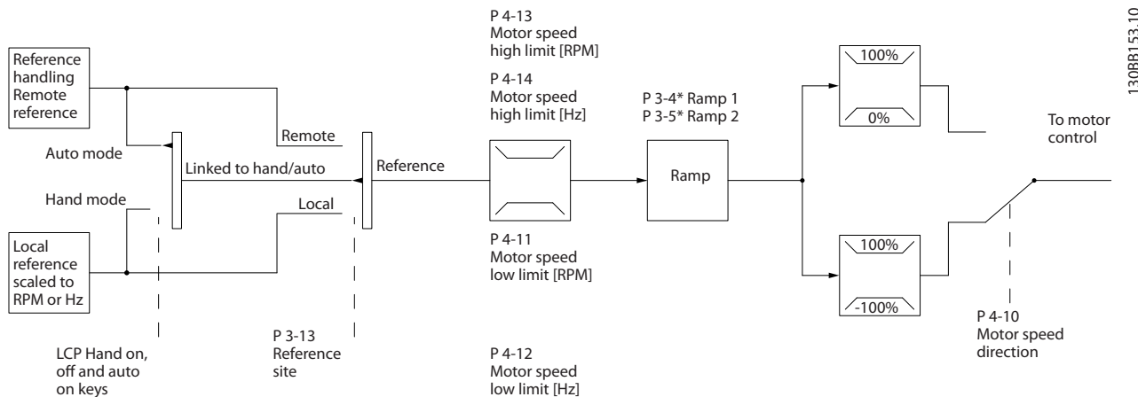
图 2.11 开环模式框图
