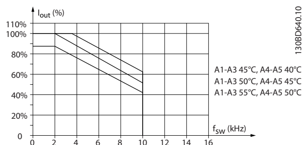
图 5.6 I_{out} 在不同 T_{AMB, MAX} 下的降容 - A 型机箱, 开关模式为 SFAVM, 电动机电缆的最大长度不超过 10 m
