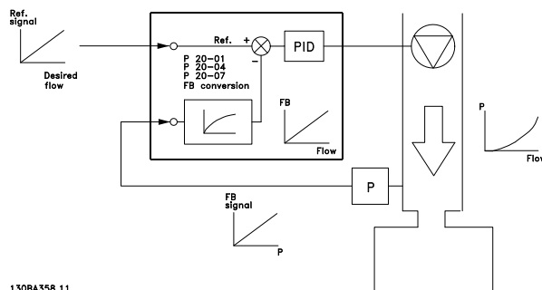
图 2.17 反馈转换
