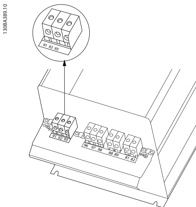
图 8.8 机箱 C3 (IP20) 的主电源连接。
