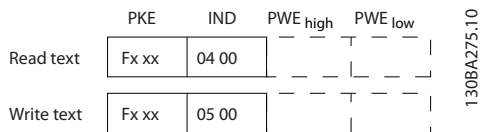
图 3.50 通过 PWE 块输入的文本
