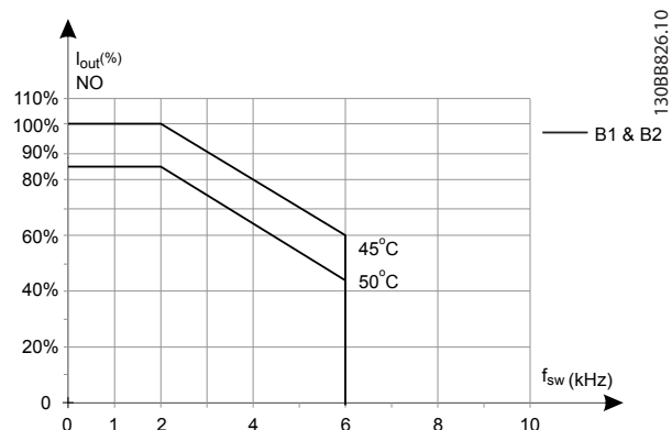
图 5.12 输出电流在不同开关频率和环境温度下的降容 - 600 V 变频器, 机箱类型 B; SFAVM, NO
