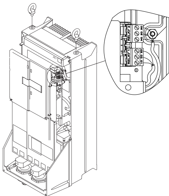
图 8.19 继电器连接端子 (机箱规格 C1 和 C2)
