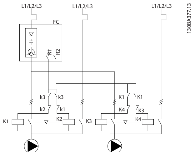
图 4.13 变频泵轮换接线图
