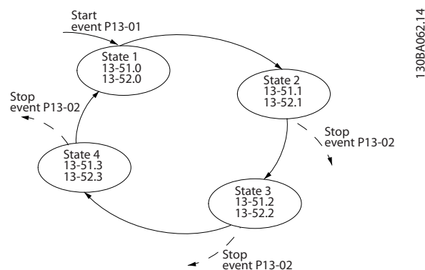
图 2.20 对 4 个事件/操作编程时的执行顺序
