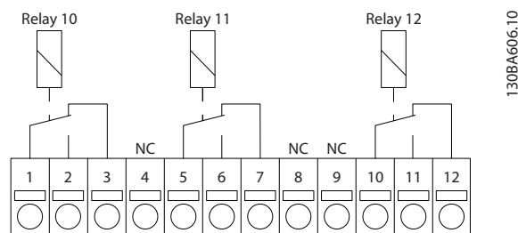
图 7.14 连接用途
