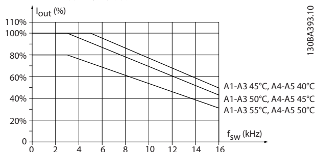
图 5.3 I_{out} 在不同 T_{AMB, MAX} 下的降容 (机箱规格 A), 采用 60^{\circ}AVM
