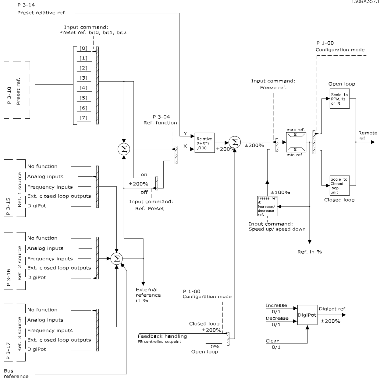
图 2.15 框图显示了远程参考值处理
