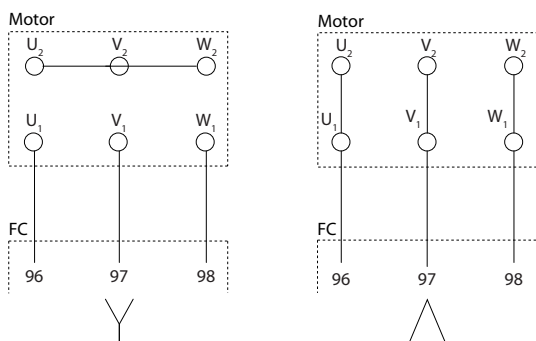
图 8.10 星形和三角形连接
