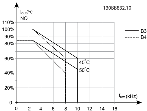
图 5.10 I_{out} 在不同 T_{AMB, MAX} 下的降容 - 机箱类型 B3 和 B4, 在正常过载模式 (110% 过转矩) 下使用 SFAVM
