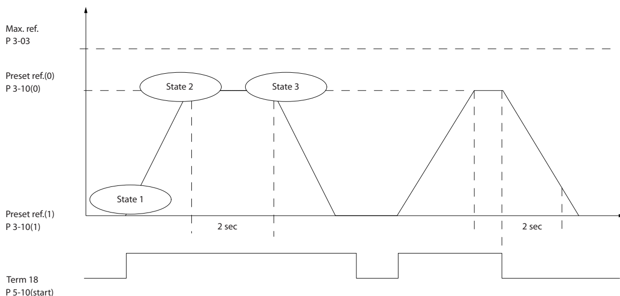
图 4.5 加速/减速
