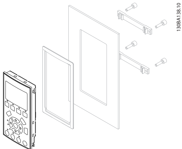
图 3.35 LCP 套件, 包括图形 LCP、固定件、3 米长电缆和衬垫。
