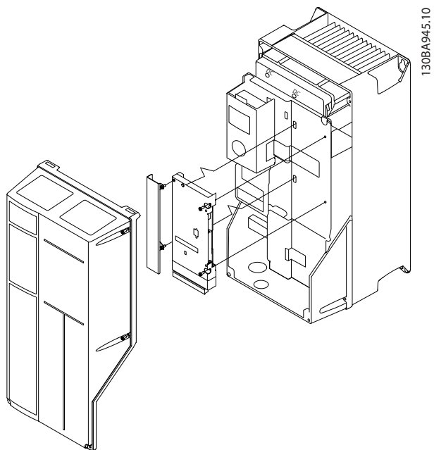
图 7.18 机箱 B (B3 除外) 和 C。
