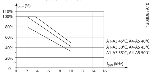
图 5.4 I_{out} 在不同 T_{AMB, MAX} 下的降容 - 使用 SFAVM 的机箱类型 A
