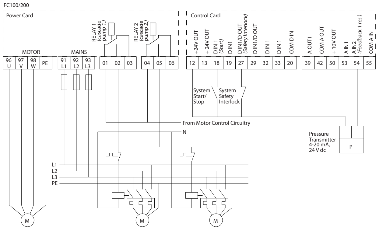
图 4.11 多泵控制器接线图
