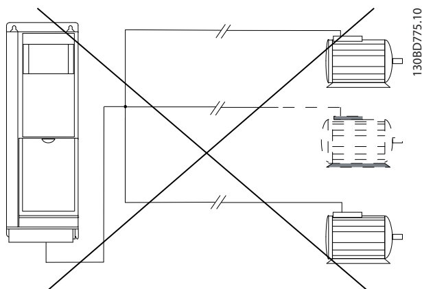
图 3.12 长电缆的共用节点连接
