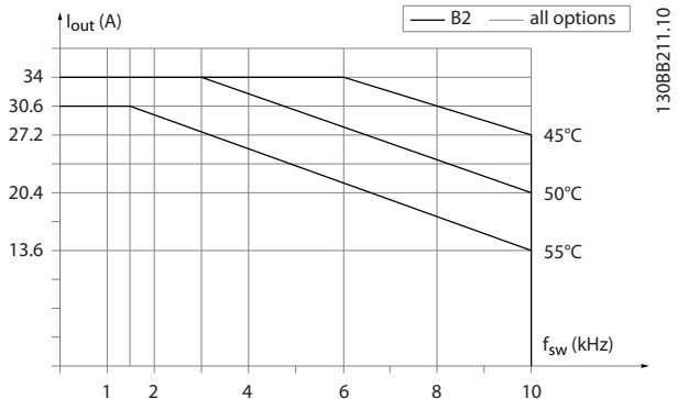
图 5.13 输出电流在不同开关频率和环境温度下的降容 - 机箱类型 B2 和 B4, 60° AVM。
