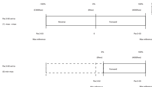
图 3.58 参考值和 MAV
