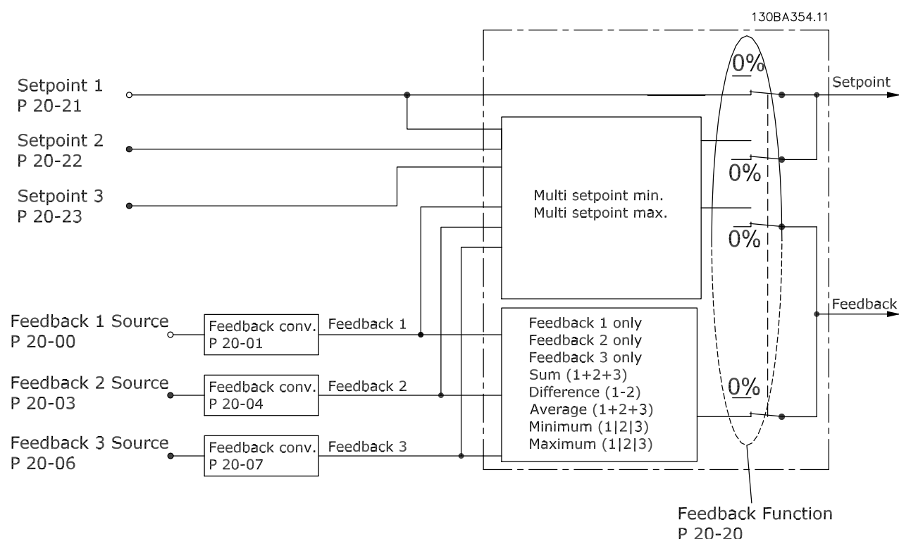
图 2.16 反馈信号处理框图
