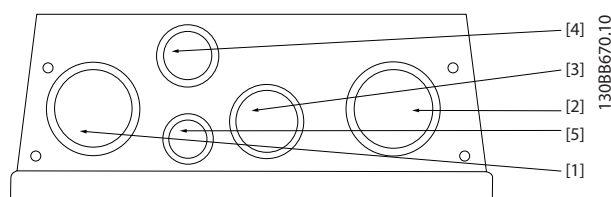
图 8.31 机箱规格 B2, IP55
