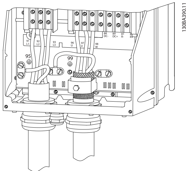
图 8.16 机箱 C1 和 C2 的电动机连接 (IP21/NEMA 类型 1 和 IP55/66/NEMA 类型 12)
