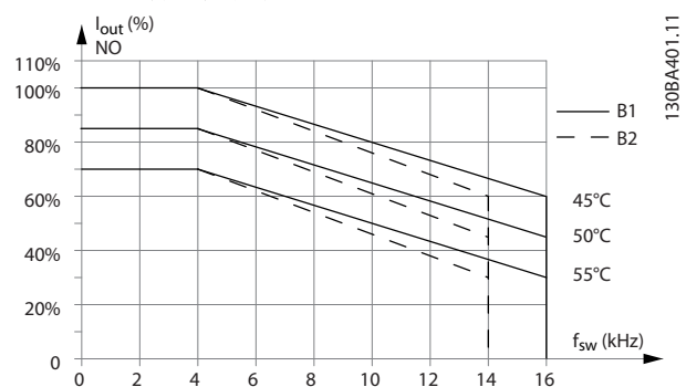
图 5.7 I_{out} 在不同 T_{AMB, MAX} 下的降容 - 机箱类型 B1 和 B2, 在正常过载模式 (110% 过转矩) 下使用 60^{\circ}AVM
