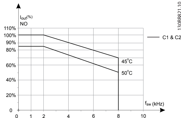
图 5.19 输出电流在不同开关频率和环境温度下的降容 - 600 V 变频器, 机箱类型 C, 60 AVM, 常开
