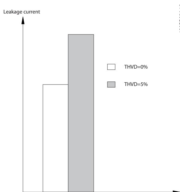
图 3.7 线路失真会影响漏电电流
