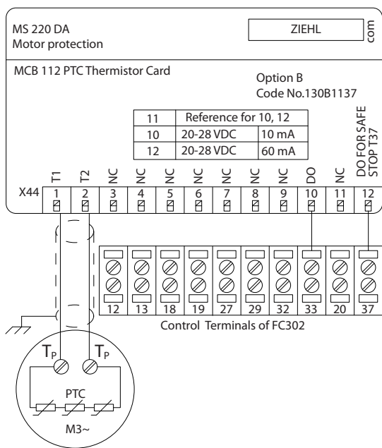
图 7.9 安装 MCB 112
