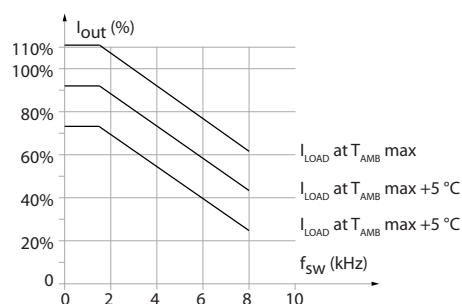
图 5.23 输出电流在不同开关频率和环境温度下的降容 - 机箱类型 C3。
