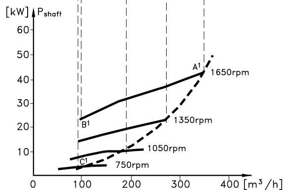
图 2.7 不同速度的能耗
