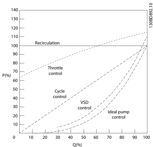
图 2.5 流量控制曲线比较
