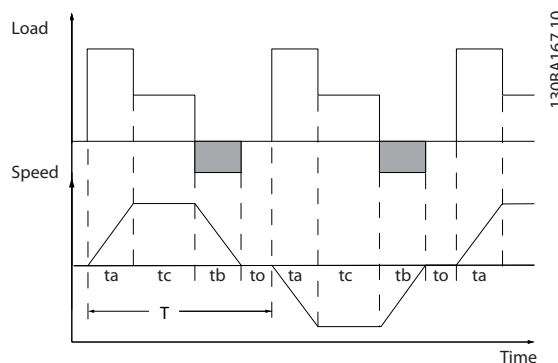
图 3.18 制动电阻器工作周期
