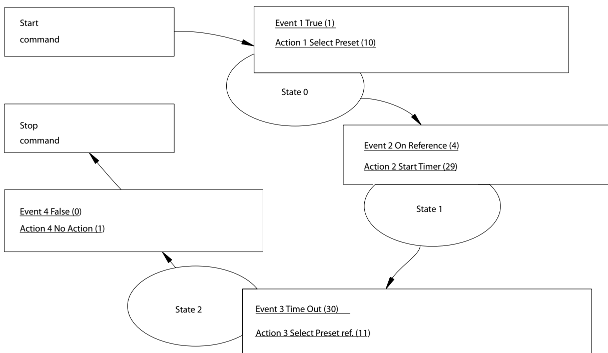
图 4.6 SLC 应用范例
