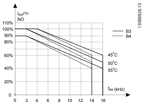
图 5.8 I_{out} 在不同 T_{AMB, MAX} 下的降容 - 机箱类型 B3 和 B4, 在正常过载模式 (110% 过转矩) 下使用 60° AVM
