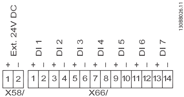
图 7.20 高级多泵控制器 MCO 102 端子连接, 7 数字输入和访问内部的直流 24 V
