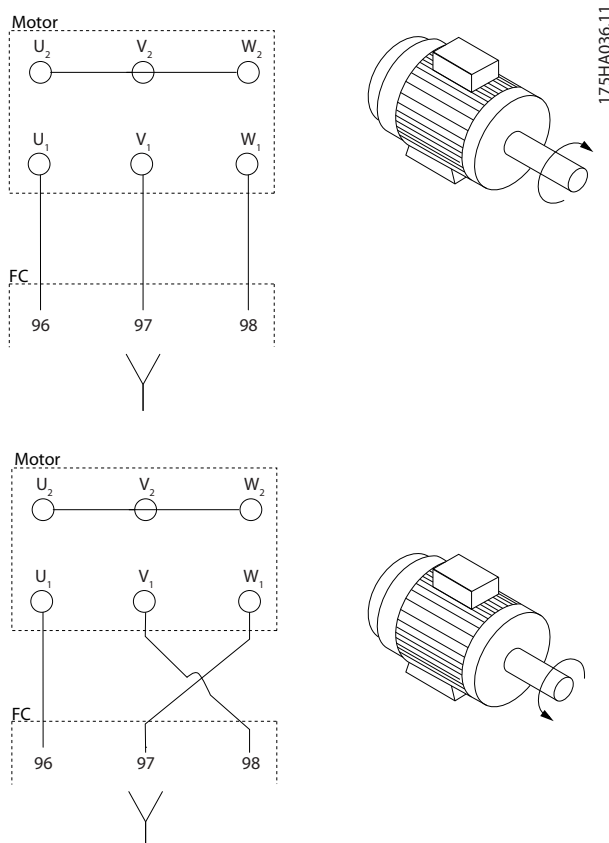
图 3.10 顺时针和逆时针旋转的端子连接
