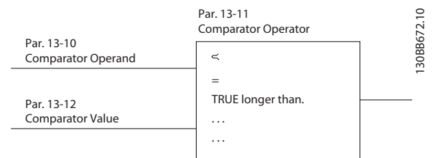
Рисунок 2.21 Компараторы
