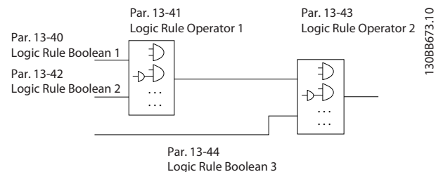
Рисунок 2.22 Логические соотношения
