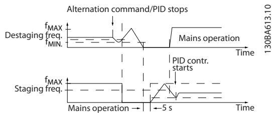
Рисунок 3.79 Конфигурация с медленным режимом
