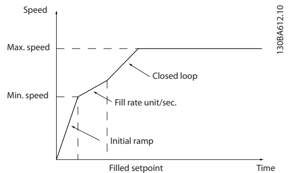
Рисунок 3.82 Вертикальная трубопроводная система
