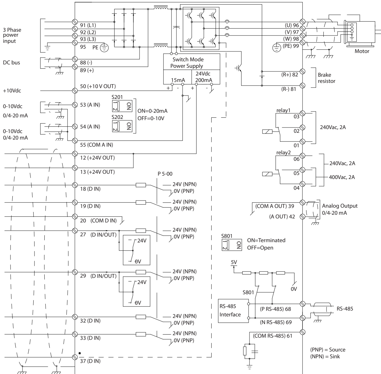
Рисунок 1.2 На схеме показаны все электрические клеммы без дополнительных устройств.
