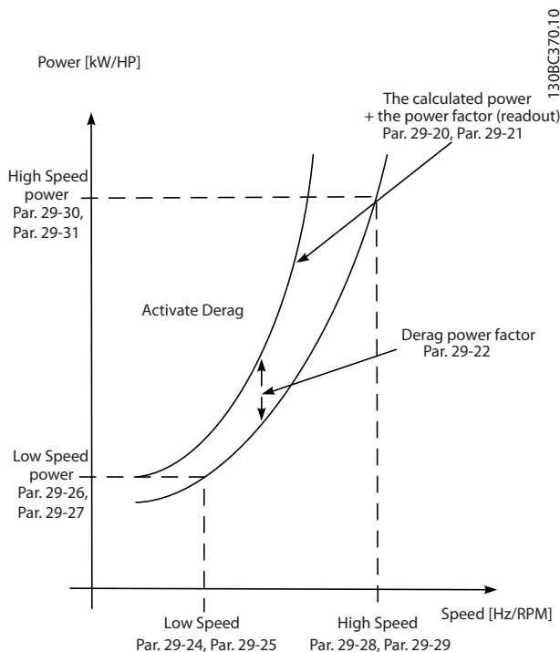
Рисунок 3.84 Derag Power Tuning (Настройка мощности очистки)
