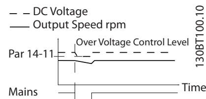
Рисунок 3.39 Кинетический резерв, короткое замыкание сети. Скачок длится, пока в системе есть энергия.
