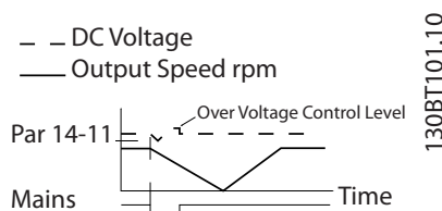
Рисунок 3.37 Управляемое замедление — короткое замыкание сети. После замедления и остановки следует разгон до заданного значения.
