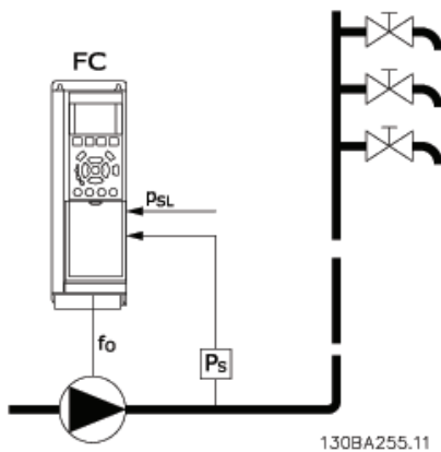
Рисунок 3.51 Условные обозначения: FC=преобразователь частоты; fo=частотный выход; Ps=P системы; PsL=P задан.
