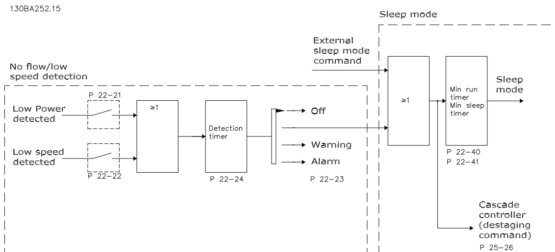
Рисунок 3.48 Схема потока сигналов
