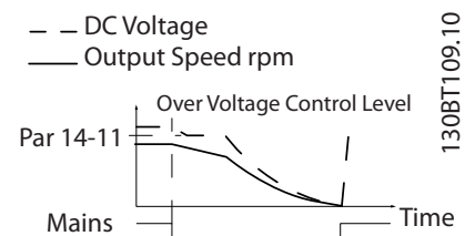
Рисунок 3.40 Кинетический резерв, более длительное замыкание сети. Двигатель останавливается выбегом, как только энергия в системе падает слишком низко.
