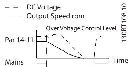
Рисунок 3.38 Управляемое замедление, более длительное замыкание цепи. Замедление длится до тех пор, пока в системе остается энергия, после этого двигатель останавливается выбегом.
