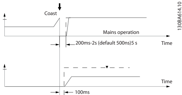
Рисунок 3.80 Конфигурация с быстрым режимом
