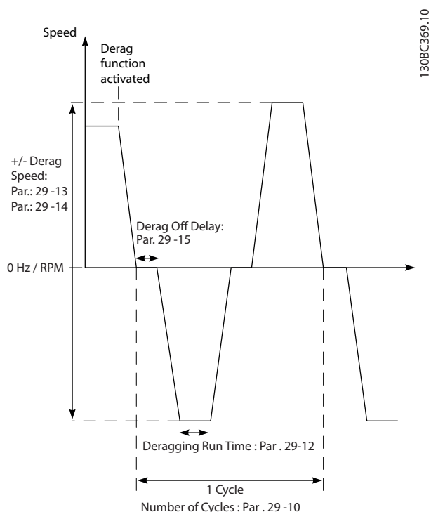
Рисунок 3.83 Функция очистки
