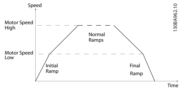
Рисунок 3.18 Время начального и конечного изменения скорости
