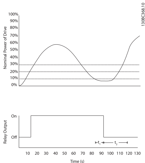
Рисунок 3.28 Пример выходной функции
