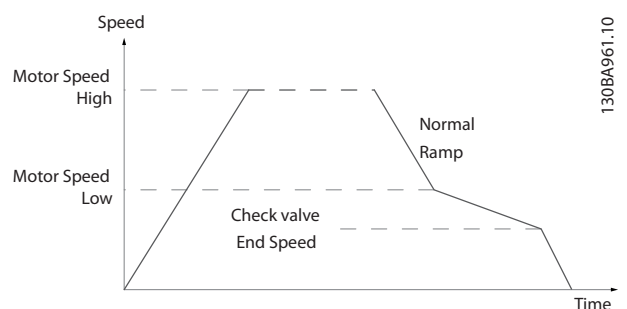
Рисунок 3.19 Изменение скорости контрольного клапана
