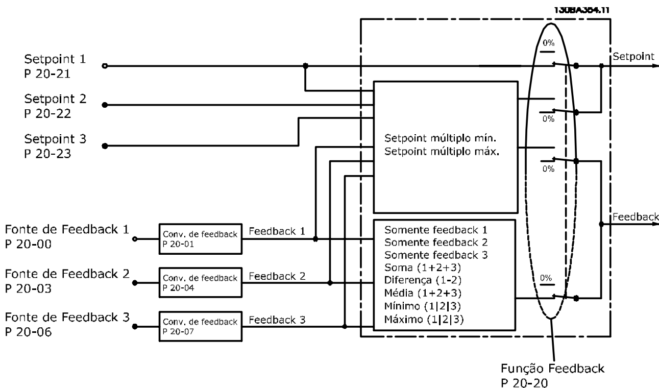
Ilustração 3.51 Sinais de Entrada no Controlador PID de Malha Fechada
