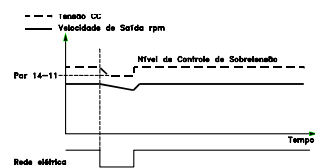
Ilustração 3.47 Backup Cinético, falha de rede elétrica de curta duração.
