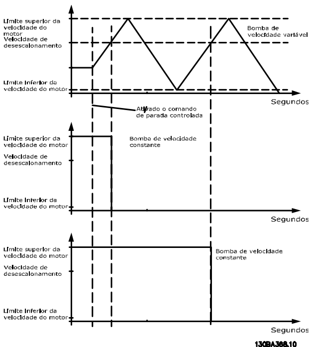
Ilustração 3.84 Velocidade de Desescalonamento
