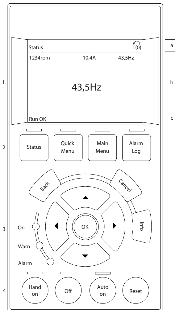
Ilustração 2.1 Painel de controle (LCP)
