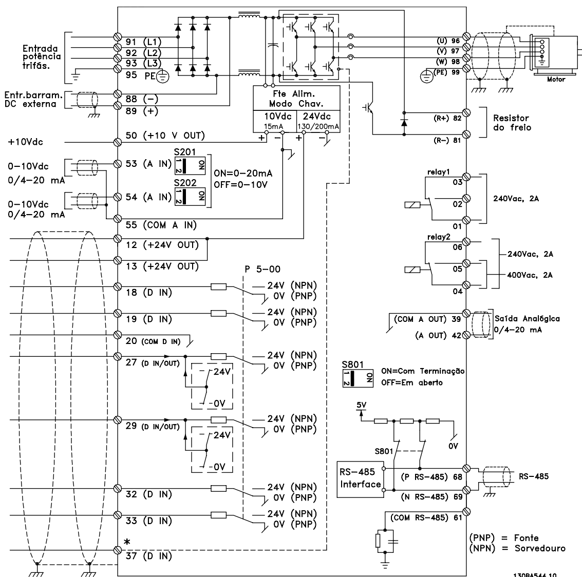
Ilustração 1.2 Desenho Esquemático de Fiação Básica
