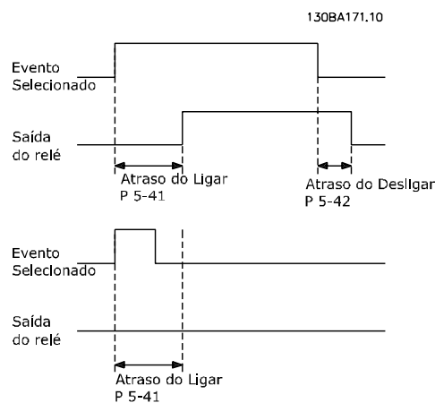
Ilustração 3.25 Atraso de Ativação do Relé
