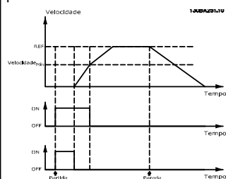
Ilustração 3.24 Princípio de Controle da Válvula de Bypass
