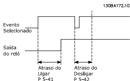
Ilustração 3.26 Atraso de desabilitação, Relé
