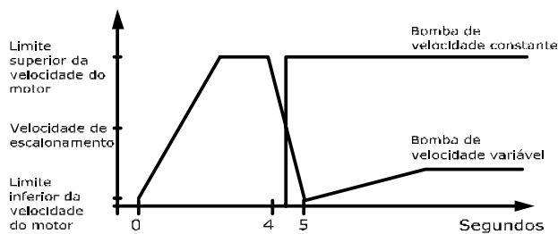
Ilustração 3.82 Limite de Escalonamento
