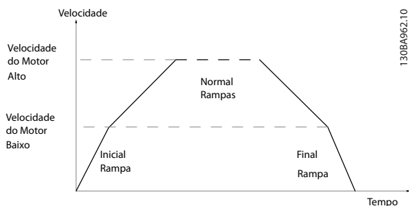
130BA962.10 Ilustração 3.19 Tempo de Rampa Inicial e Final
