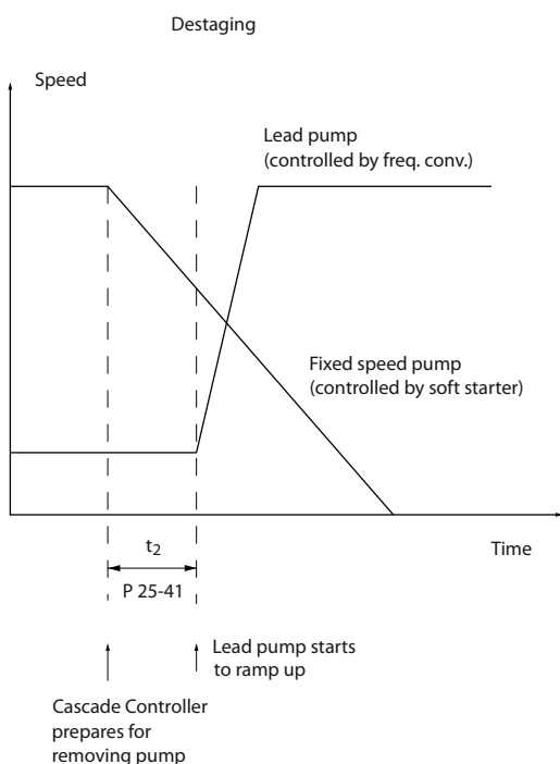
Ilustração 3.81 Desescalamento
