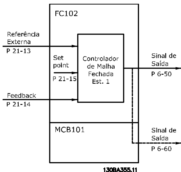
Ilustração 3.53 Feedback/Ref. de Malha Fechada 1
