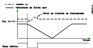
Ilustração 3.45 Desaceleração Controlada - Falha de rede elétrica de curta duração. Desaceleração para parada seguida por aceleração até a referência
