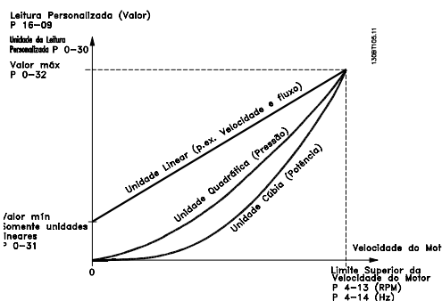
Ilustração 3.3 Leitura Personalizada
