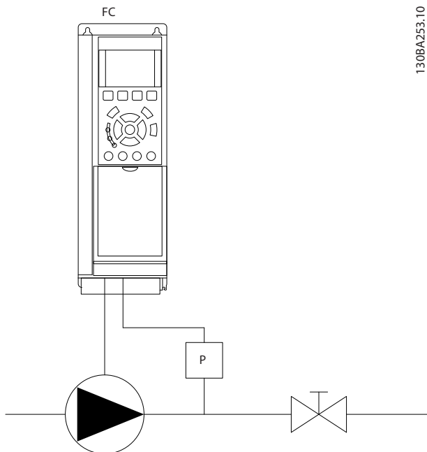
Ilustração 3.55 Esquema de Detecção de Fluxo Zero
