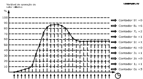
Ilustração 3.69 Tempo e valores relativos
