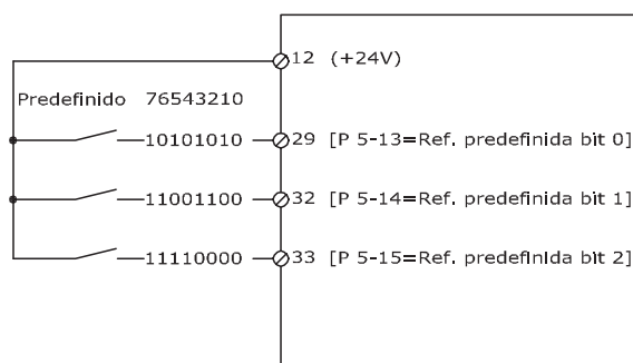
Ilustração 3.14 Esquema de Referência Predefinida
