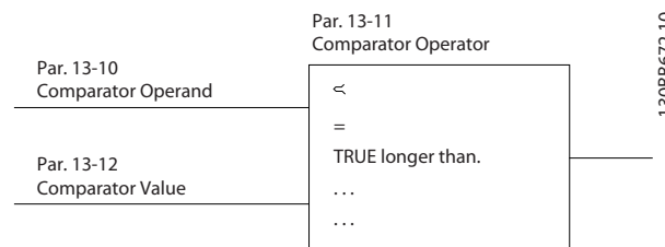
Ilustração 3.37 Comparadores
