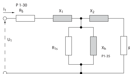
Ilustração 3.4 Diagrama Equivalente de Motor para um Motor Assíncrono
