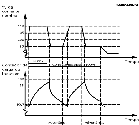
Ilustração 3.44 Corrente de Saída em Condição de Sobrecarga
