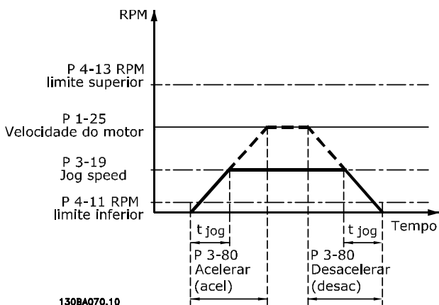
130BA070.10 Ilustração 3.18 Tempo de Rampa do Jog
