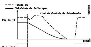
Ilustração 3.46 Desaceleração Controlada, falha de rede elétrica mais longa. Desaceleração enquanto a energia no sistema permitir, em seguida o motor é parado por inércia
