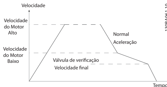
130BA961.10 Ilustração 3.20 Rampa da Válvula de Retenção
