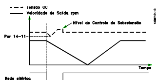
Ilustração 3.39 Desaceleração Controlada - Falha de rede elétrica de curta duração. Desaceleração para parada seguida por aceleração até a referência
