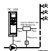
Ilustração 3.59 Sistema com Feedback de Pressão
