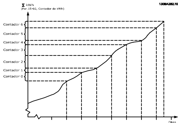
Ilustração 3.66 Gráfico do registro de energia
