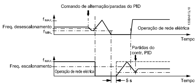
Ilustração 3.85 Configuração Lento
