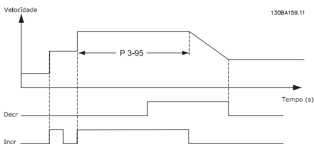
Ilustração 3.22 Atraso de Rampa Caso 2
