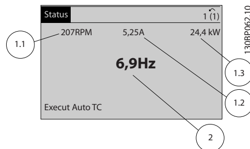
Ilustração 2.11 Tela de status II
