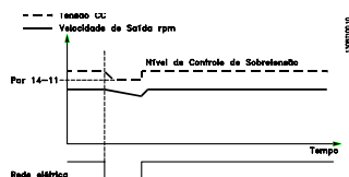
Ilustração 3.41 Backup Cinético, falha de rede elétrica de curta duração.
