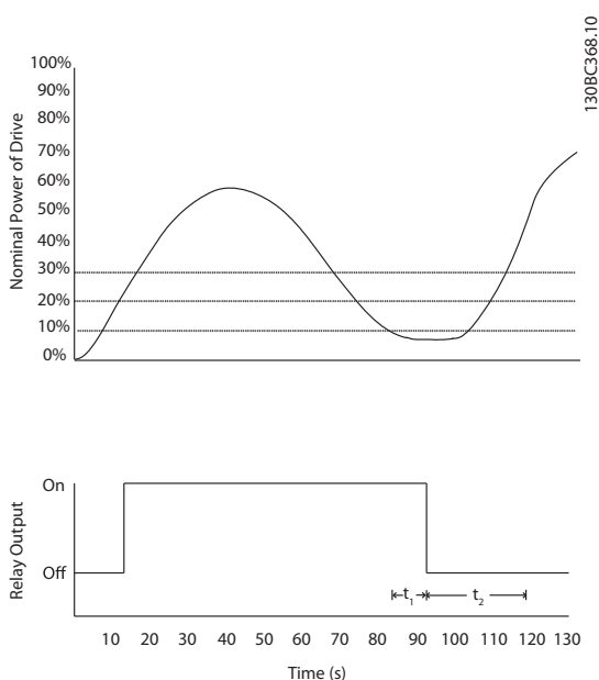
Ilustração 3.29 Exemplo da Função de Saída
