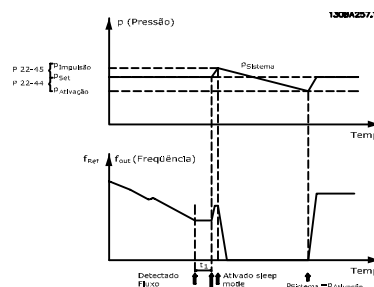
Ilustração 3.58 Sistema de Impulso com Feedback de Pressão
