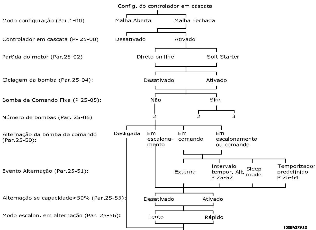
Ilustração 3.71 Setup da amostra do controlador em cascata
