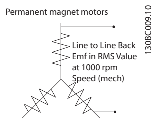
Ilustração 3.7 Definições de parâmetros da máquina da Força Contra Eletro Motriz de motores de ímã permanente
