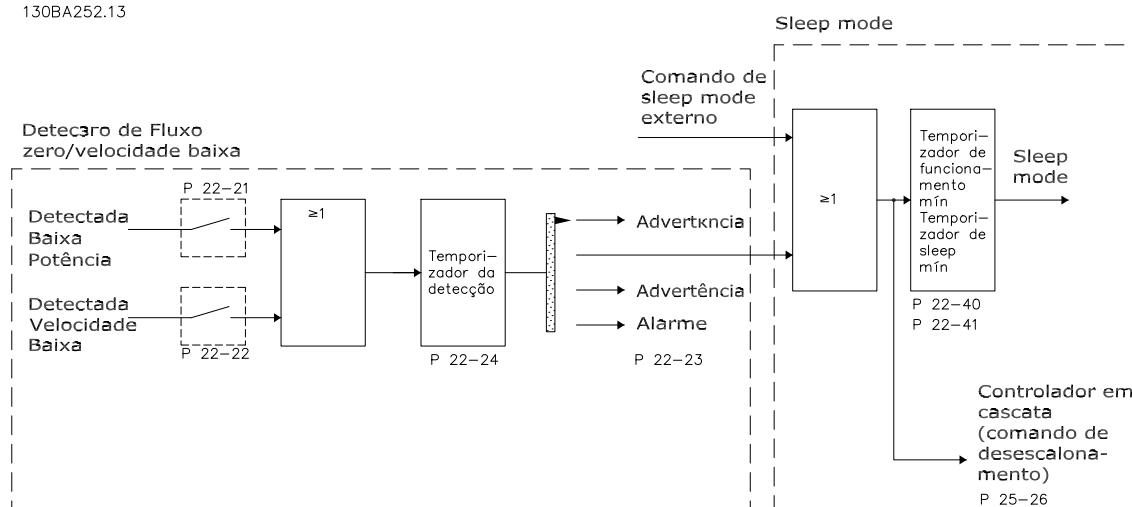
Ilustração 3.54 Fluxograma do Sinal
