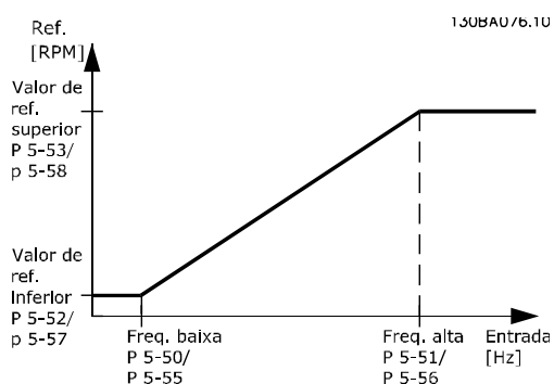
Ilustração 3.27 Entrada de Pulso
