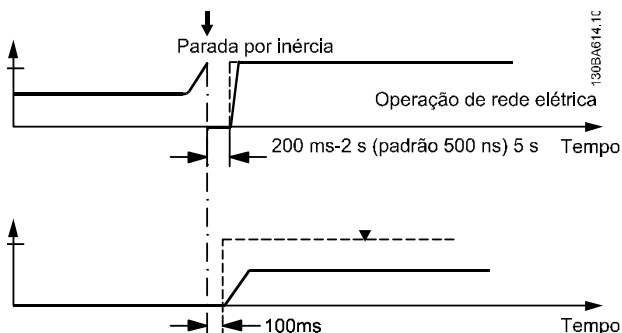
Ilustração 3.86 Configuração Rápido
