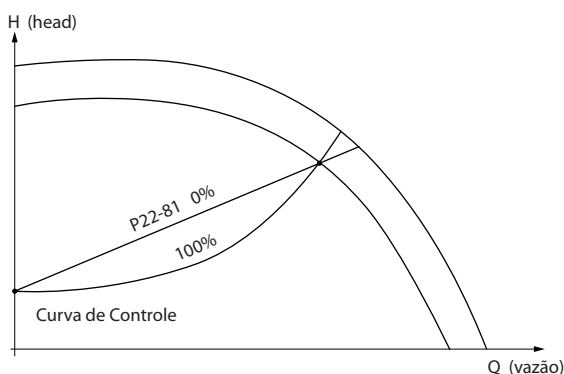
Ilustração 3.62 Curva de Aproximação Quadrático-Linear
