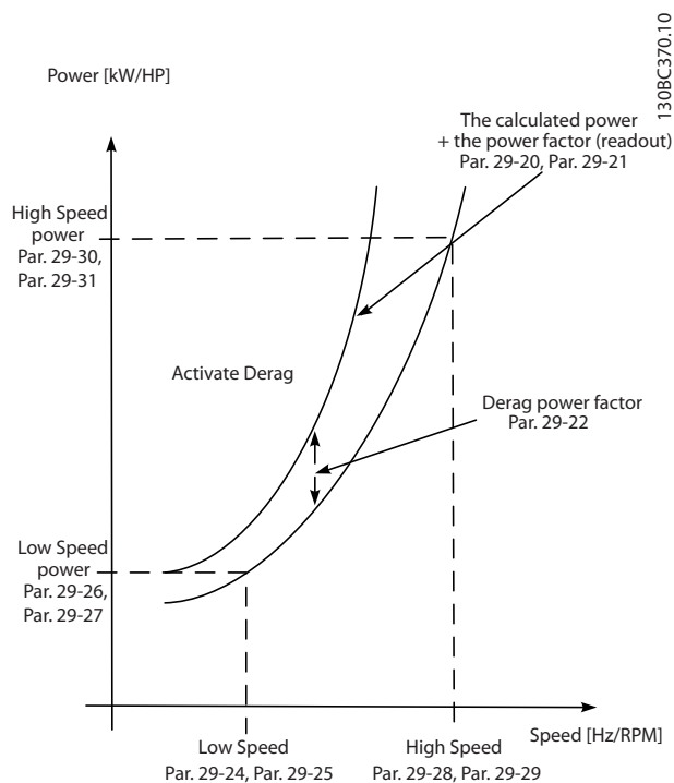
Ilustração 3.90 Sintonização da Potência de Derag
