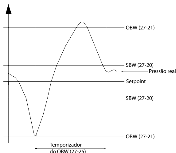
Ilustração 3.78 Tempo da OBW
