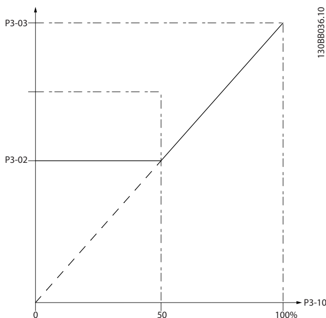
Ilustração 3.13 Referência Predefinida
