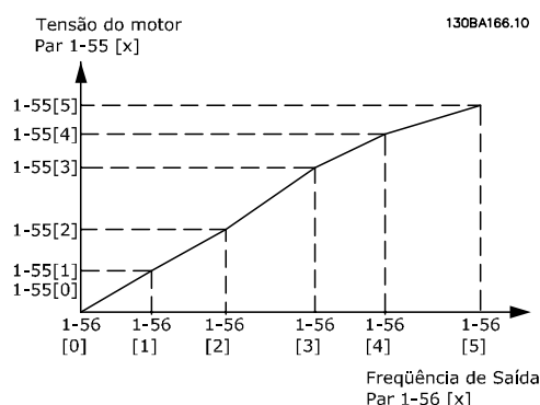
Ilustração 3.9 Característica U/f
