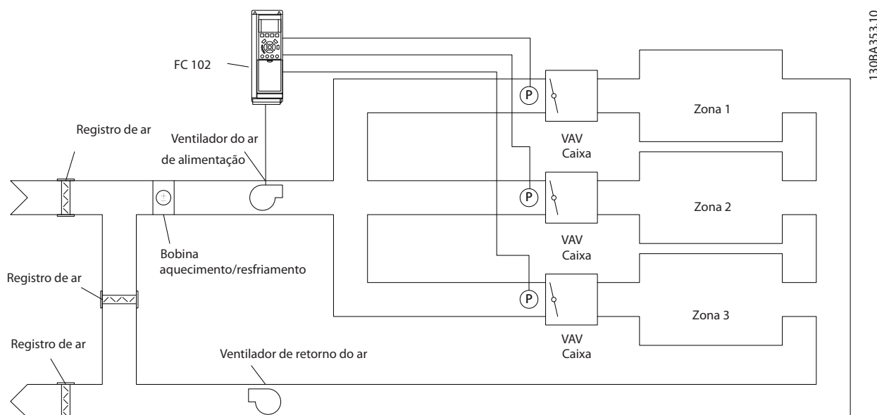
Ilustração 3.52 Esquema de Aplicação Multizonas
