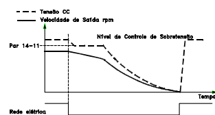
Ilustração 3.42 Backup Cinético, falha de rede elétrica mais longa.
