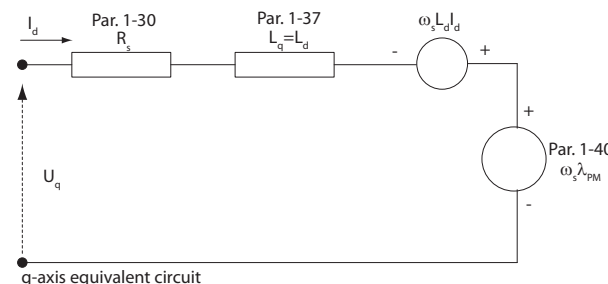
Ilustração 3.5 Diagrama de Circuito Equivalente de Motor para um motor PM não saliente
