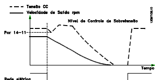
Ilustração 3.40 Desaceleração Controlada, falha de rede elétrica mais longa. Desaceleração enquanto a energia no sistema permitir, em seguida o motor é parado por inércia
