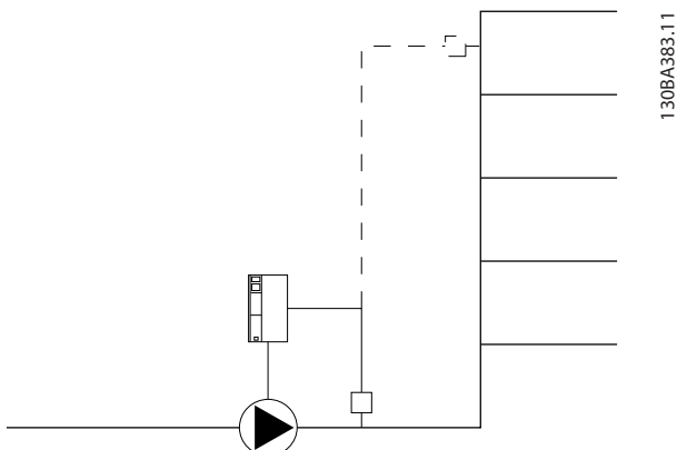
Ilustração 3.61 Setup de Compensação de Fluxo
