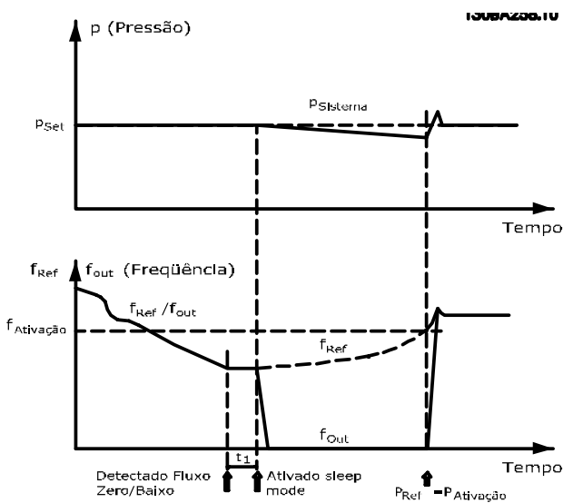
Ilustração 3.60 Sistema de Impulso sem Feedback de Pressão
