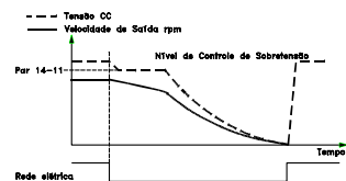
Ilustração 3.48 Backup Cinético, falha de rede elétrica mais longa.
