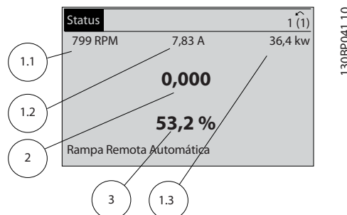
Ilustração 2.10 Tela de Status I
