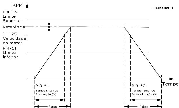
Ilustração 3.17 Rampa 1
