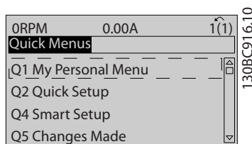
Ilustração 2.13 Quick Menus
