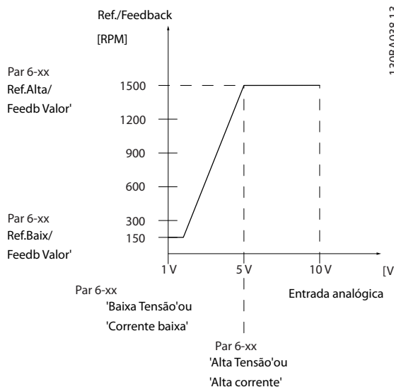
Ilustração 3.30 Condições de Live Zero
