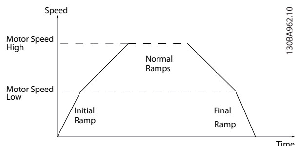
图 3.19 初始和最终加减速时间
