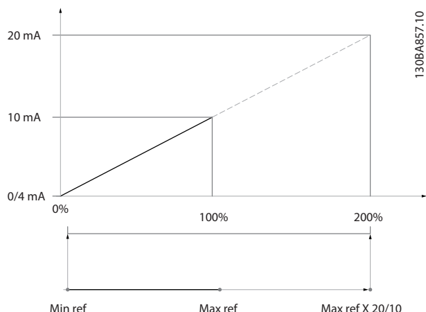
图 3.35 例 3
