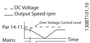
图 3.45 受控减速 - 主电源短时间故障。减速直到停止，接着减速到参考值。
