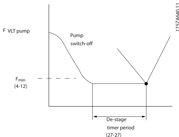
图 3.79 停止功能时间
