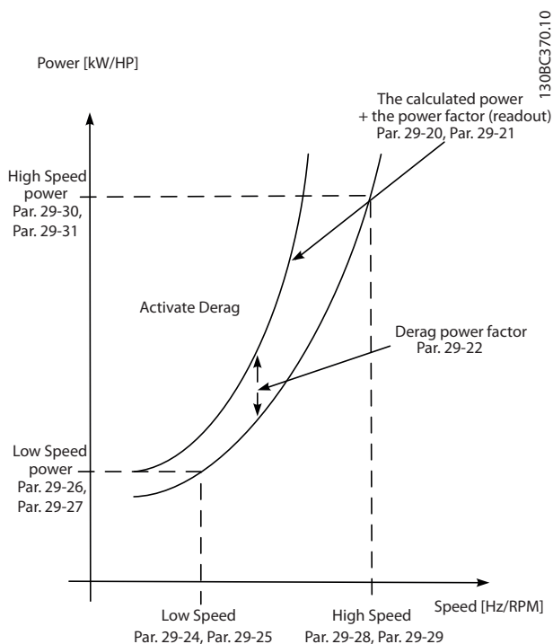
图 3.90 除屑功率调整
