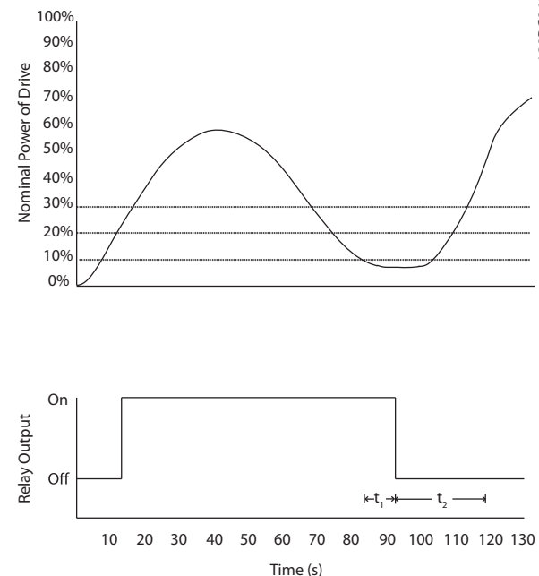
图 3.29 输出功能的示例
