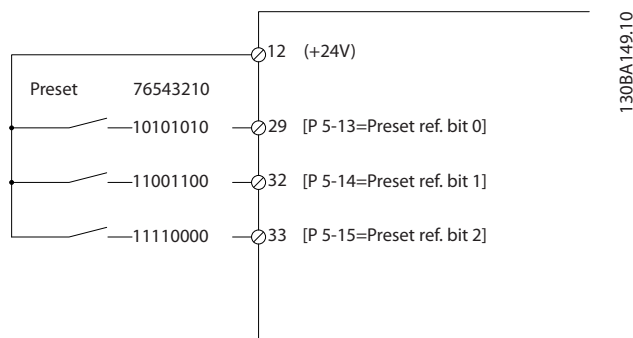
图 3.14 预置参考值方案
