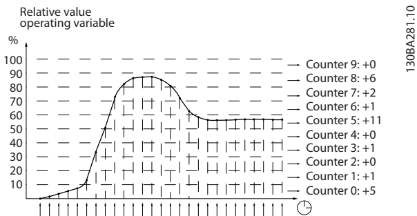
图 3.69 时间和相对值
