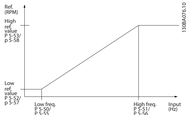
图 3.27 脉冲输入
