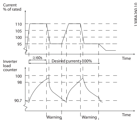
图 3.44 过载条件下的输出电流
