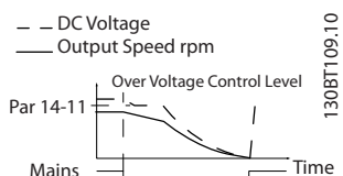
图 3.42 借能运行 - 主电源长时间故障。 一旦系统中的能量过低，电动机就会惯性停车。
