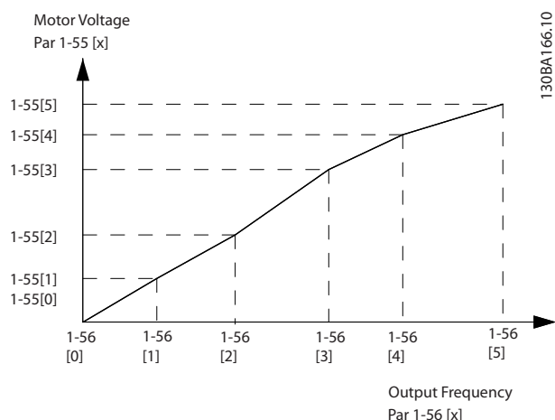
图 3.9 U/f 特性
