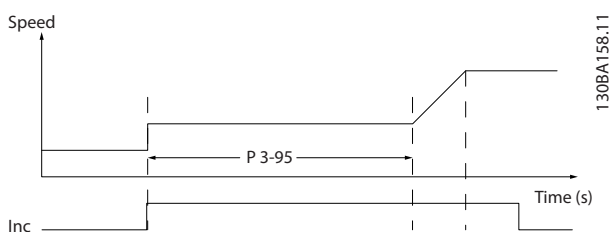
图 3.21 加减速延迟情况 1
