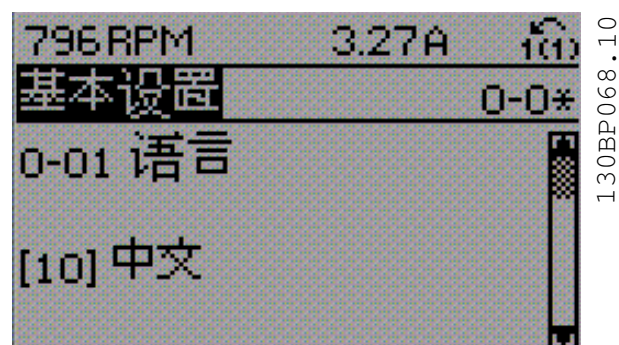
图 2.16 更改文本值
