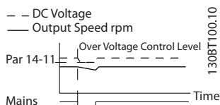
图 3.47 借能运行 - 主电源短时间故障。只要系统中的能量允许，便保持运行。
