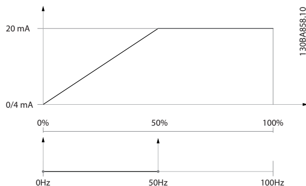
图 3.33 例 1
