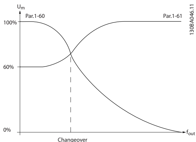
图 3.10 低速负载补偿
