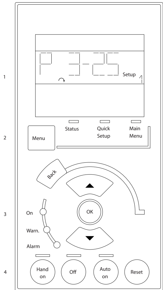
图 2.21 LCP 键
