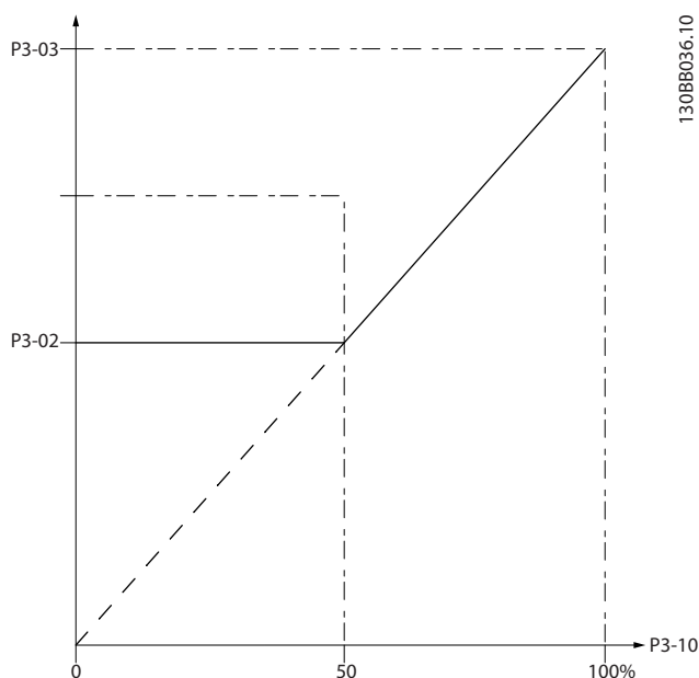
图 3.13 预置参考值
