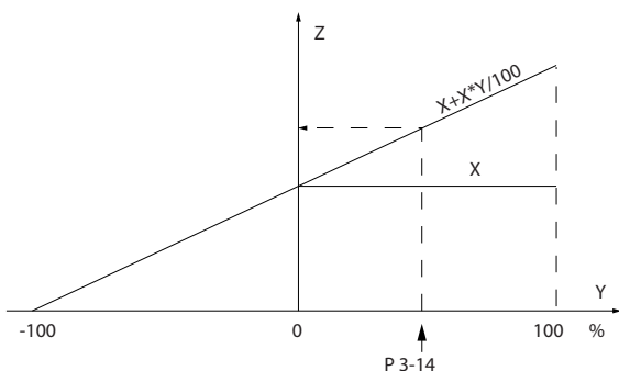
图 3.16 实际参考值
