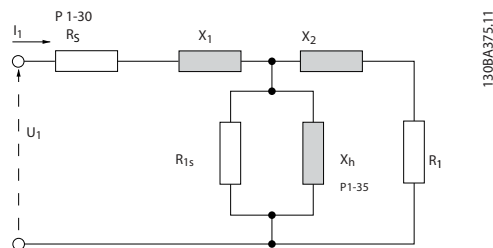
图 3.4 异步电动机的电动机当量图
