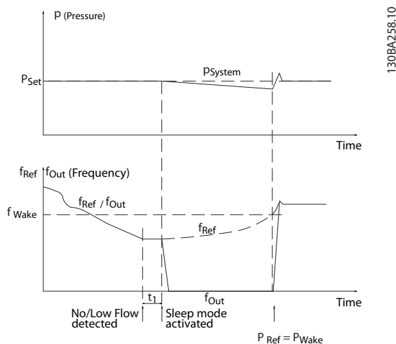
图 3.60 无压力反馈的放大系统
