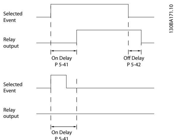
图 3.25 继电器打开延时
