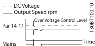
图 3.41 借能运行 - 主电源短时间故障。 只要系统中的能量允许，便保持运行。
