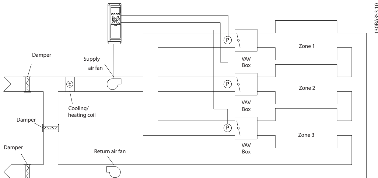
图 3.52 多区域应用方案
