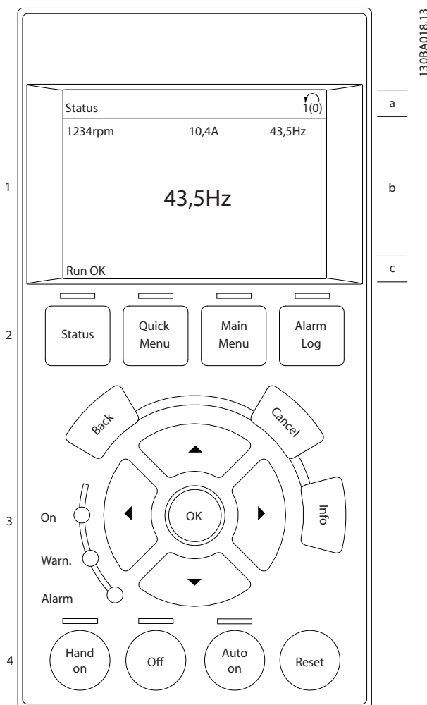
图 2.1 控制面板 (LCP)
