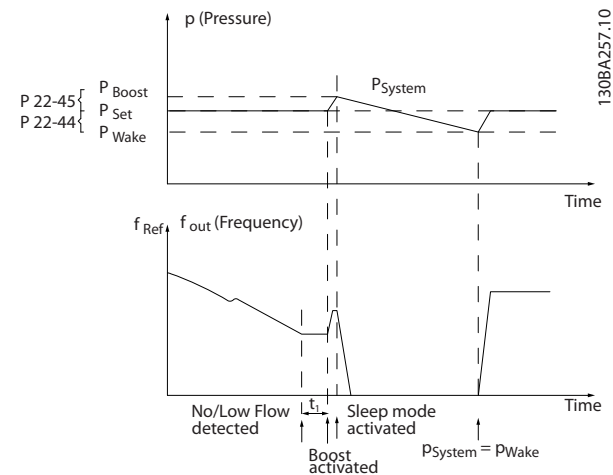
图 3.58 带有压力反馈的放大系统
