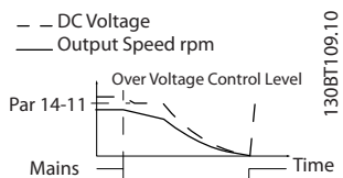
图 3.48 借能运行 - 主电源长时间故障。一旦系统中的能量过低，电动机就会惯性停车。
