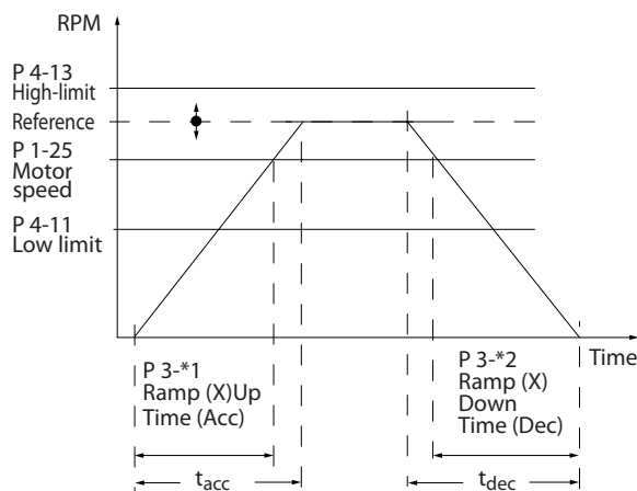
图 3.17 加减速 1
