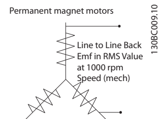
图 3.7 设备参数中关于永磁电动机的反电动势定义
