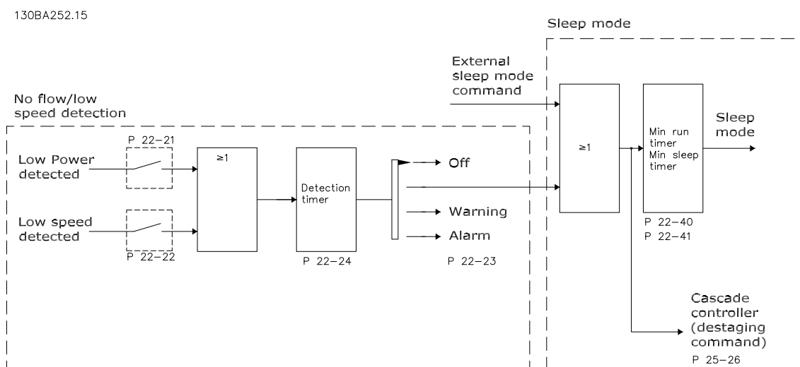
图 3.54 信号流程图
