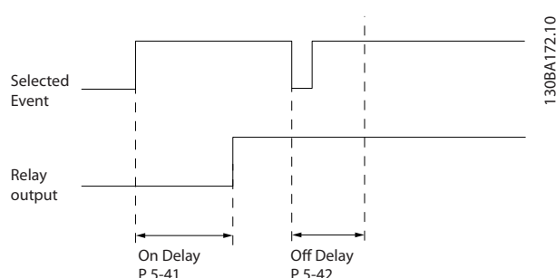
图 3.26 继电器关闭延迟
