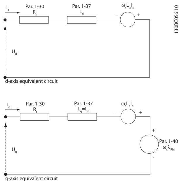
图 3.5 PM 非突出电动机的电动机当量图
