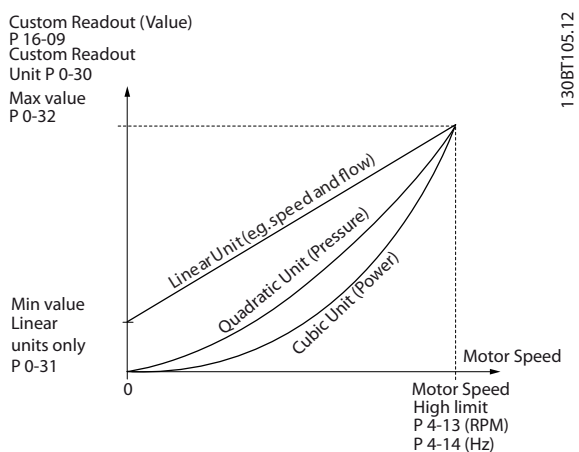
图 3.3 自定义读数
