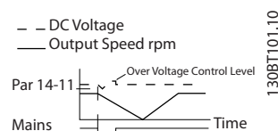
图 3.39 受控减速 - 主电源短时间故障。减速直到停止,接着减速到参考值。
