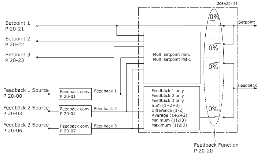
图 3.51 闭环 PID 控制器中的输入信号
