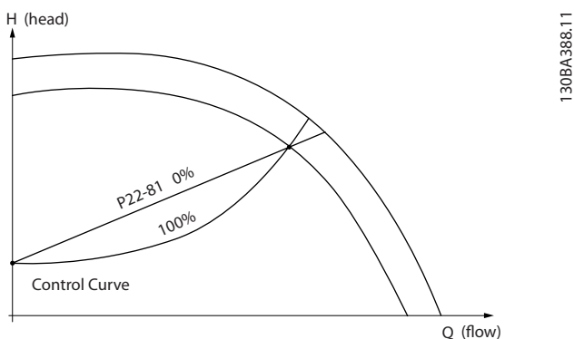
图 3.62 平方-线性曲线近似
