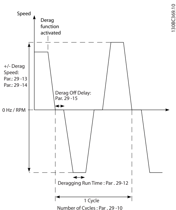
图 3.89 除屑功能
