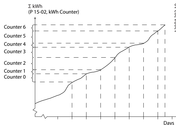
图 3.66 能量记录图
