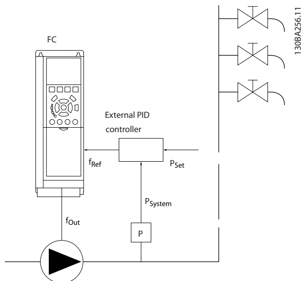
图 3.59 带有压力反馈的系统
