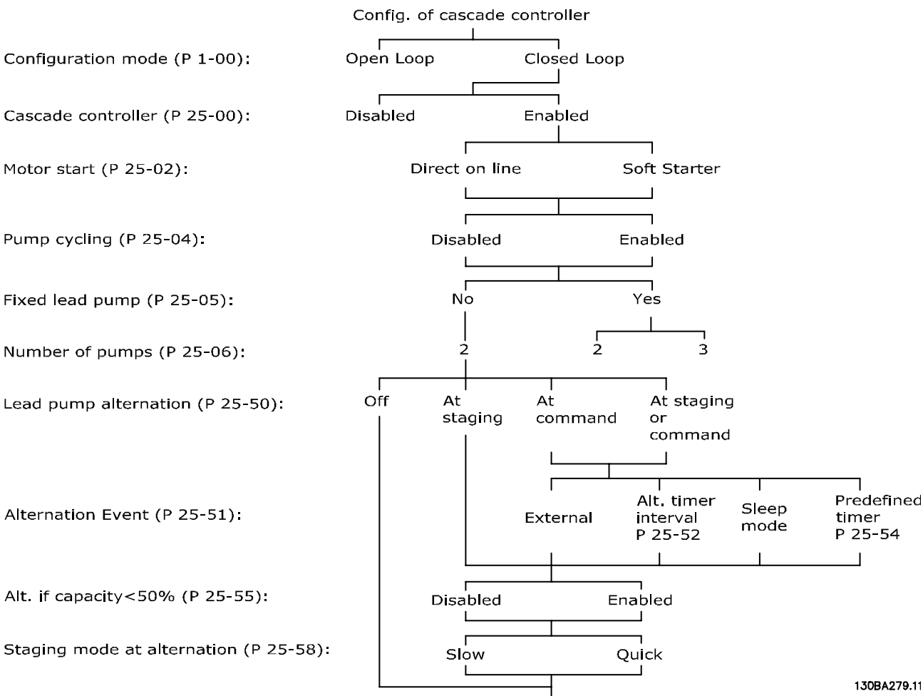
图 3.71 多泵控制器示例设置
