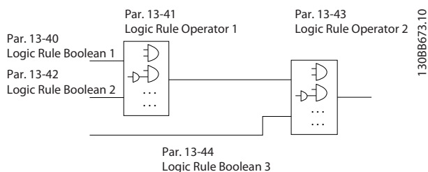
图 3.38 逻辑规则
