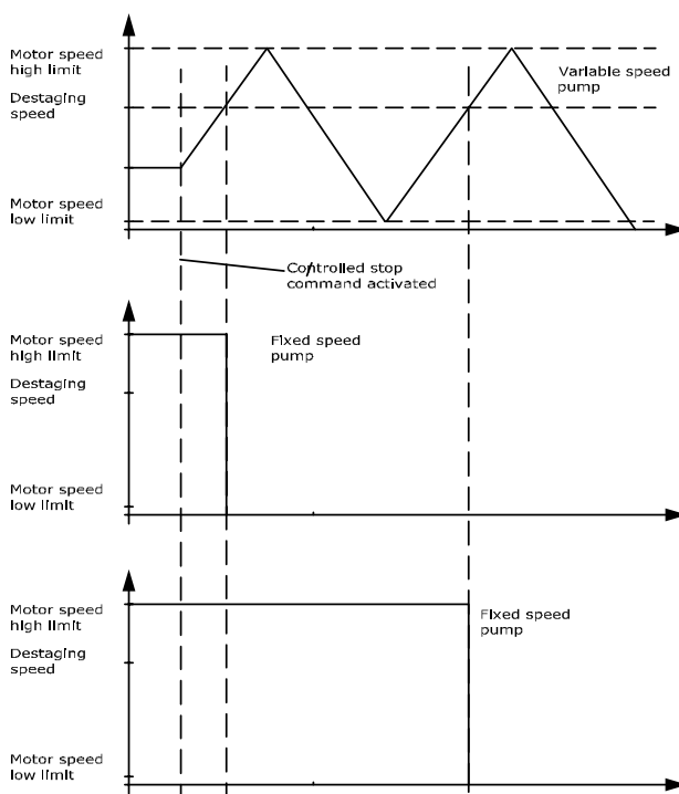
图 3.84 停止速度
