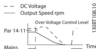
图 3.40 受控减速 - 主电源长时间故障。只要系统中的能量允许,便进行减速,之后电动机将惯性停车。
