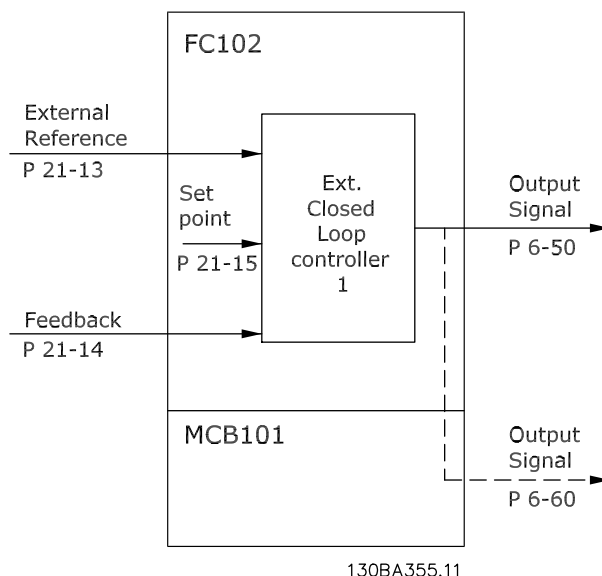
图 3.53 闭环 1 参考值/反馈
