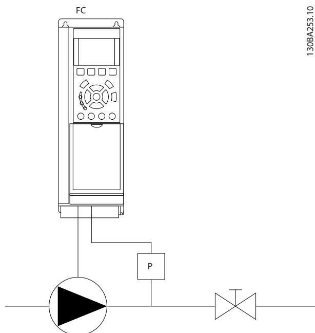
图 3.55 无流量检测方案
