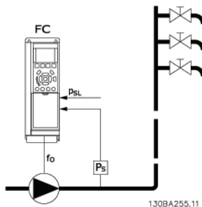
图 3. 57 图例: FC=变频器; fo=频率输出; Ps=P system; Psl=P setpoint
