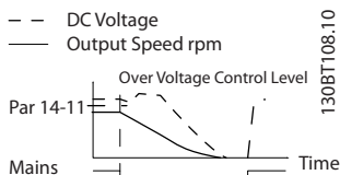
图 3.46 受控减速 - 主电源长时间故障。只要系统中的能量允许，便进行减速，之后电动机将惯性停车。
