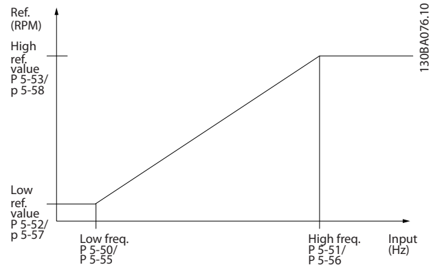
Рисунок 3.27 Импульсный вход
