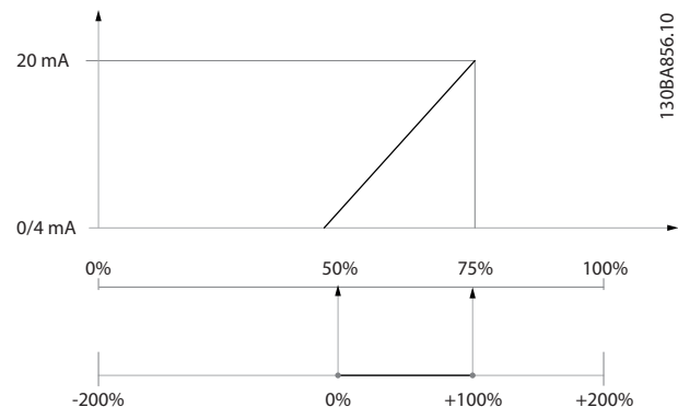
Рисунок 3.34 Пример 2
