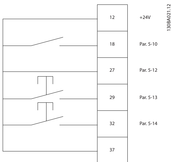
Рисунок 1.8 Увеличение/снижение скорости
