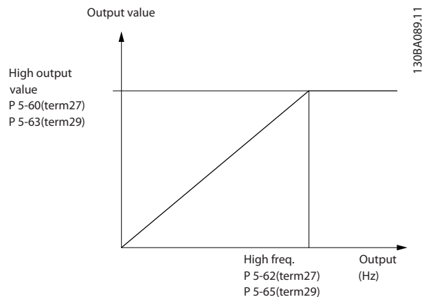
Рисунок 3.28 Импульсный выход
