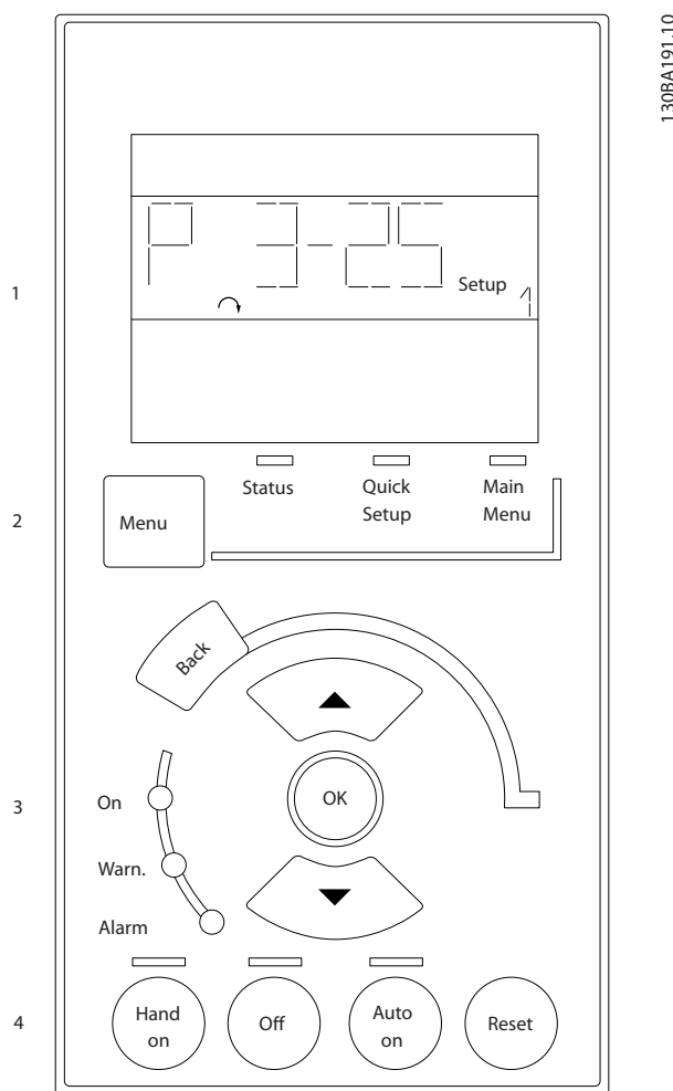
Рисунок 2.21 Кнопки LCP
