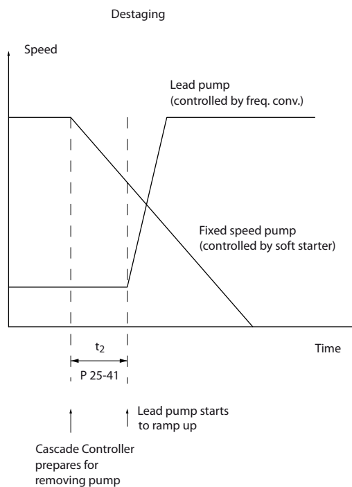
Рисунок 3.77 Выключение
