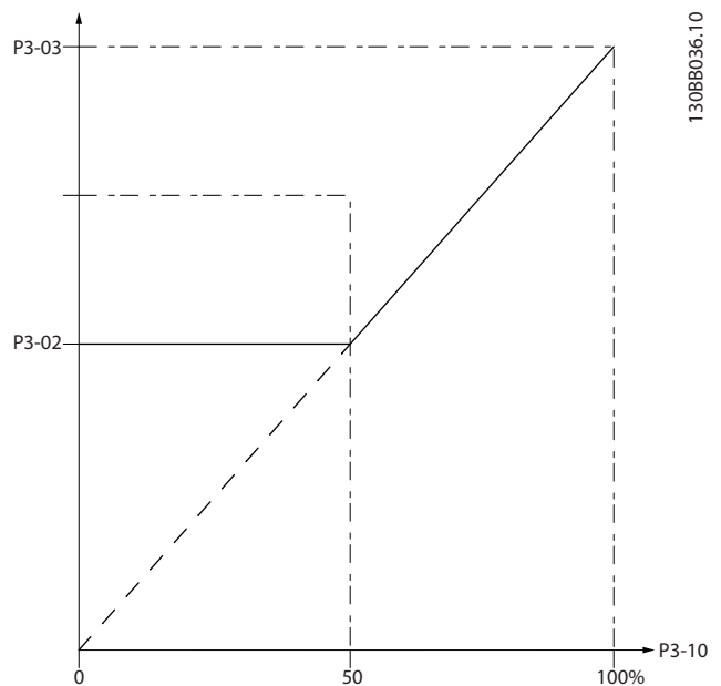
Рисунок 3.13 Предустановленное задание
