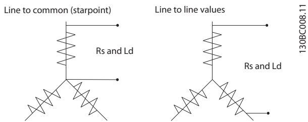
Рисунок 3.6 Параметры двигателя представлены в разных форматах. Преобразователи частоты Danfoss всегда требуют использования значения между линией и общей точкой
