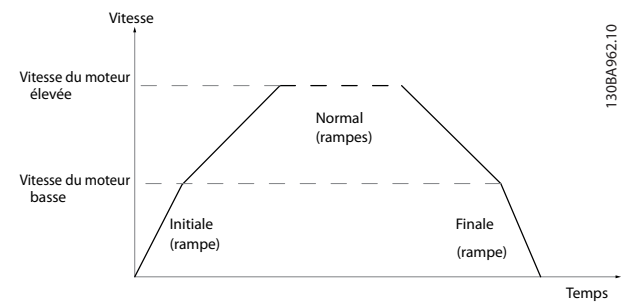
Illustration 3.19 Temps de rampe initial et final
