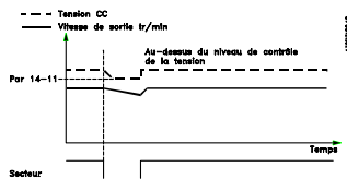
Illustration 3.43 Sauvegarde cinétique, brève panne de secteur. Fonctionnement tant que l'énergie du système le permet.
