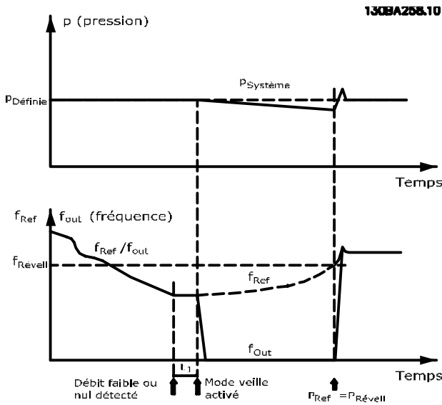
Illustration 3.58 Système de suralimentation sans retour de la pression
