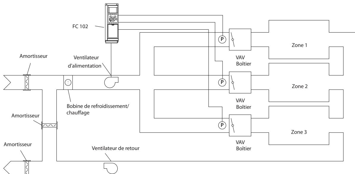
Illustration 3.50 Schéma d'application multizones
