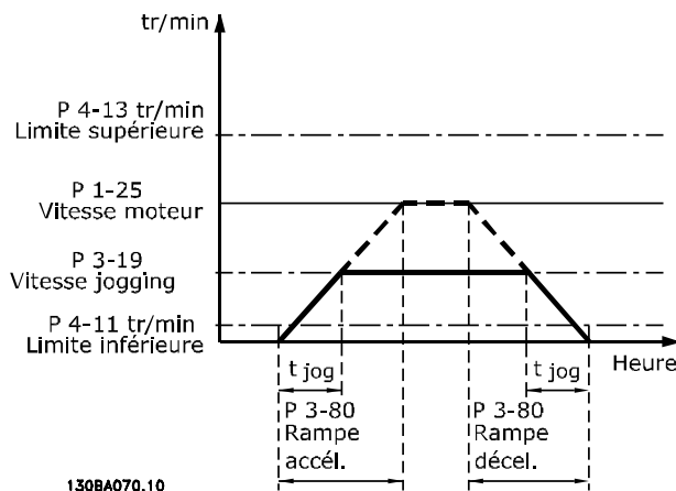
Illustration 3.18 Temps de la rampe de jogging
