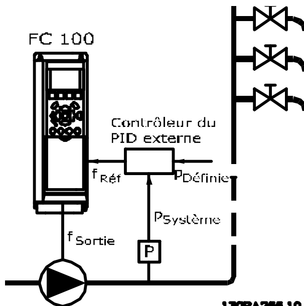
Illustration 3.57 Système avec retour de la pression
