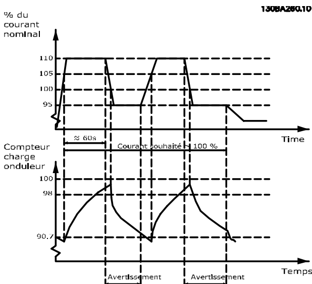
Illustration 3.46 Courant de sortie en condition de surcharge
