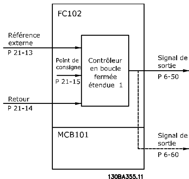
Illustration 3.51 Réf/ret PID ét. 1
