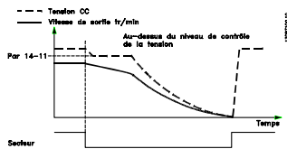
Illustration 3.44 Sauvegarde cinétique, panne secteur plus longue. Le moteur est en roue libre dès que l'énergie du système est trop basse.
