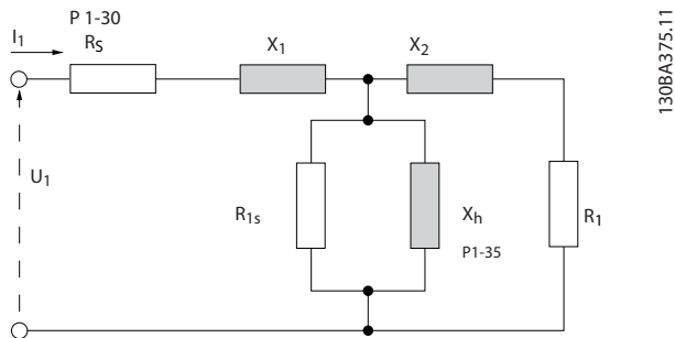
Illustration 3.4 Schéma moteur équivalent pour un moteur asynchrone
