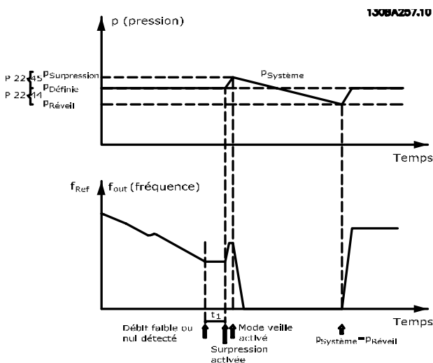
Illustration 3.56 Système de suralimentation avec retour de pression
