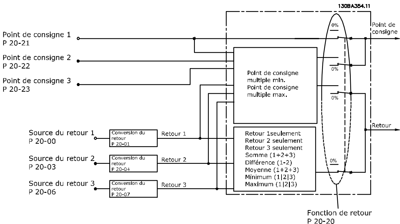
Illustration 3.49 Signaux d'entrée du régulateur PID en boucle fermée
