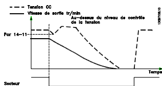
Illustration 3.42 Rampe de décélération ctrlée, défaut secteur plus long. Décélération tant que l'énergie du système le permet, puis mise en roue libre du moteur.
