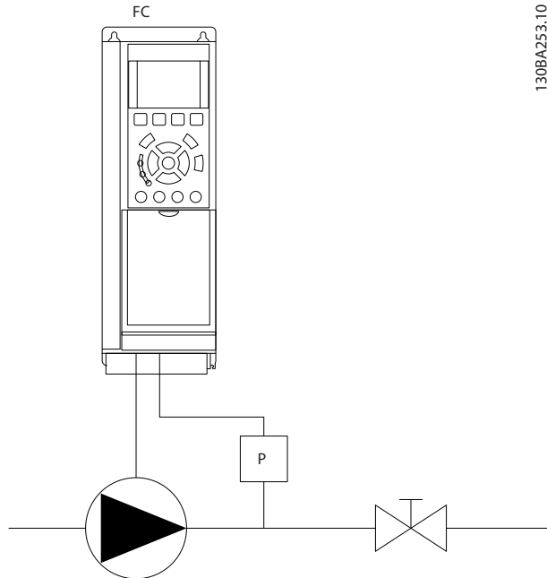
Illustration 3.53 Schéma de détection d'absence de débit
