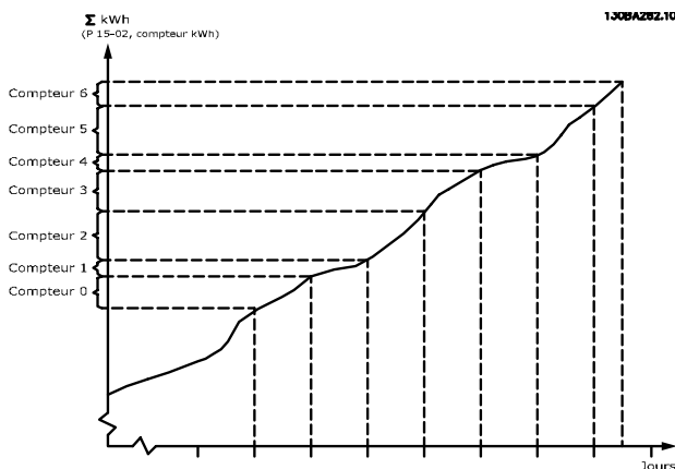
Illustration 3.64 Graphique du journal énergétique
