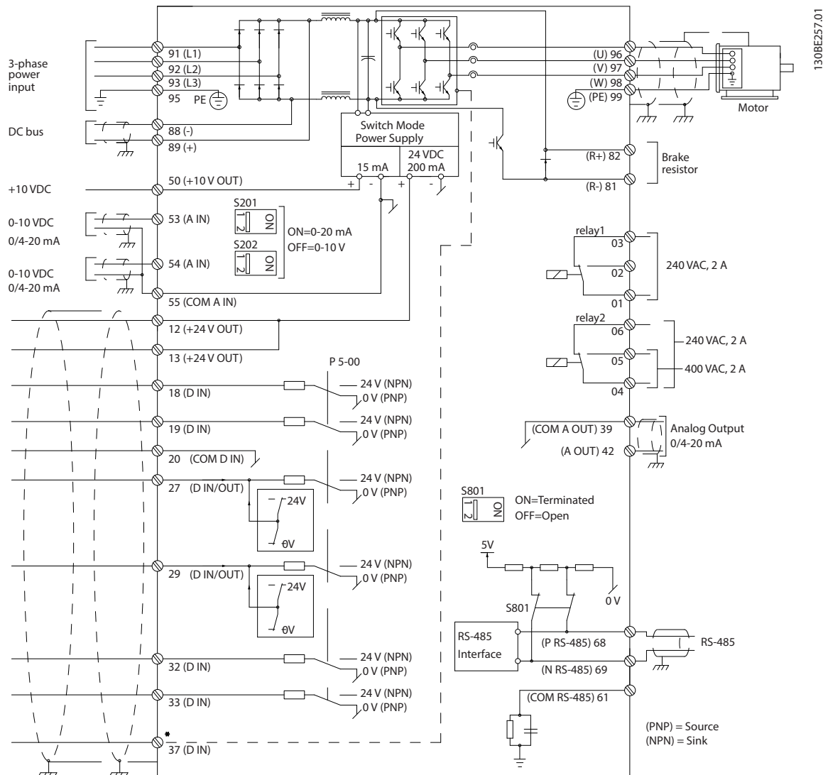
Illustration 1.2 Dessin schématique du câblage de base
