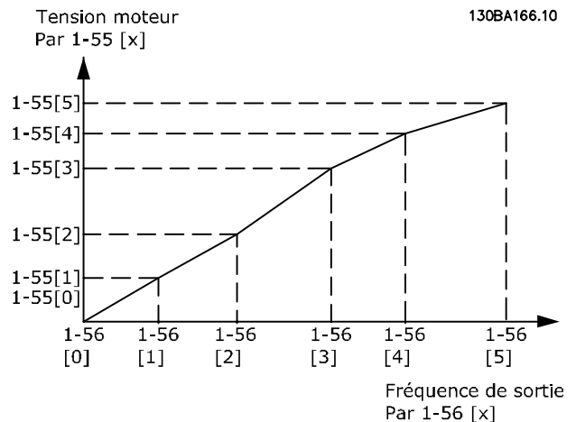
Illustration 3.9 Caractéristique U/f
