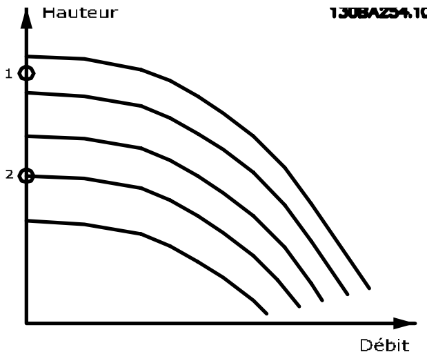
Illustration 3.54 Graphique de détection d'absence de débit
