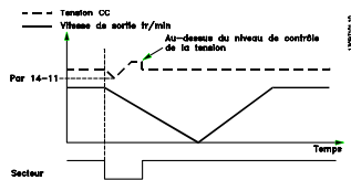
Illustration 3.41 Rampe de décélération ctrlée - Bref défaut secteur. Décélération jusqu'à l'arrêt, puis accélération jusqu'à la référence.
