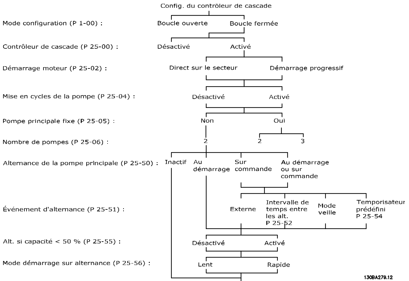
Illustration 3.68 Process de configuration du contrôleur de cascade
