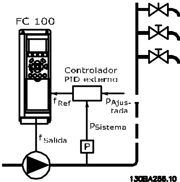
Ilustración 3.57 Sistema con realimentación de presión
