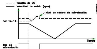
Ilustración 3.41 Rampa de deceleración controlada - fallo breve aliment. Rampa de desaceleración hasta parar seguida por una rampa de aceleración hasta la referencia.
