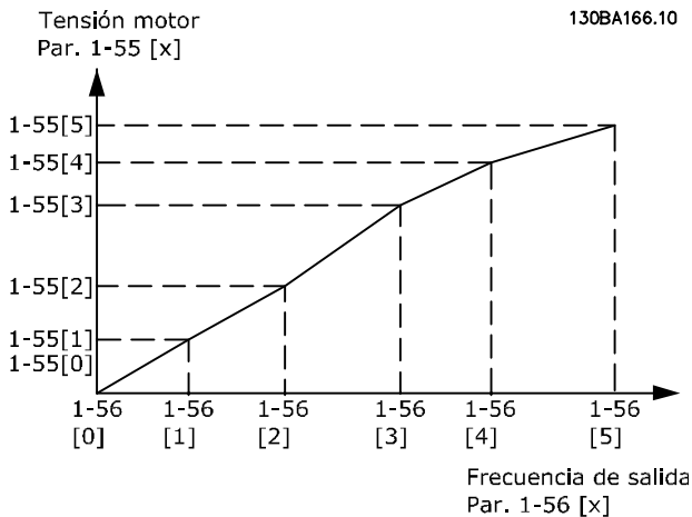
Ilustración 3.9 Característica u/f
