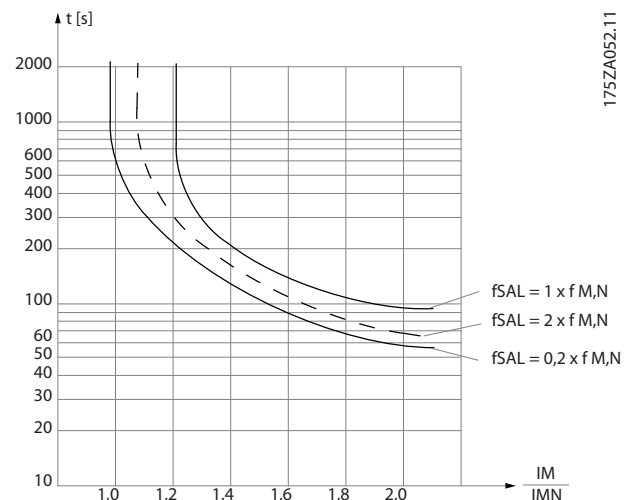
Ilustración 3.12 Protección de sobrecarga del motor
