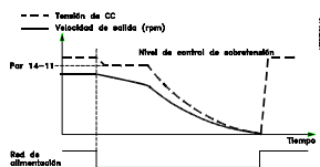
Ilustración 3.44 Energía regenerativa, fallo más largo de alimentación. El motor queda en inercia tan pronto como se detecte que la energía del sistema es demasiado baja.
