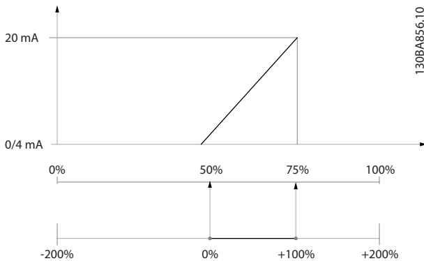
Ilustración 3.34 Ejemplo 2
