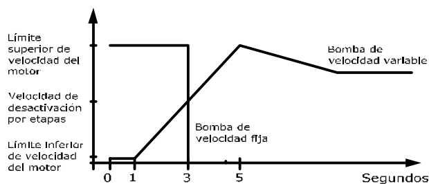
Ilustración 3.80 Umbral desconex. por etapas
