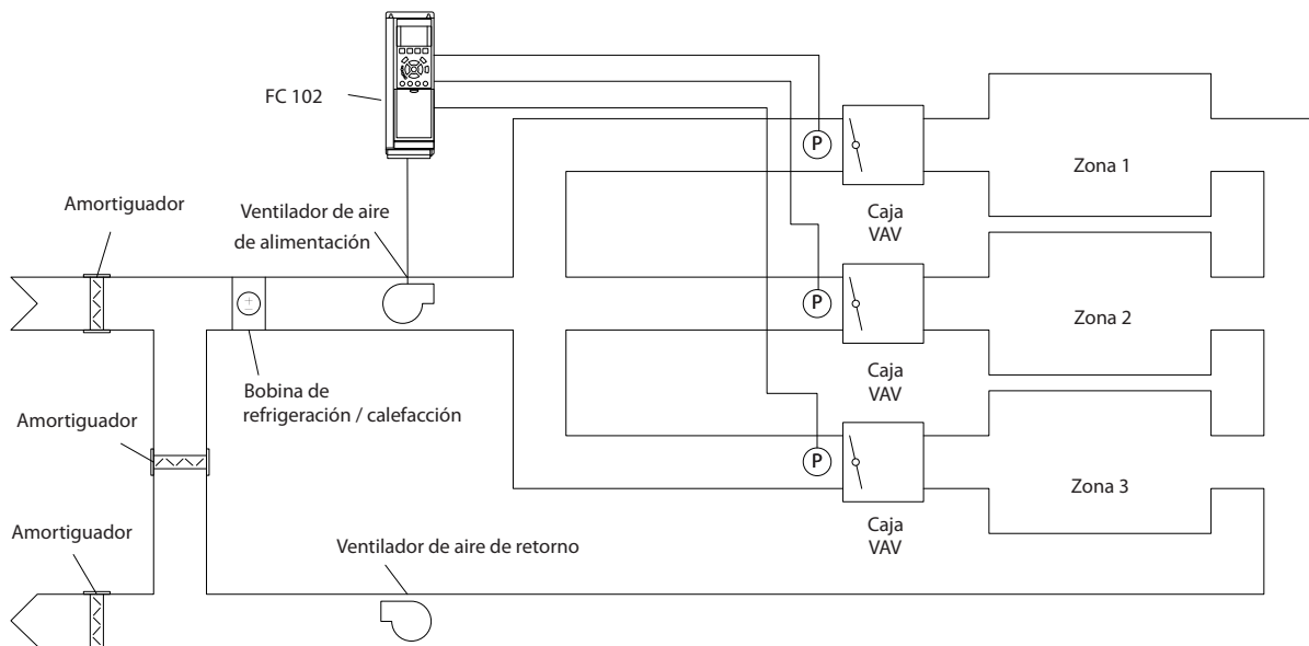
Ilustración 3.50 Esquema de aplicación multizona
