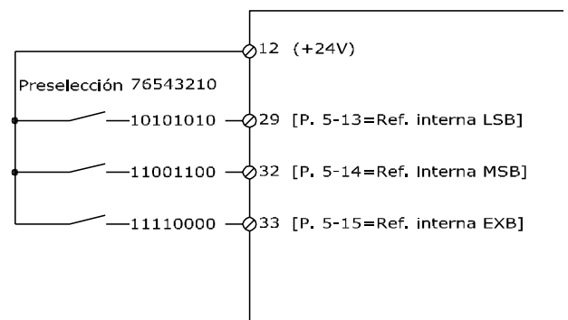
Ilustración 3.14 Esquema de referencia interna
