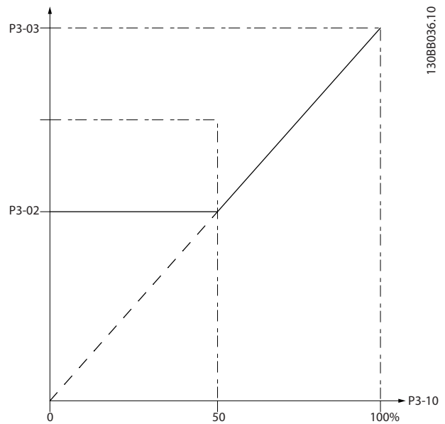
Ilustración 3.13 Referencia interna
