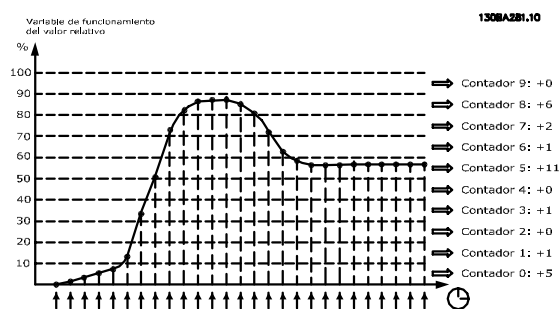
Ilustración 3.66 Tiempo y valores relativos
