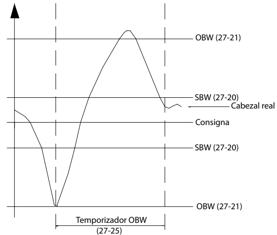
Ilustración 3.75 Tiempo OBW
