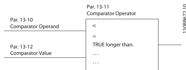
Ilustración 3.37 Comparadores
