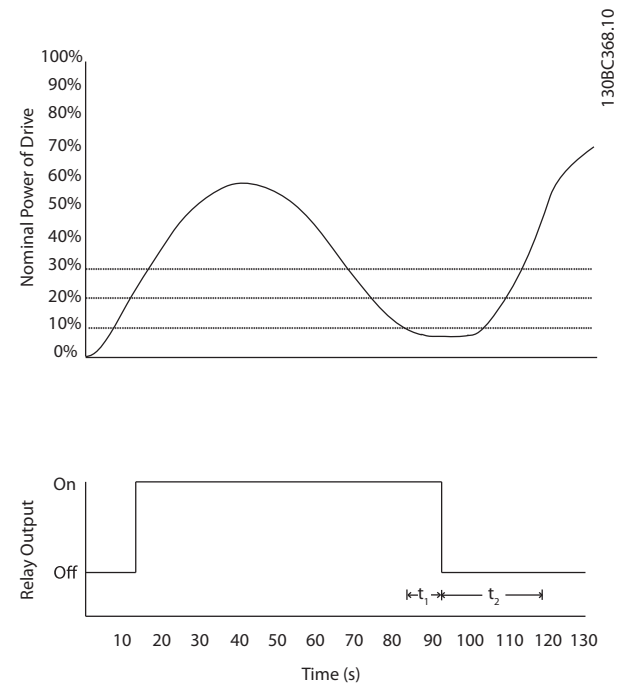
Ilustración 3.29 Ejemplo de la función de salida
