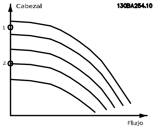
Ilustración 3.54 Gráfico de detección de falta de caudal
