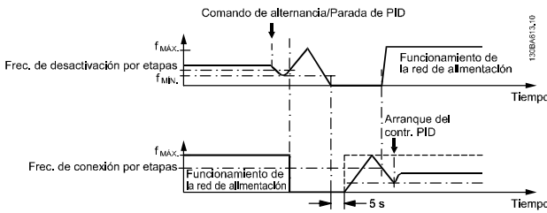
Ilustración 3.82 Configuración lenta
