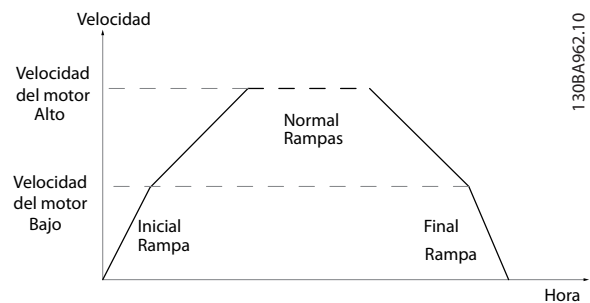
Ilustración 3.19 Tiempo de rampa inicial y final
