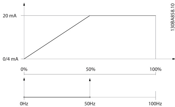
Ilustración 3.33 Ejemplo 1
