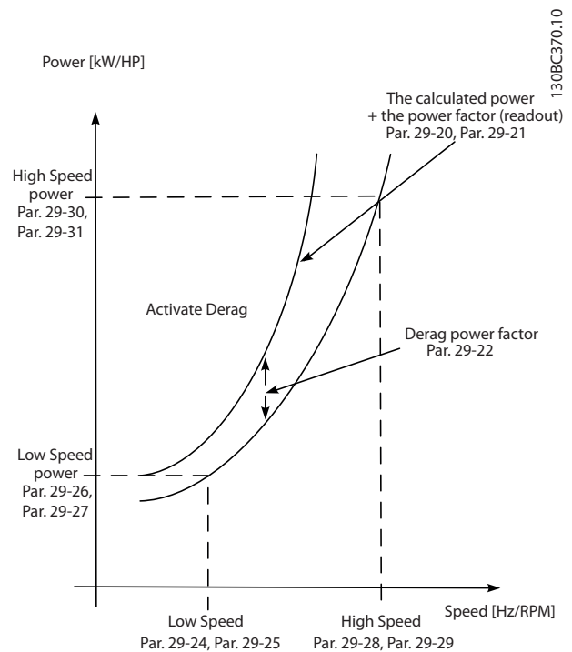
Ilustración 3.87 Ajuste de potencia de barrido
