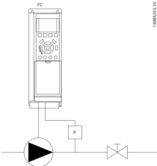
Ilustración 3.53 Esquema de detección de falta de caudal
