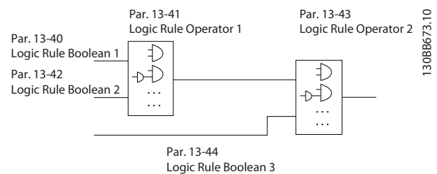
Ilustración 3.40 Reglas lógicas
