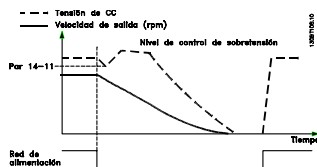
Ilustración 3.42 Rampa de deceleración controlada, fallo más largo de aliment. Rampa de desaceleración tan larga como lo permita la energía almacenada en el sistema, y luego motor a inercia.
