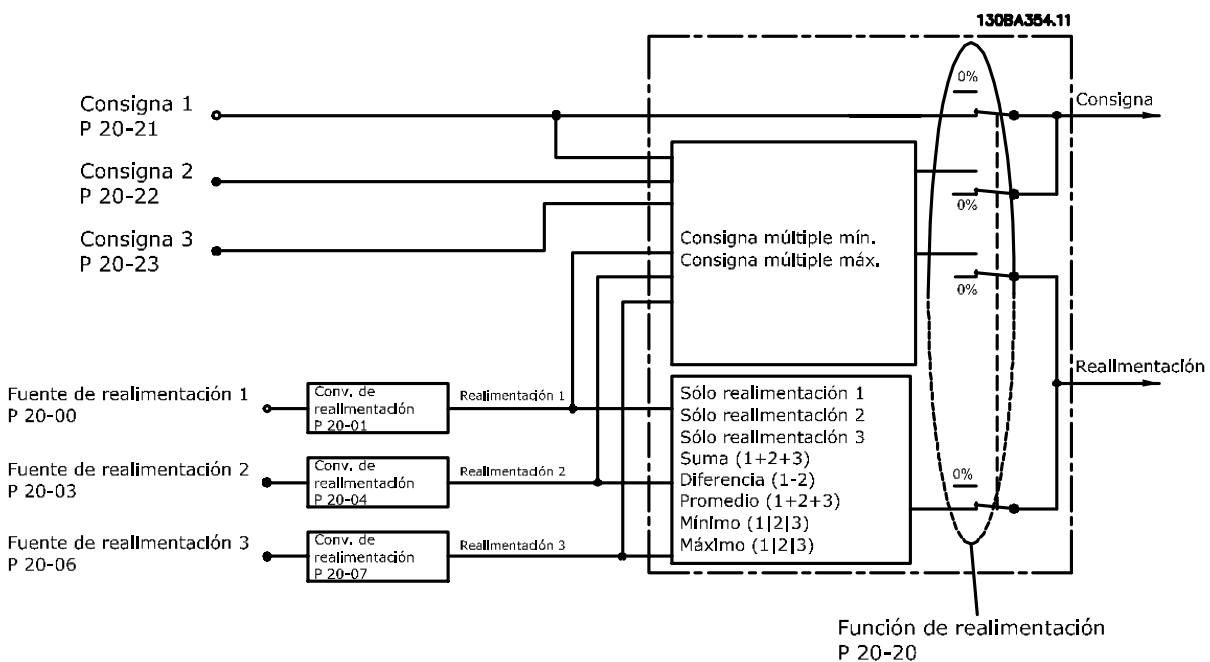
Ilustración 3.49 Señales de entrada en el controlador PID de lazo cerrado
