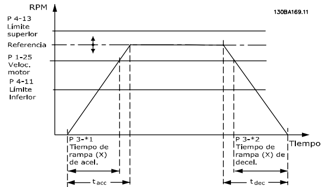
Ilustración 3.17 Rampa 1
