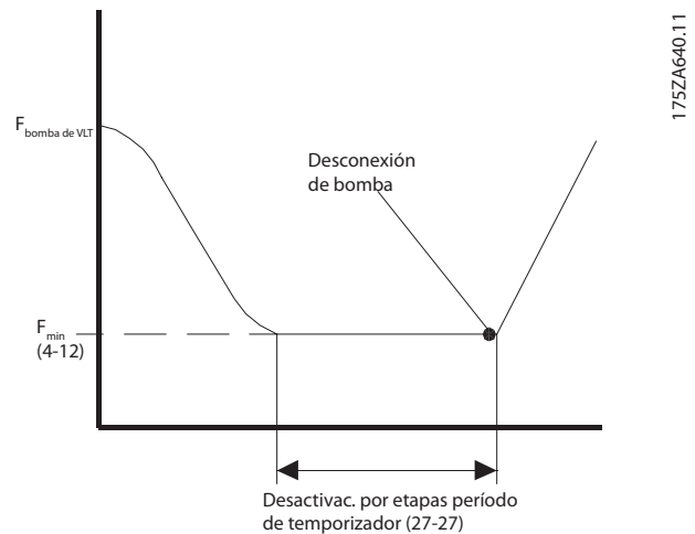
Ilustración 3.76 Tiempo función desactiv. por etapas
