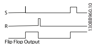
Ilustración 3.39 Salidas de Flip Flop
