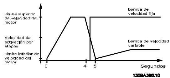
Ilustración 3.79 Umbral conex. por etapas
