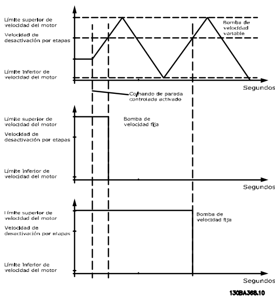
Ilustración 3.81 Veloc. desconex. por etapas
