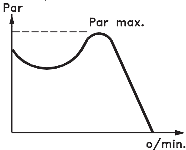
Ilustración 1.1 Par de arranque
