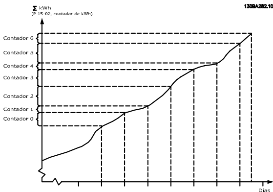
Ilustración 3.64 Gráfico de registro de energía
