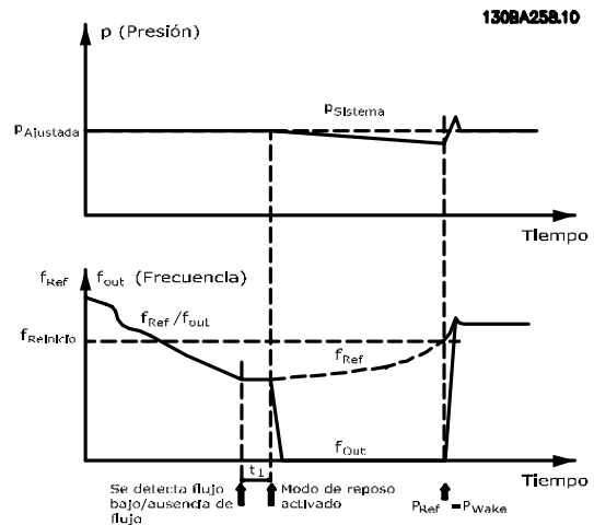
Ilustración 3.58 Sistema de refuerzo sin realimentación de presión
