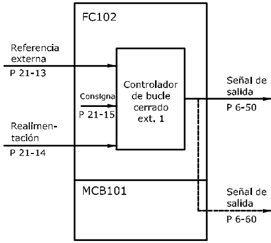
Ilustración 3.51 Ref. lazo cerrado 1/Realimentación
