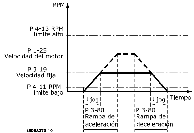
Ilustración 3.18 Tiempo rampa veloc. fija
