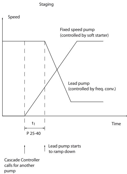
Ilustración 3.77 Conexión por etapas
