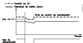
Ilustración 3.43 Energía regenerativa, fallo breve de aliment. Mantener tanto como lo permita la energía almacenada en el sistema.
