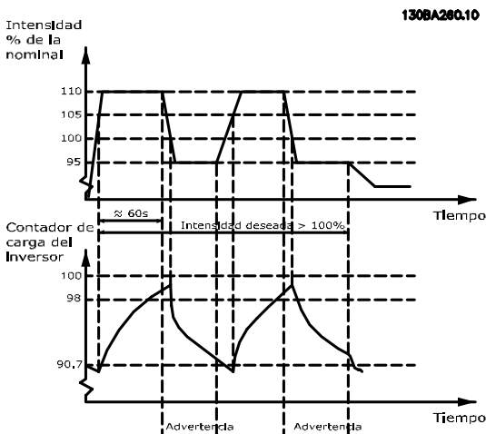
Ilustración 3.46 Intensidad de salida en condiciones de sobrecarga
