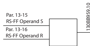
Ilustración 3.38 Flip Flops de Reset/Set
