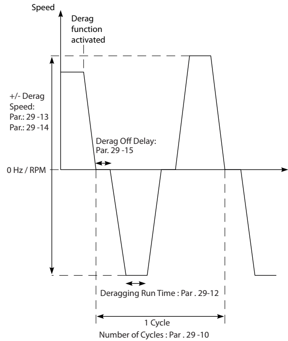
Ilustración 3.86 Función de barrido
