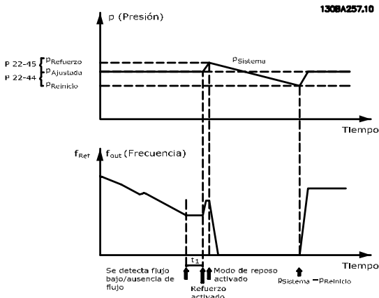
Ilustración 3.56 Sistema de refuerzo con realimentación de presión
