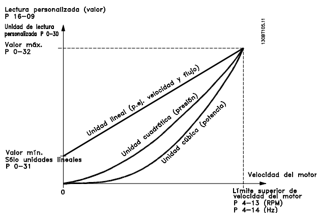
Ilustración 3.3 Lectura personalizada
