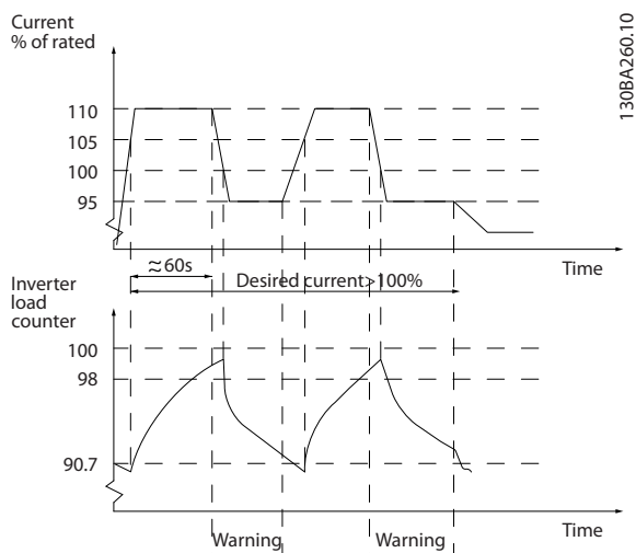
Рисунок 3.45 Выходной ток в условиях перегрузки
