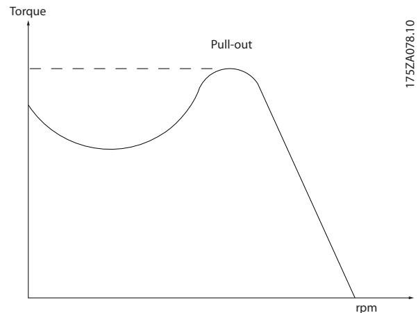
Рисунок 1.1 Момент опрокидывания
