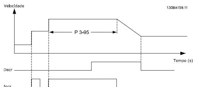
Ilustração 3.26 Atraso de Rampa Caso 2
