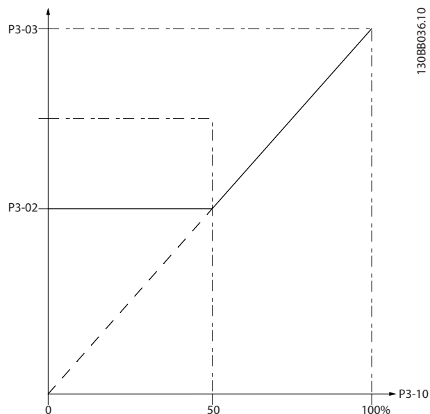
Ilustração 3.17 Referência predefinida
