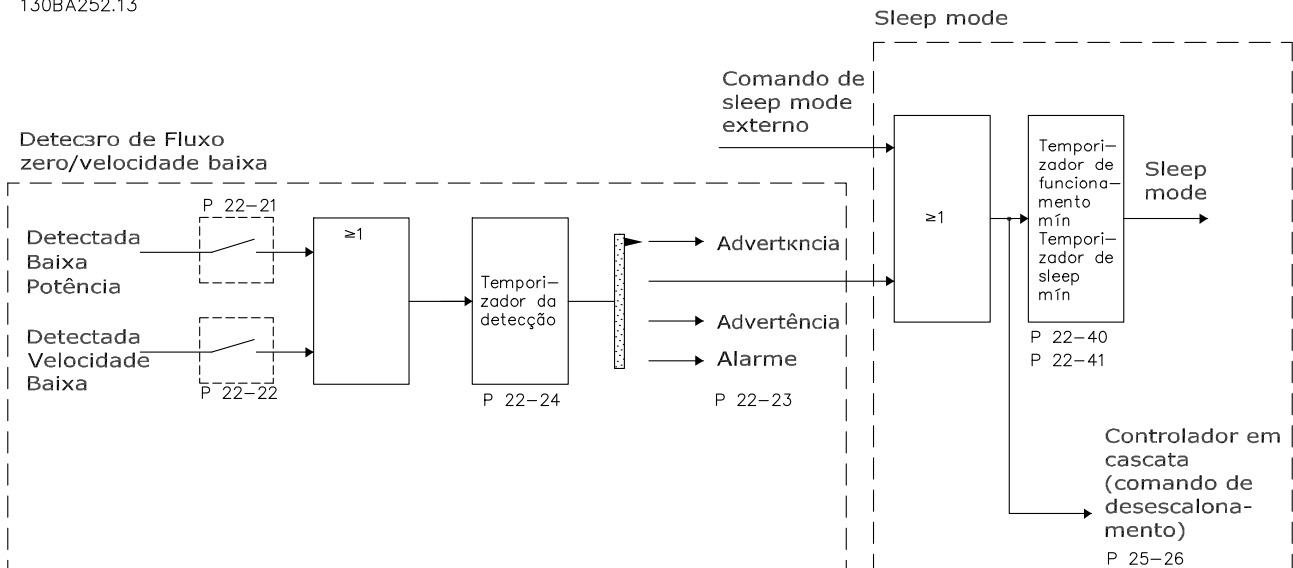
Ilustração 3.63 Fluxograma do sinal
