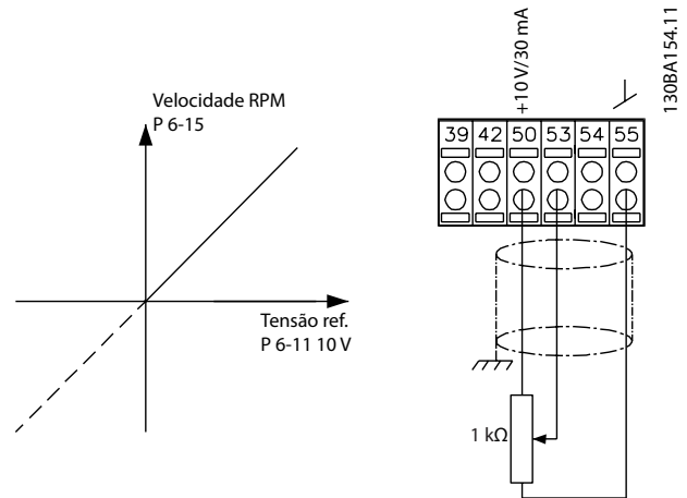
Ilustração 1.9 Referência do Potenciômetro
