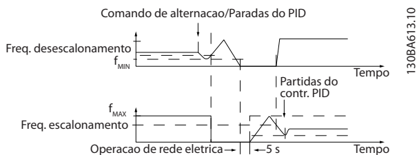
Ilustração 3.93 Configuração Lento
