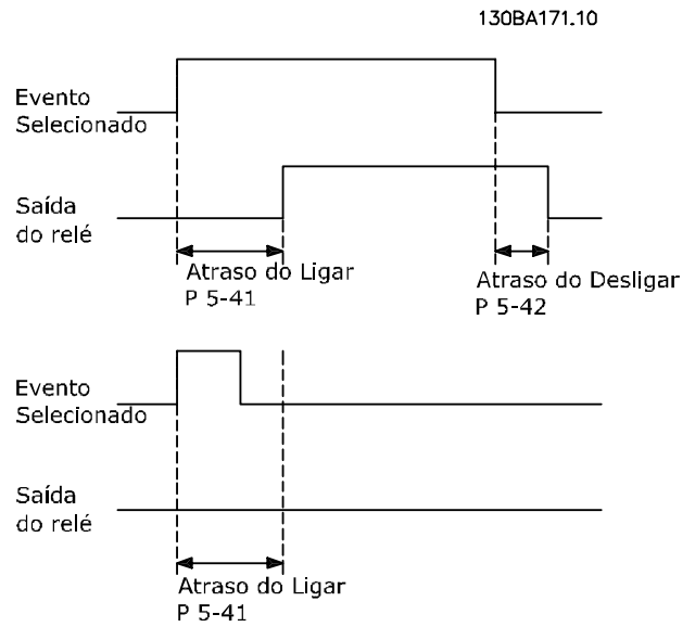
Ilustração 3.29 Atraso de ativação do relé
