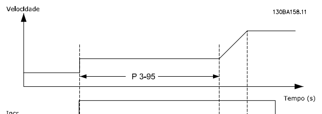
Ilustração 3.25 Atraso de Rampa Caso 1
