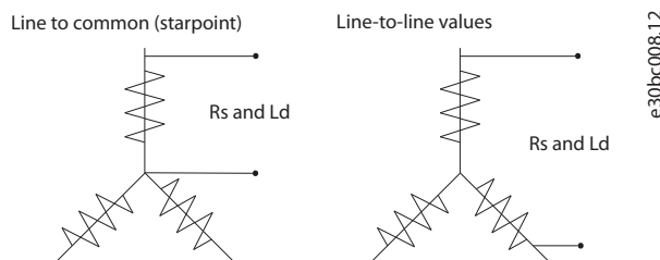
Ilustração 3.6 Setups do enrolamento do estator
