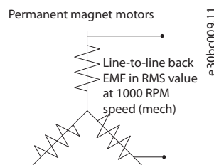
Ilustração 3.7 Definições dos parâmetros da máquina para a Força Contra Eletromotriz de Motores PM
