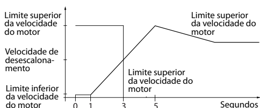
Ilustração 3.91 Limite Desescal.
