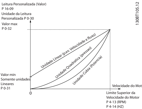
Ilustração 3.3 Leit.Personalz.
