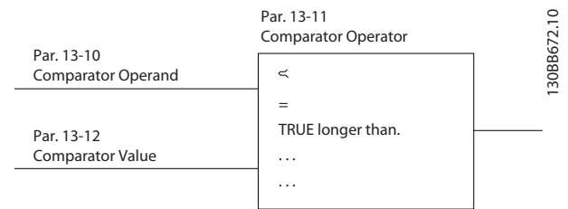
Ilustração 3.41 Comparadores
