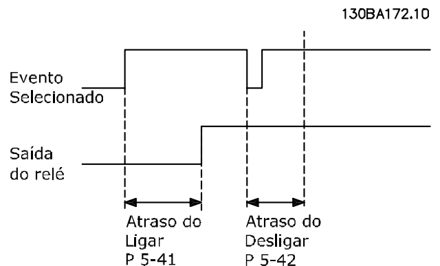
Ilustração 3.30 Atraso de desativação do relé
