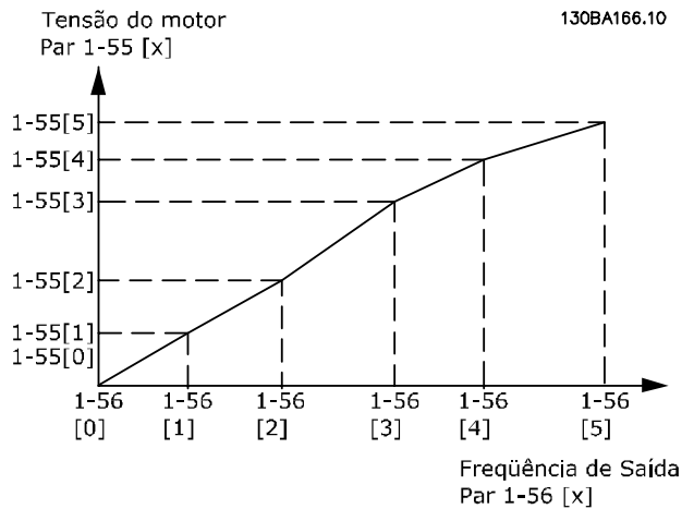
Ilustração 3.9 Característica U/f
