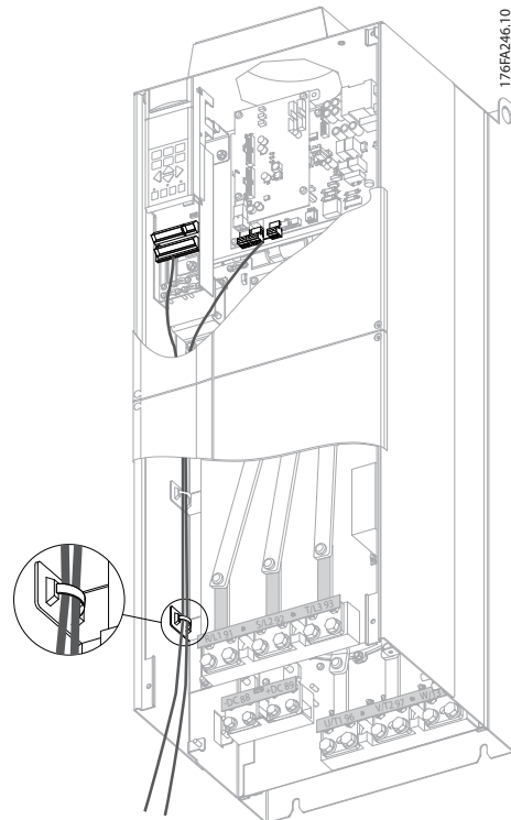
Εικόνα 3.68 Διαδρομή καλωδίωσης κάρτας ελέγχου για E1 και E2
