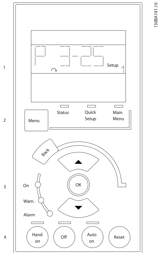
Εικόνα 4.13 Αριθμητικό LCP (NLCP)
