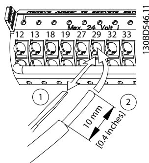
Illustration 4.26 Tilslutning af styreledninger
