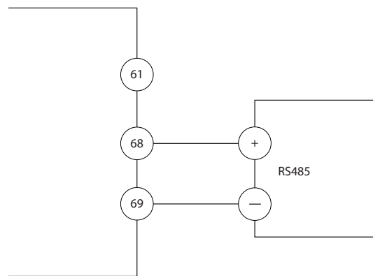
Illustration 4.28 Forbindelsesdiagram for seriel kommunikation
