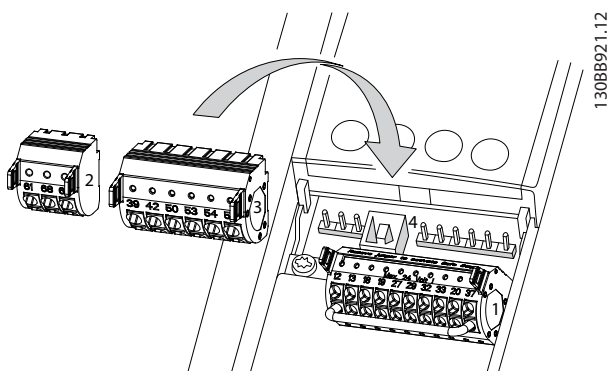
Illustration 4.24 Styreklemmeplaceringer
