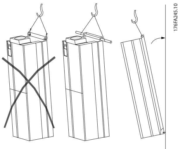
Illustration 3.2 Anbefalet løftemetode
