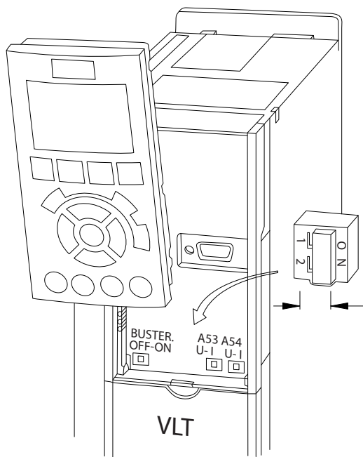
Illustration 4.27 Placering af kontakter til klemme 53 og 54
