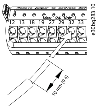
Illustrasjon 5.37 Tilkopling av solide styreledninger
