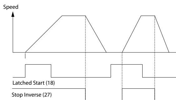
图 8.2 自锁启动/停止反逻辑
