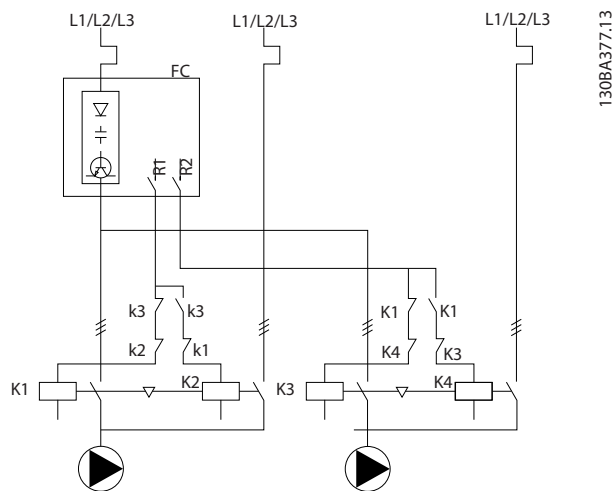
图 8.8 变频泵轮换接线图。
