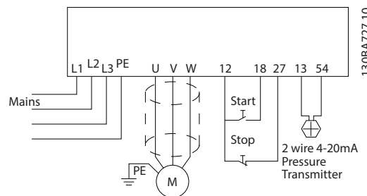
图 8.4 潜水泵应用接线
