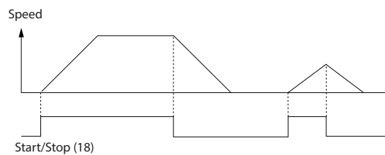
图 8.1 带 Safe Torque Off 的启动/停止
