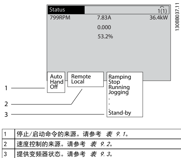
图 9.2 状态显示
