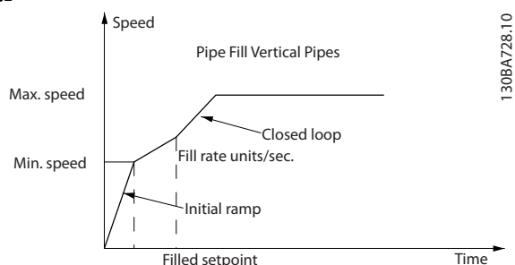
图 8.5 管道填充模式的性能曲线
