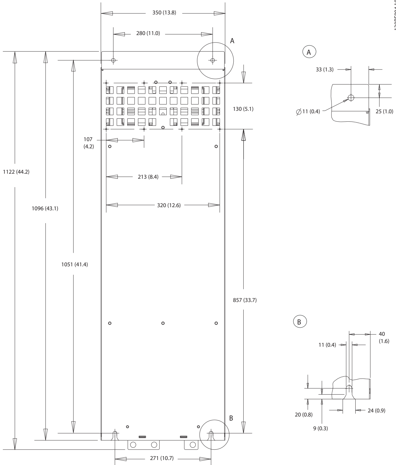
图 10.17 D4h 后视图
