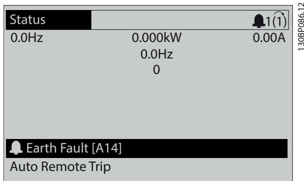
图 9.3 报警示例
