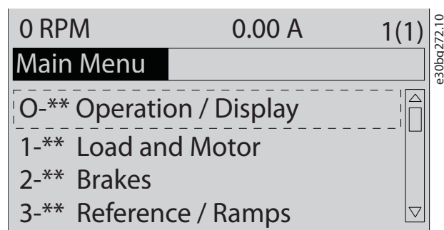
图 3.7 主菜单视图
