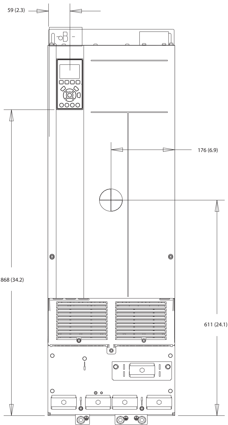
图 10.15 D4h 的正视图
