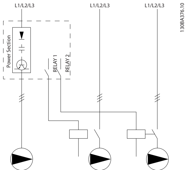
图 8.7 恒速泵/变速泵接线图
