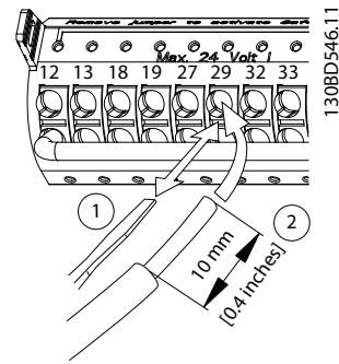
Ilustración 5.20 Conexión de los cables de control
