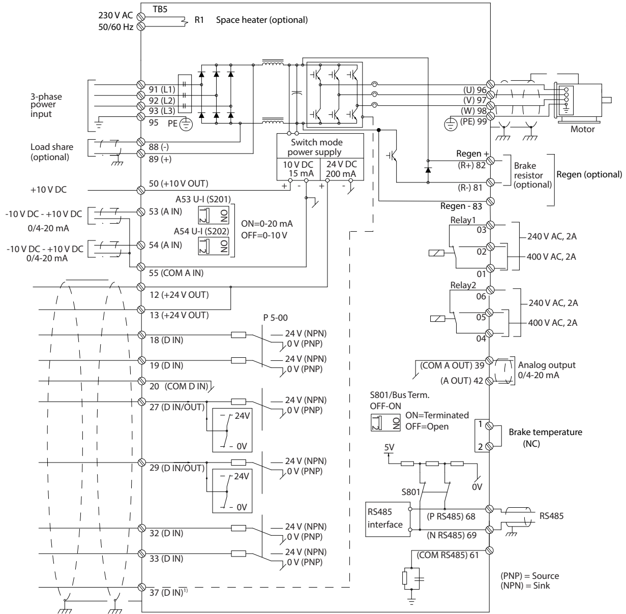
Çizim 5.2 Temel Kablo Tesisatı Şeması
