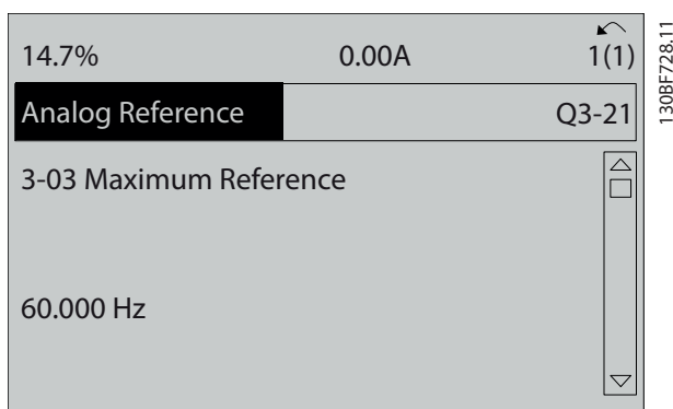
Illustration 6.7 Parameter 3-03 Maksimumreference
