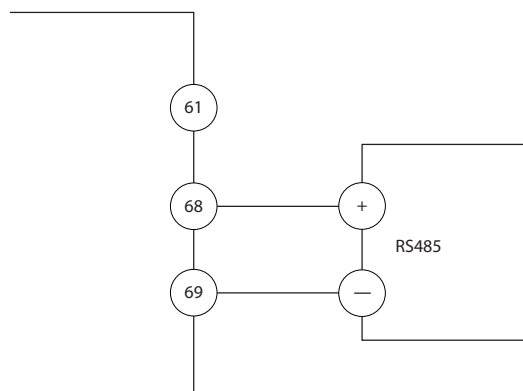
Illustration 5.22 Forbindelsesdiagram for seriel kommunikation
