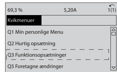
Illustration 6.3 Q3 Funktionsopsæt.
