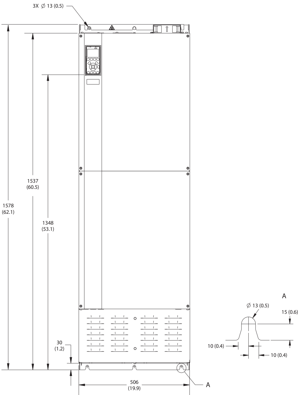
Abbildung 9.10 Frontansicht E3h
