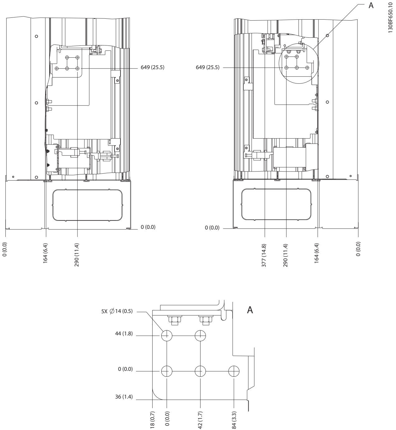
Abbildung 5.7 E1h-Klemmenabmessungen (Seitenansichten)
