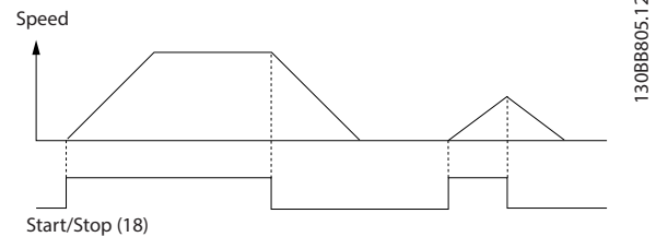
Abbildung 7.2 Start-/Stopp-Befehl mit Safe Torque Off
