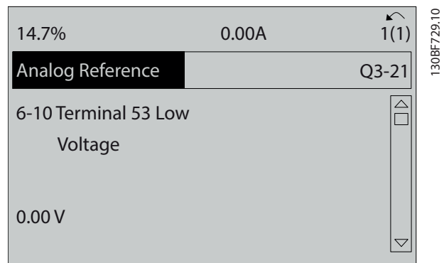
Abbildung 6.8 Parameter 6-10 Klemme 53 Skal. Min.Spannung
