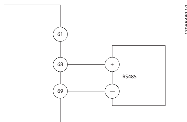
Illustration 5.22 Schéma de câblage de la communication série
