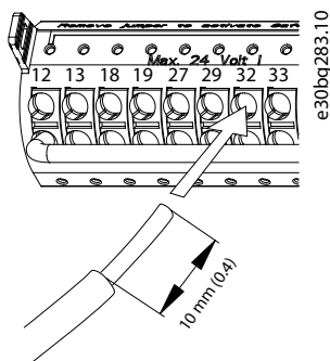
Illustration 5.20 Raccordement de fils de commande solides
