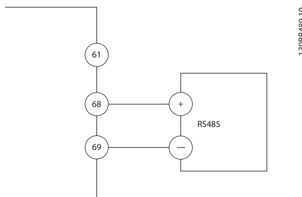
Ilustración 5.22 Diagrama de cableado de comunicación serie
