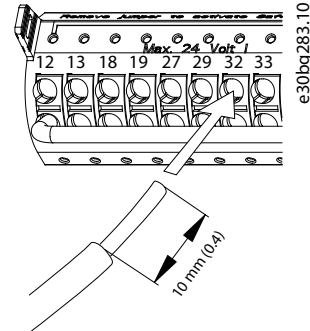
Bild 5.20 Ansluta fasta styrkablar
