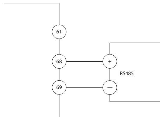
Afbeelding 5.22 Bedradingsschema voor seriële communicatie
