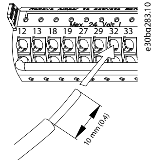
Afbeelding 5.20 Stuurdraden met massieve kern aansluiten
