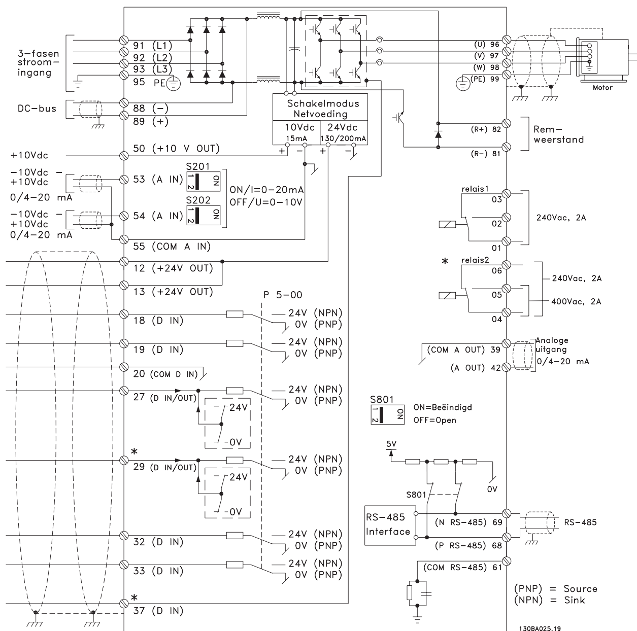
Afbeelding 5.2 Eenvoudig bedradingsschema
