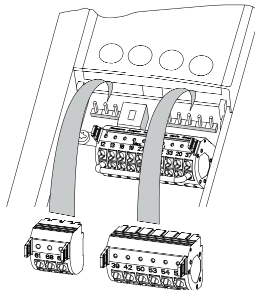
Afbeelding 5.17 Stuurklemposities
