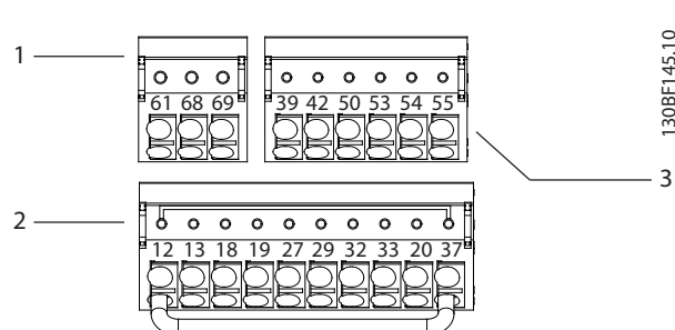
Afbeelding 5.17 Stuurklemposities
