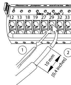
Ilustração 5.21 Conexão de fios de controle flexíveis
