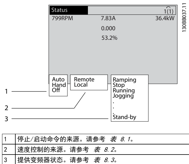
图 8.2 状态显示
