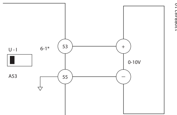
Slika 6.12 Primer ožičenja za eksterni uređaj koji daje upravljački signal od 0–10 V
