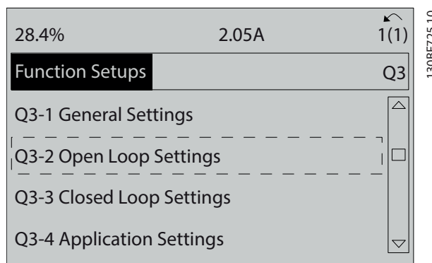
Ilustrația 6.4 Q3-2 Config bucl desch
