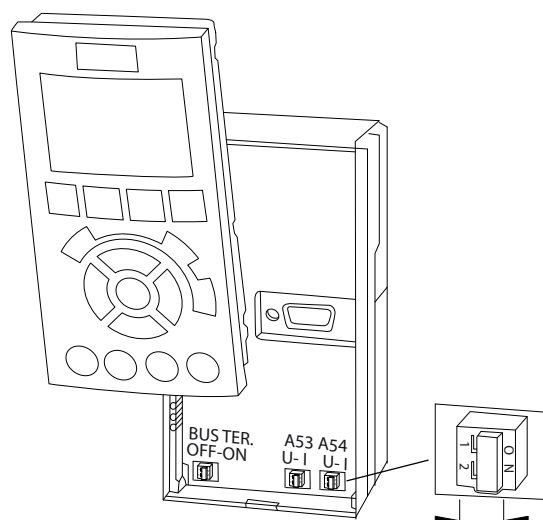
Ilustrația 5.23 Locația comutatoarelor bornelor 53 și 54
