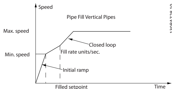
图 12.5 管道填充模式的性能曲线
