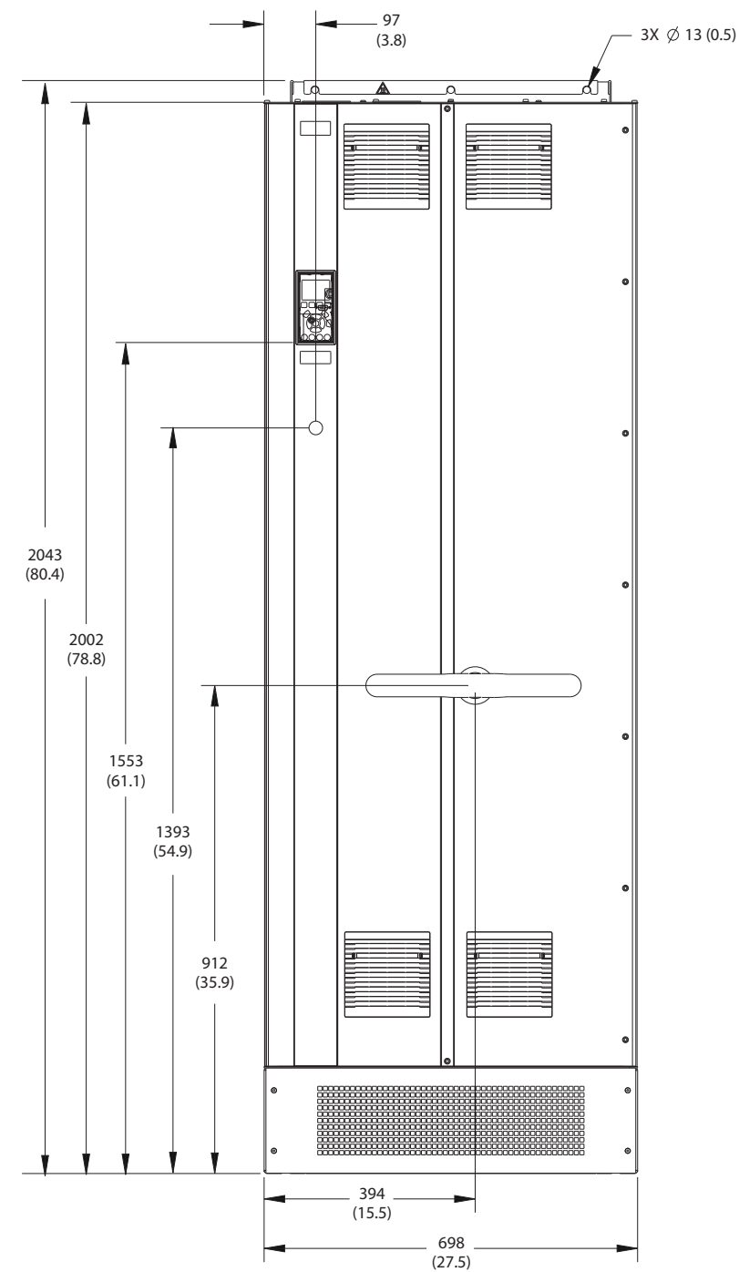
图 8.7 E2h 的正视图
