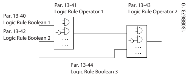
图 5.6 逻辑规则
