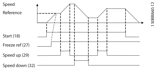
图 12.3 加速/减速
