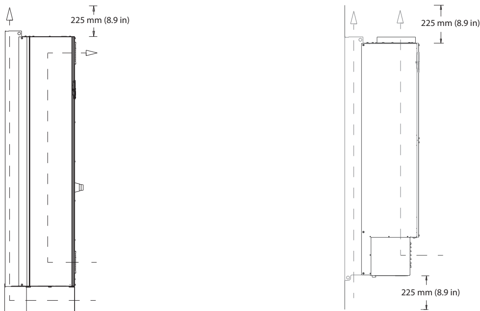
图 5.17 E1h/E2h (左) 和 E3h/E4h (右) 的标准气流配置
