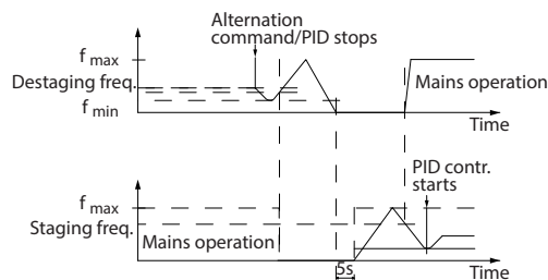
图 5.11 变频泵轮换
