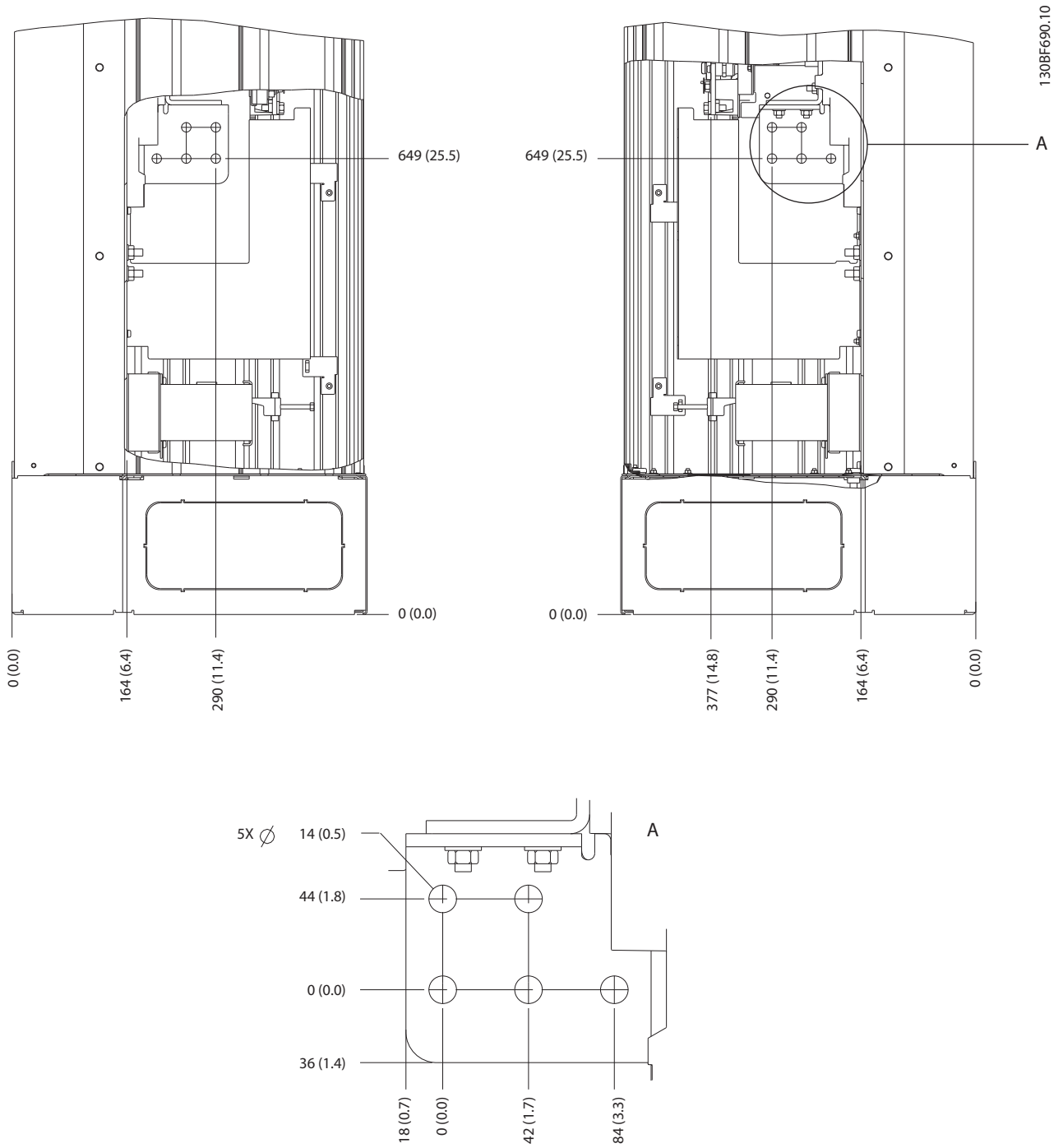
图 8.12 E2h 端子尺寸 (侧视图)
