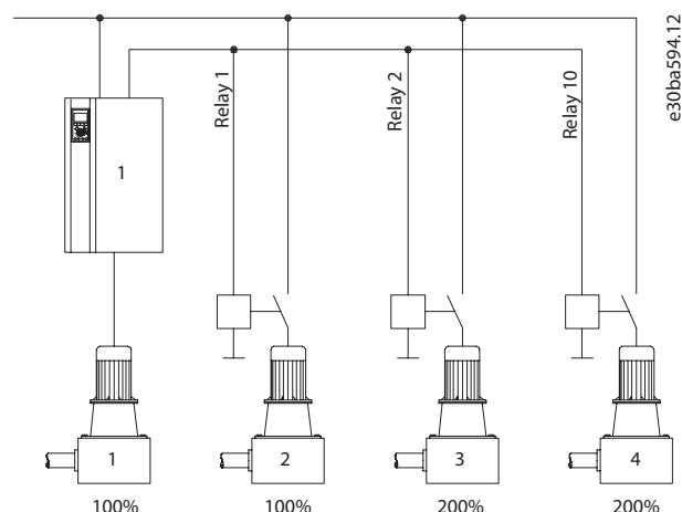
图 5.8 应用概述
