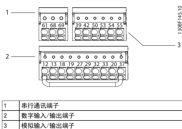
图 10.6 连接器上的端子号
