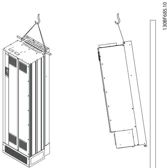
图 9.1 建议的起吊方法
