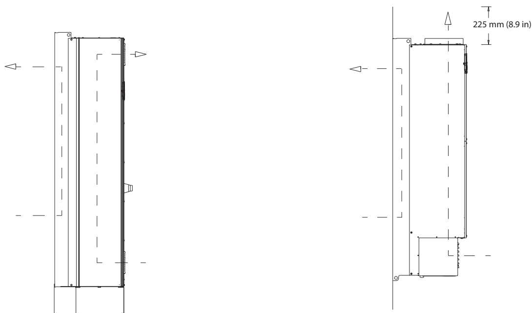
图 5.18 E1h/E2h (左) 和 E3h/E4h (右) 上通过后壁的可选气流配置
